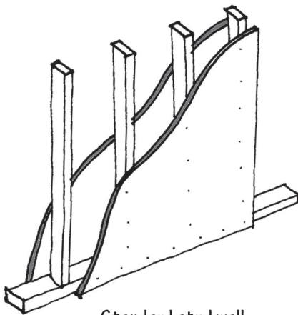
Standard stud wall
