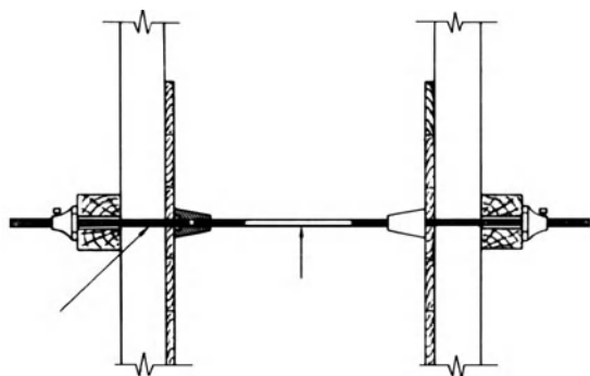
tie rod
