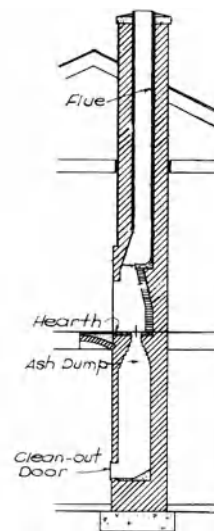
chimney
