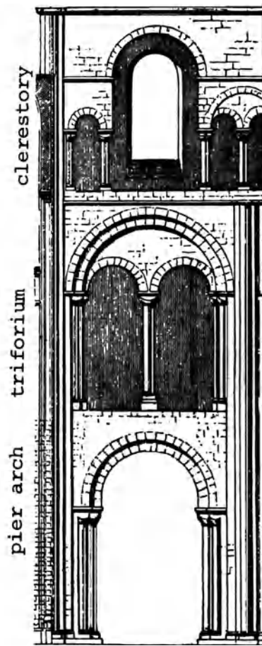
triforium
