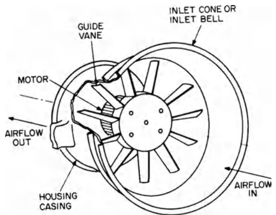
axial-flow fan
