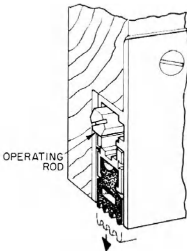
automatic door bottom
