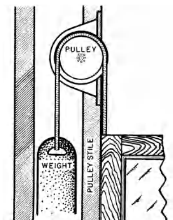
pulley stile
