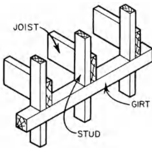
girt, 2
