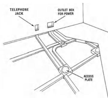
underfloor conduit system
