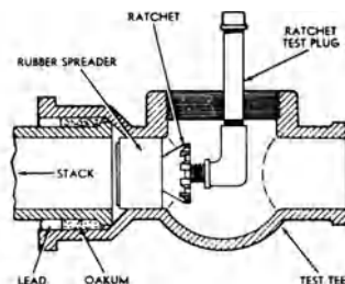
test tee
