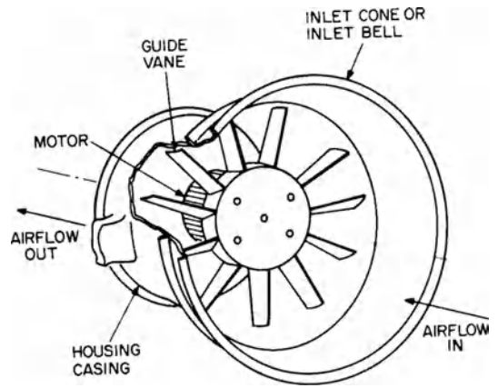
axial-flow fan
