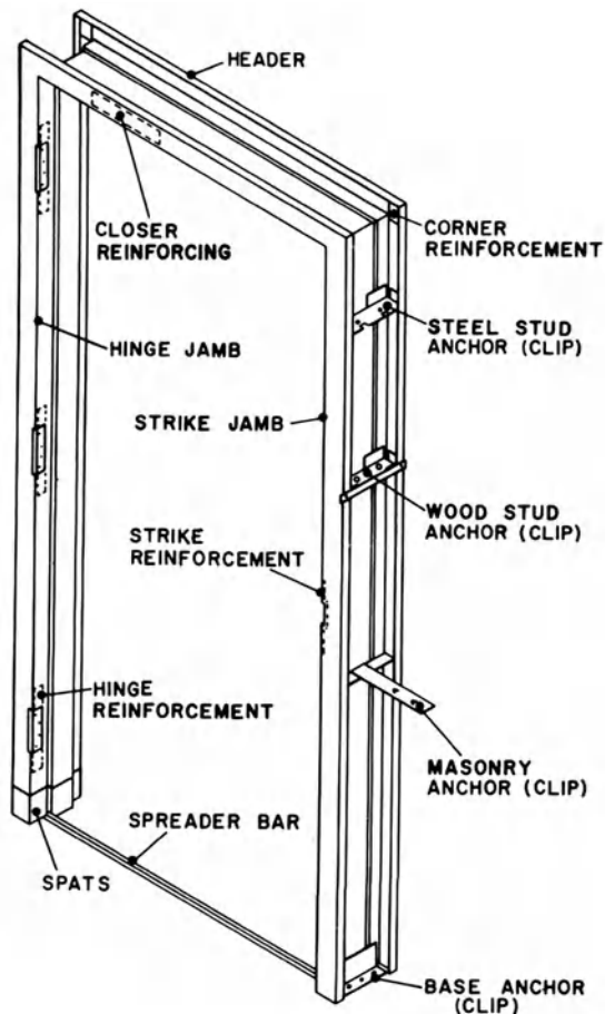
doorframe
