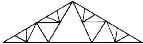
fan Fink truss
