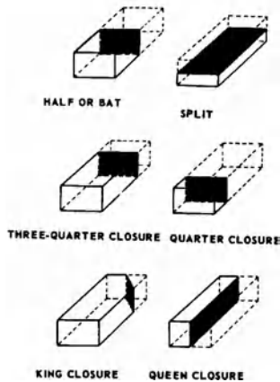
brick: nomenclature
