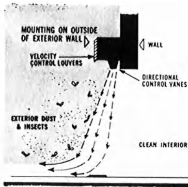
air curtain or air door
