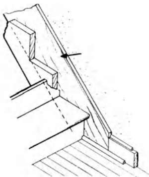
face string
