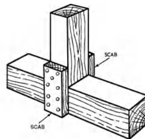
scab
