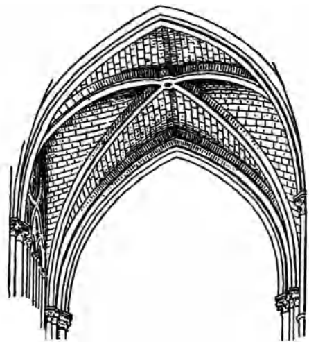
quadripartite vault
