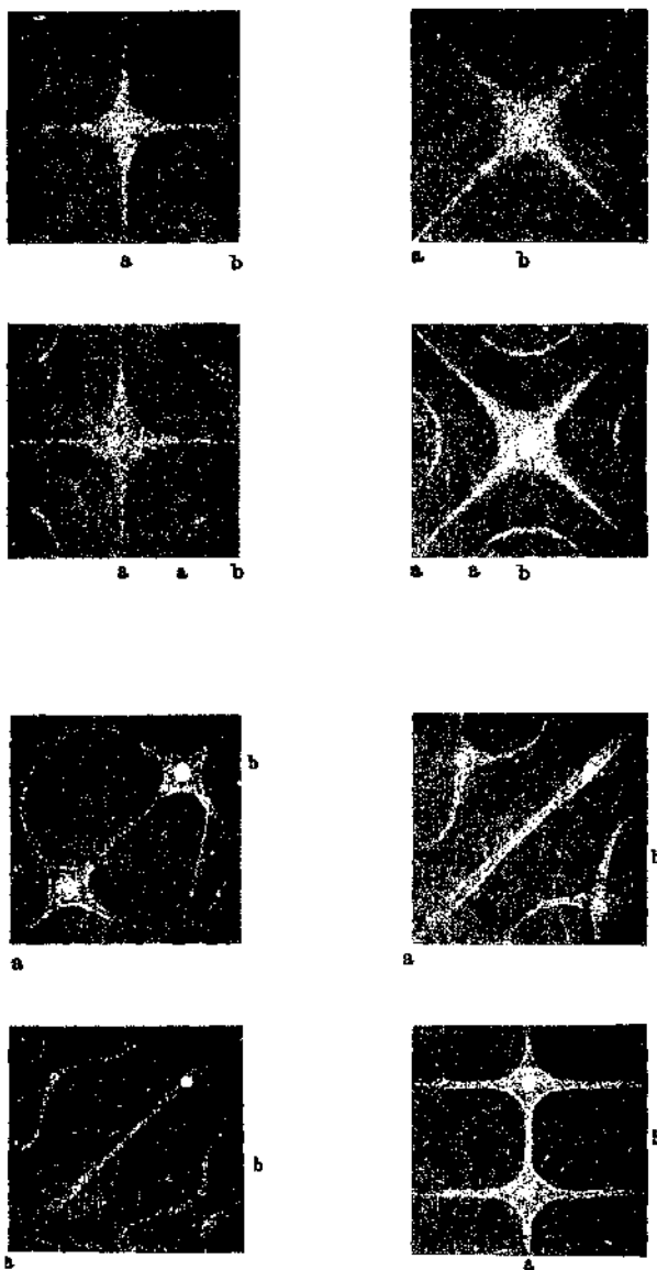
Fig. 27. CHLADNI FIGURES.*
