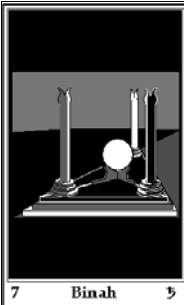
7 Binah ♁
