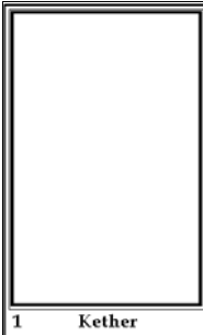
1 Kether
