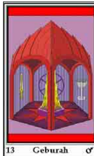
13 Geburah ♂
