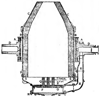
FIG. 16.—12-15 ton Bessemer Converter.
