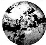
FIG. 4.—GRANITE RUBISLAW, ABERDEEN ( \times 10 ).
