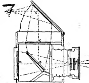
Fig. 10.—Reflex Camera.
