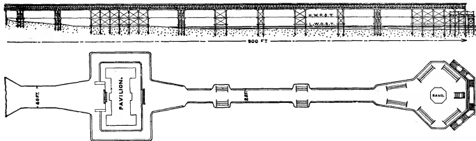
Fig. 3.—Promenade Pier.
