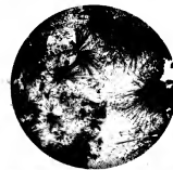
FIG. 7.—LUXULLIANITE, LUXULYAN, CORNWALL ( \times 15 ).
