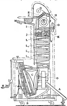
FIG. 36.—Modern Pianola.
