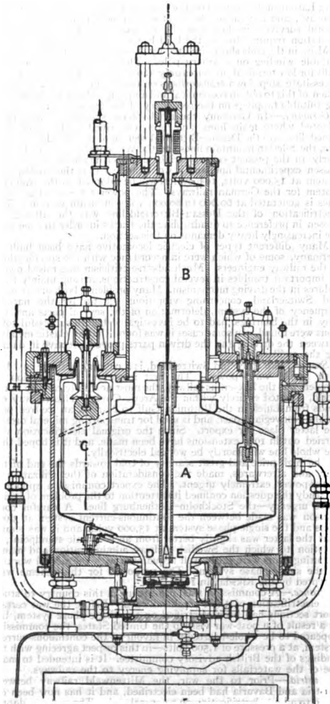
FIG. 2.—300-Ampere Mercury-Vapour Rectifier.
