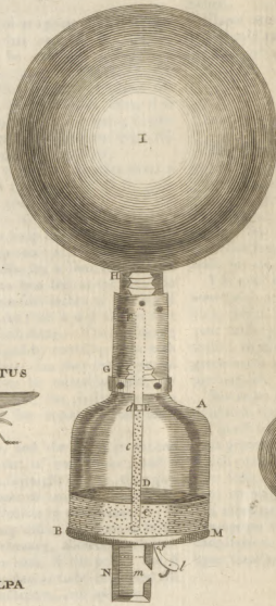
Fig. 1. SEA GAGE
