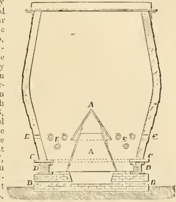
FIG. 1.—Gjers's Kiln.
