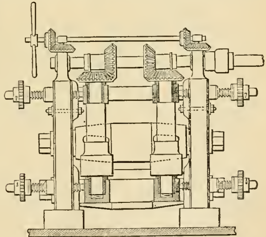
FIG. 48.—Universal Rolls.
