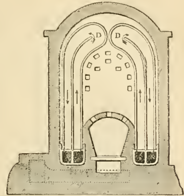
FIG. 18. Pistol Pipe Stove.
