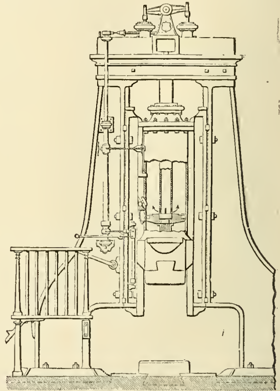
FIG. 45.—Condie's Hammer.
