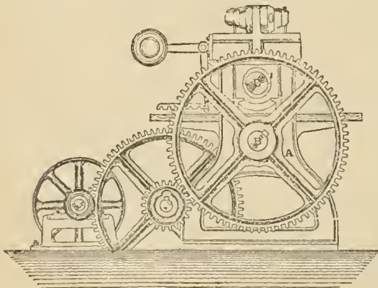
Fig. 10.—Plate Calender.
