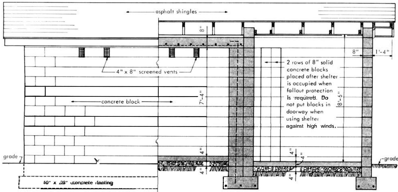
ELEVATION
