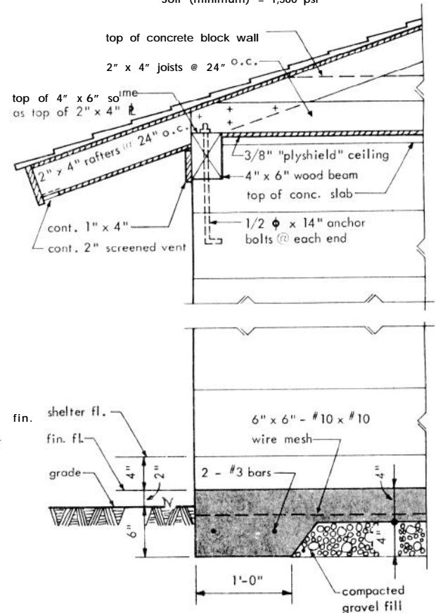
SECTION D-D
