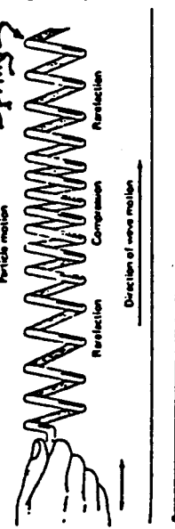
LONGITUDINAL WAVE
