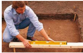
die Wasserwaage level
