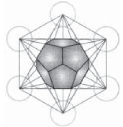
Fig. 6-21a. Solid dodecahedron.
