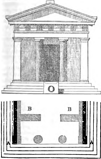
AA, the antæ; BB, the cella or vaos; O, the altar.
