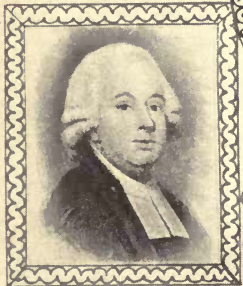
1765 MASKELYNE. 1811
