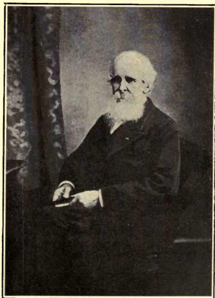
II.—A. GRAHAM.
