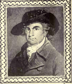
1811 POND. 1855
