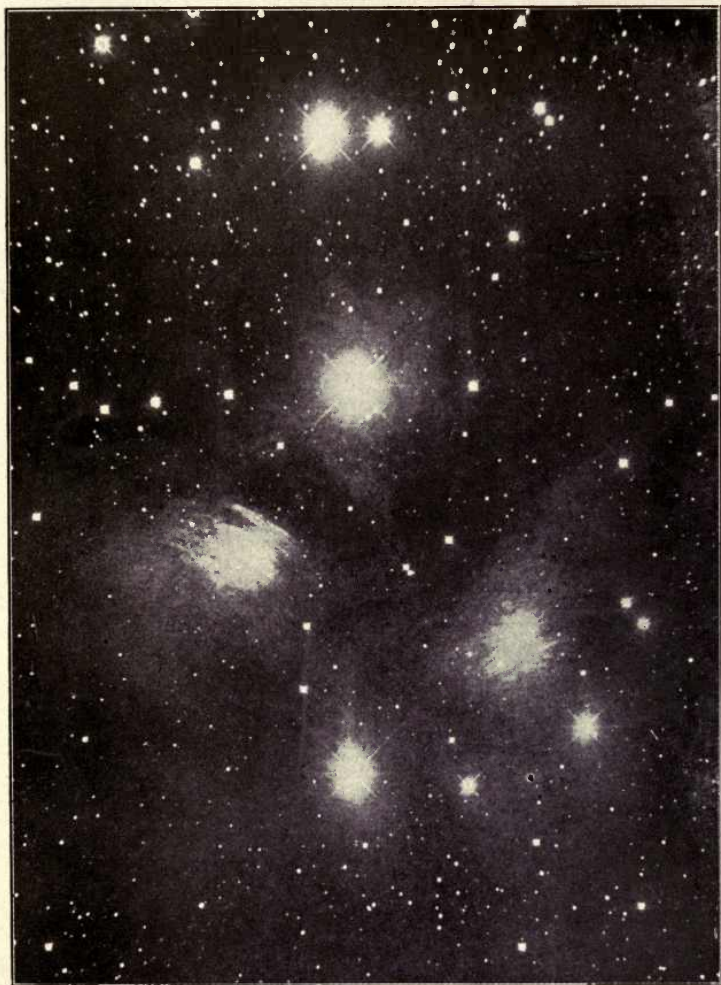
THE PLEIADES
