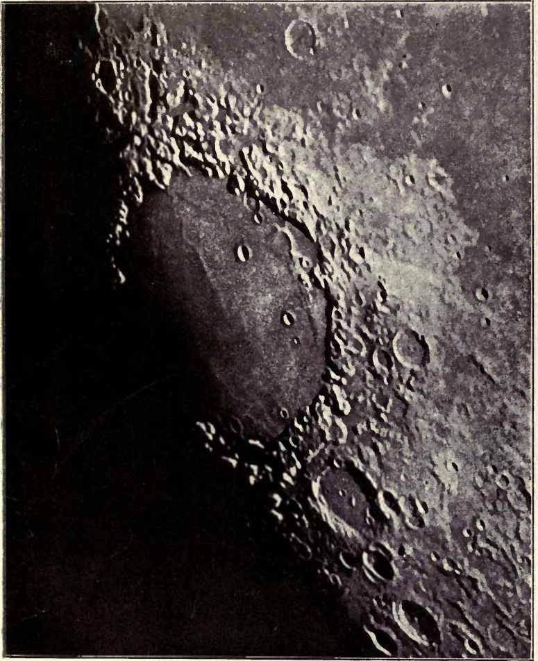
MARE CRISIUM
