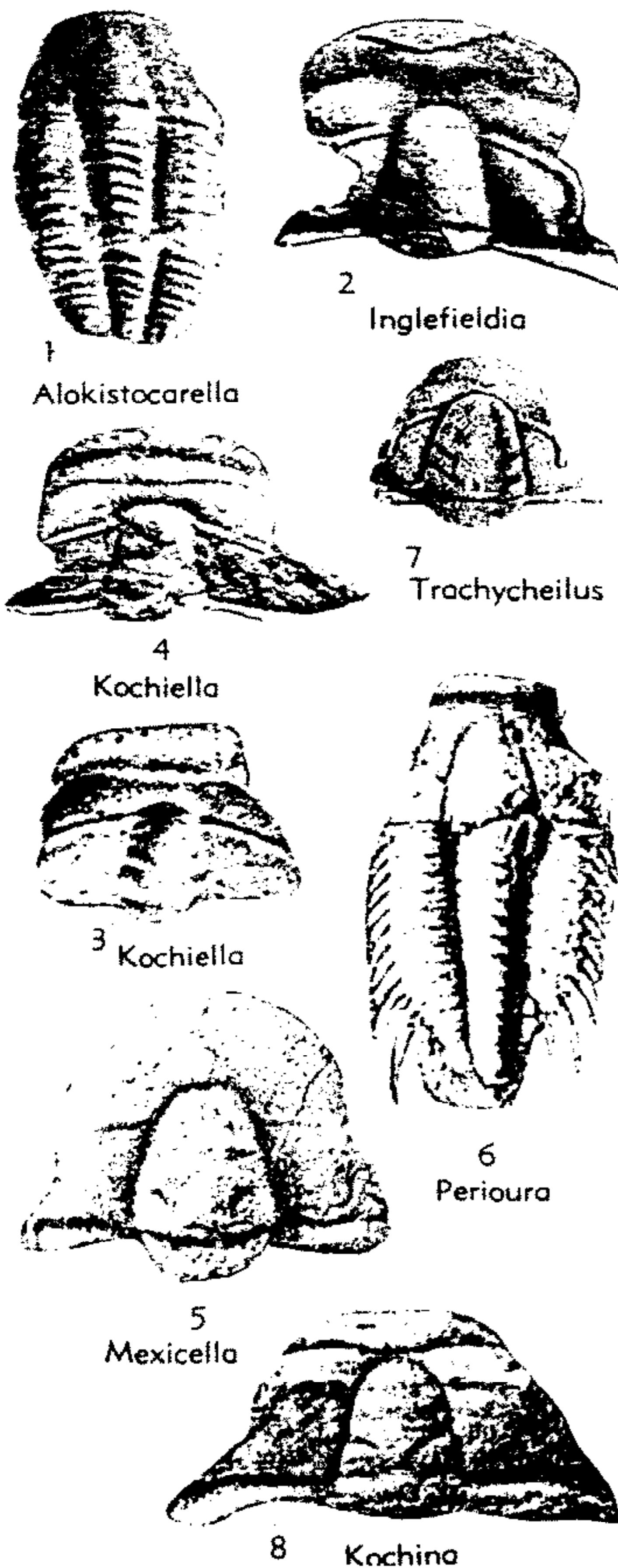
FIG. 178. Alokistocaridae (p. O238-O241).
