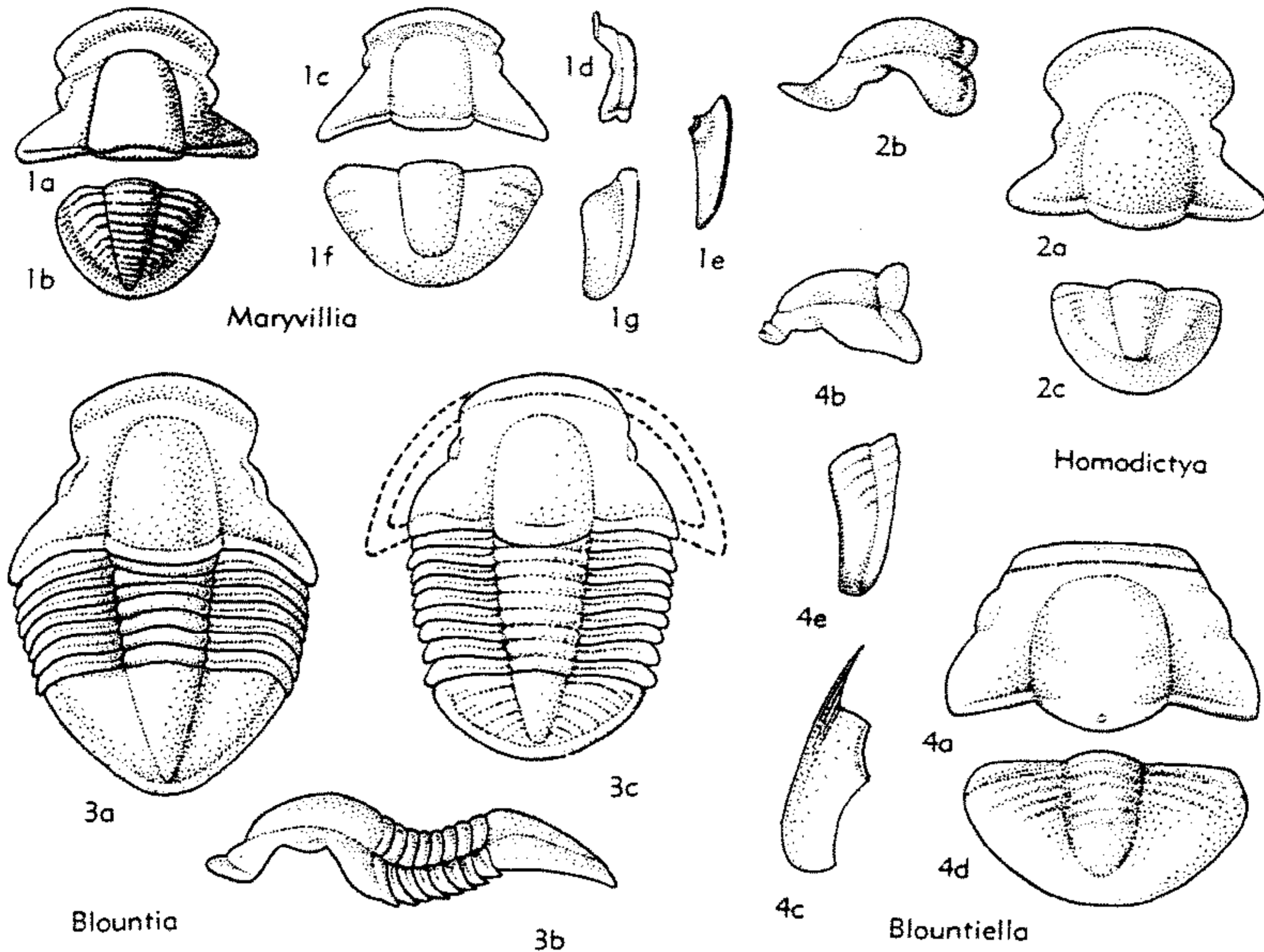
FIG. 216. Asaphiscidae (Blountiinae) (p. 0292).
