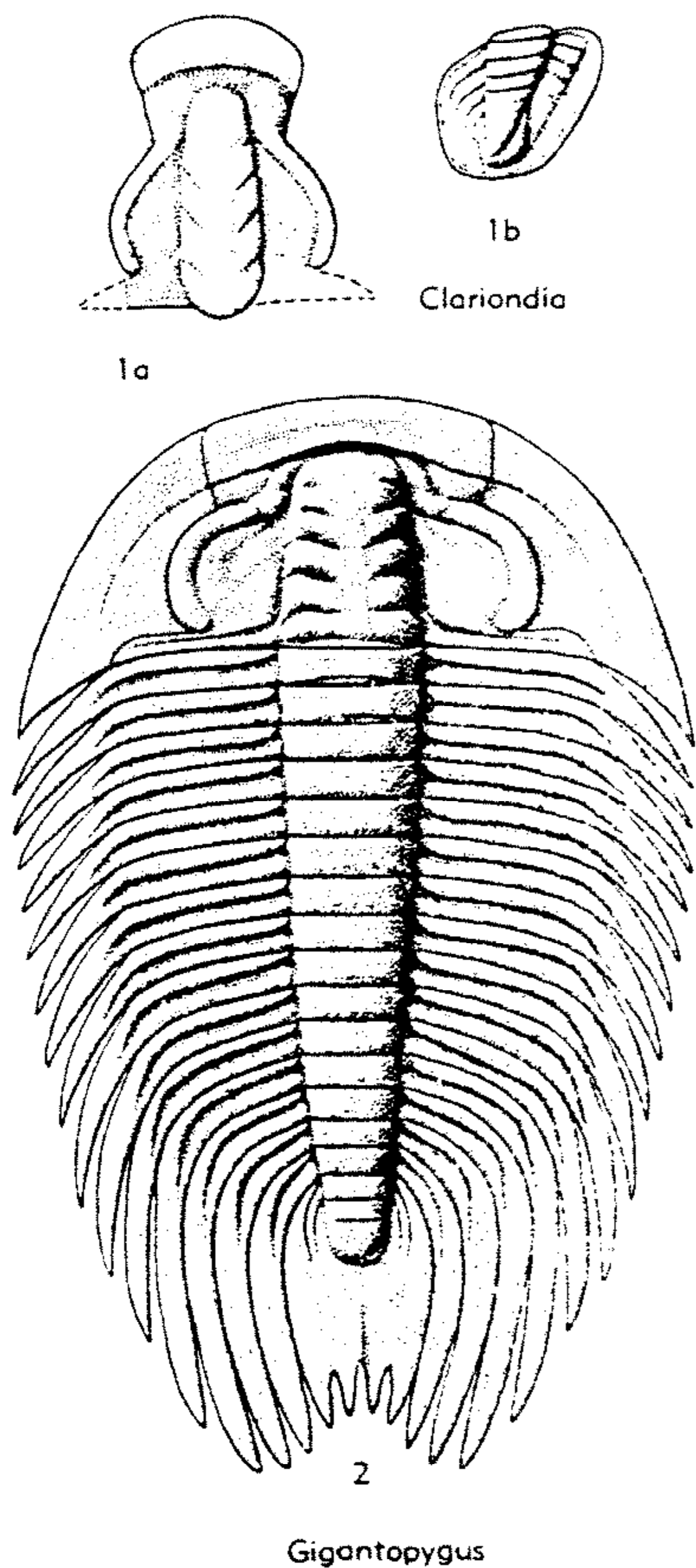
FIG. 146. Neoredlichiidae, Gigantopygidae (p. 0201, 0204).
