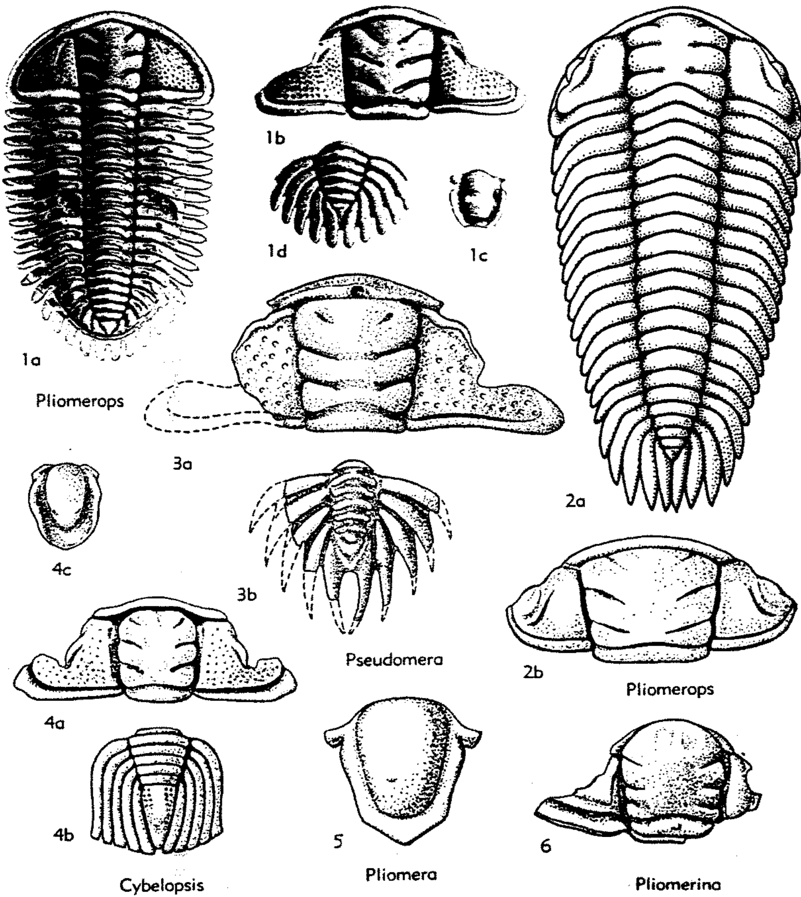
FIG. 345. Pliomeridae (Pliomerinae) (p. O439-O440).
