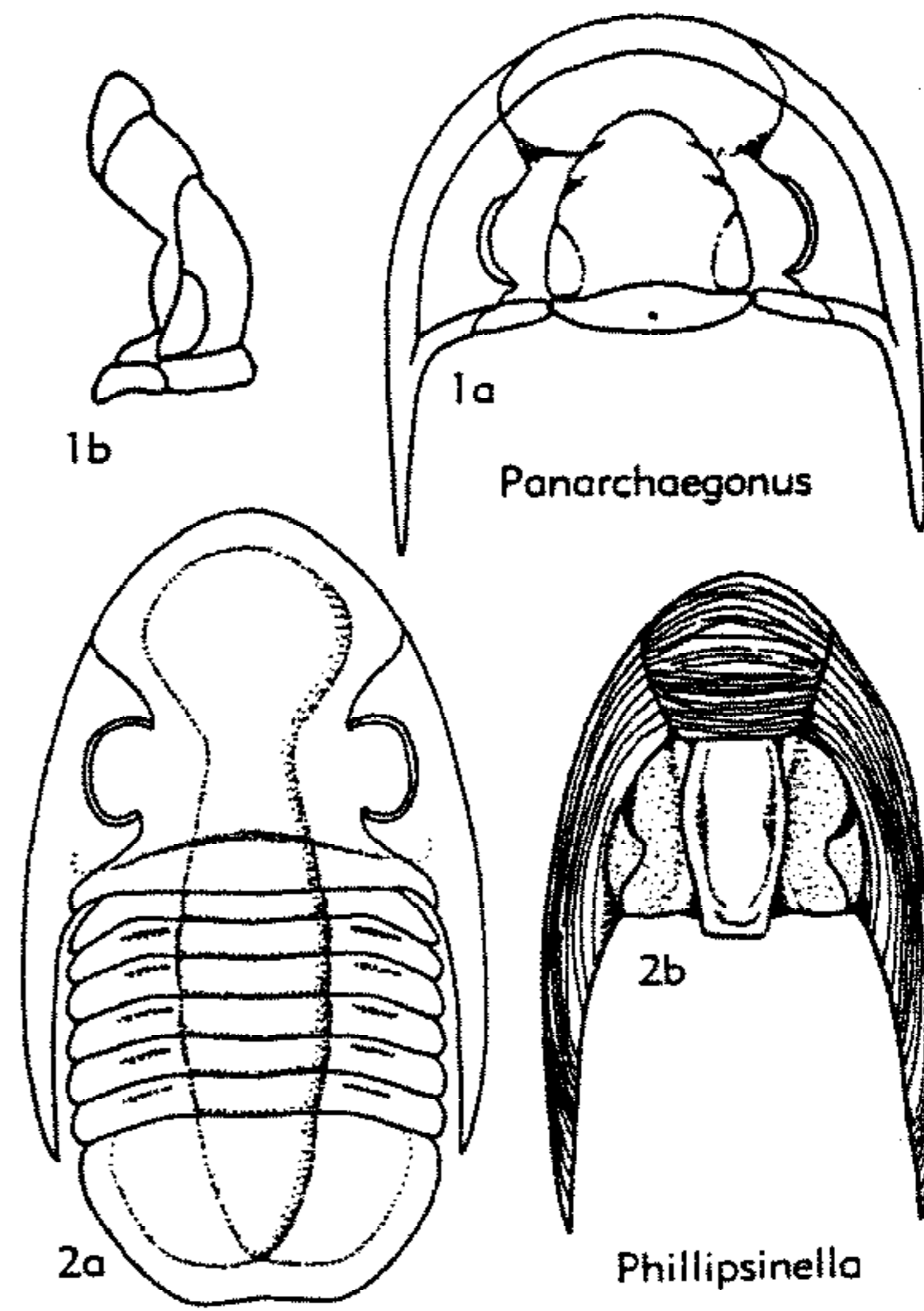
FIG. 311. Brachymetopidae, Phillipsinellidae (p. 0408-0409).
