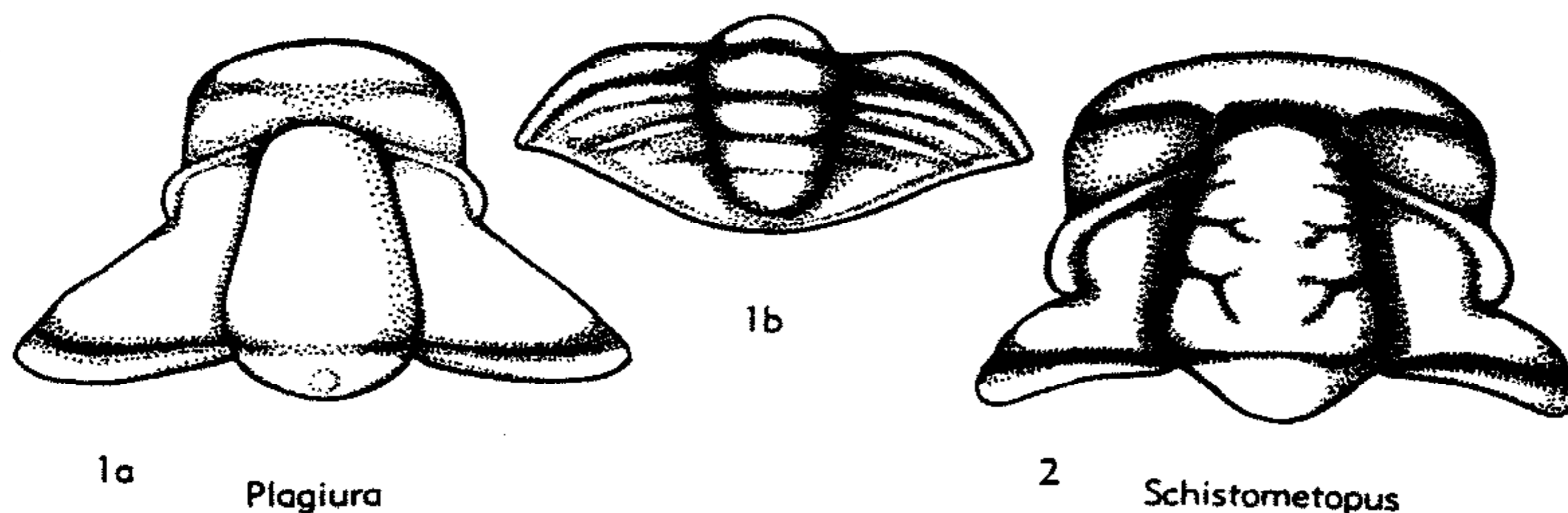
FIG. 409. Incertae sedis. Middle Cambrian genera (p. 0516).
