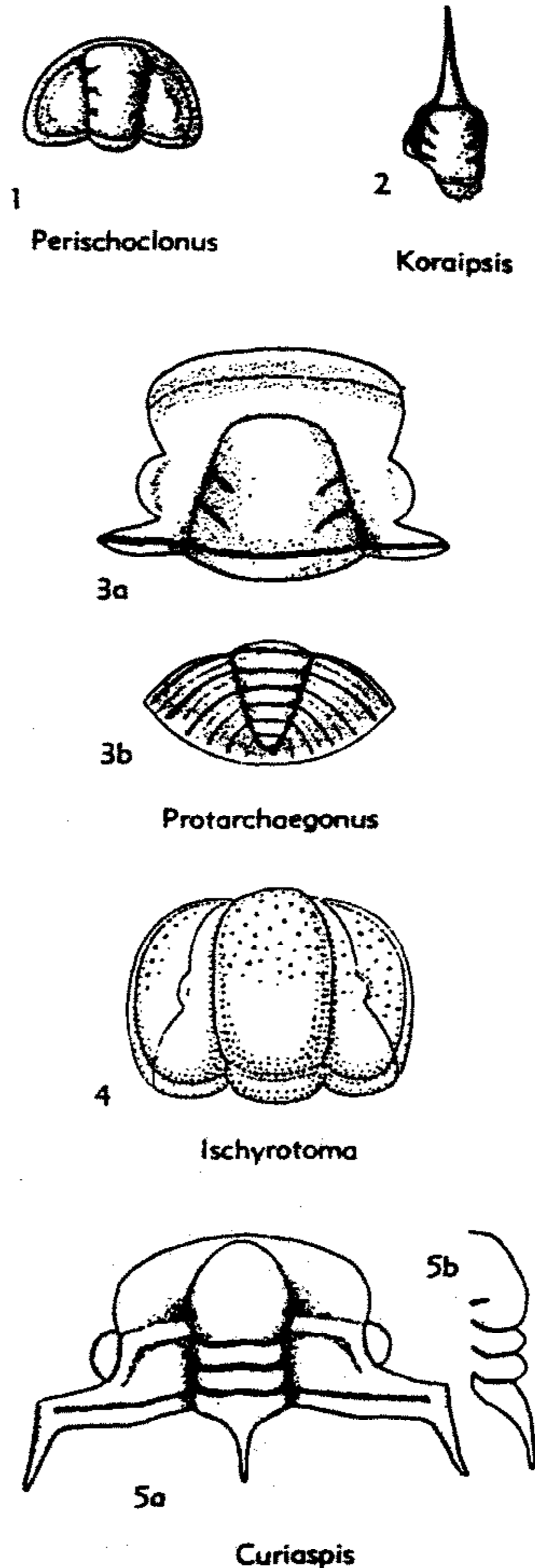
FIG. 413. Incertae sedis. Ordovician genera (p. 0521-0524).
