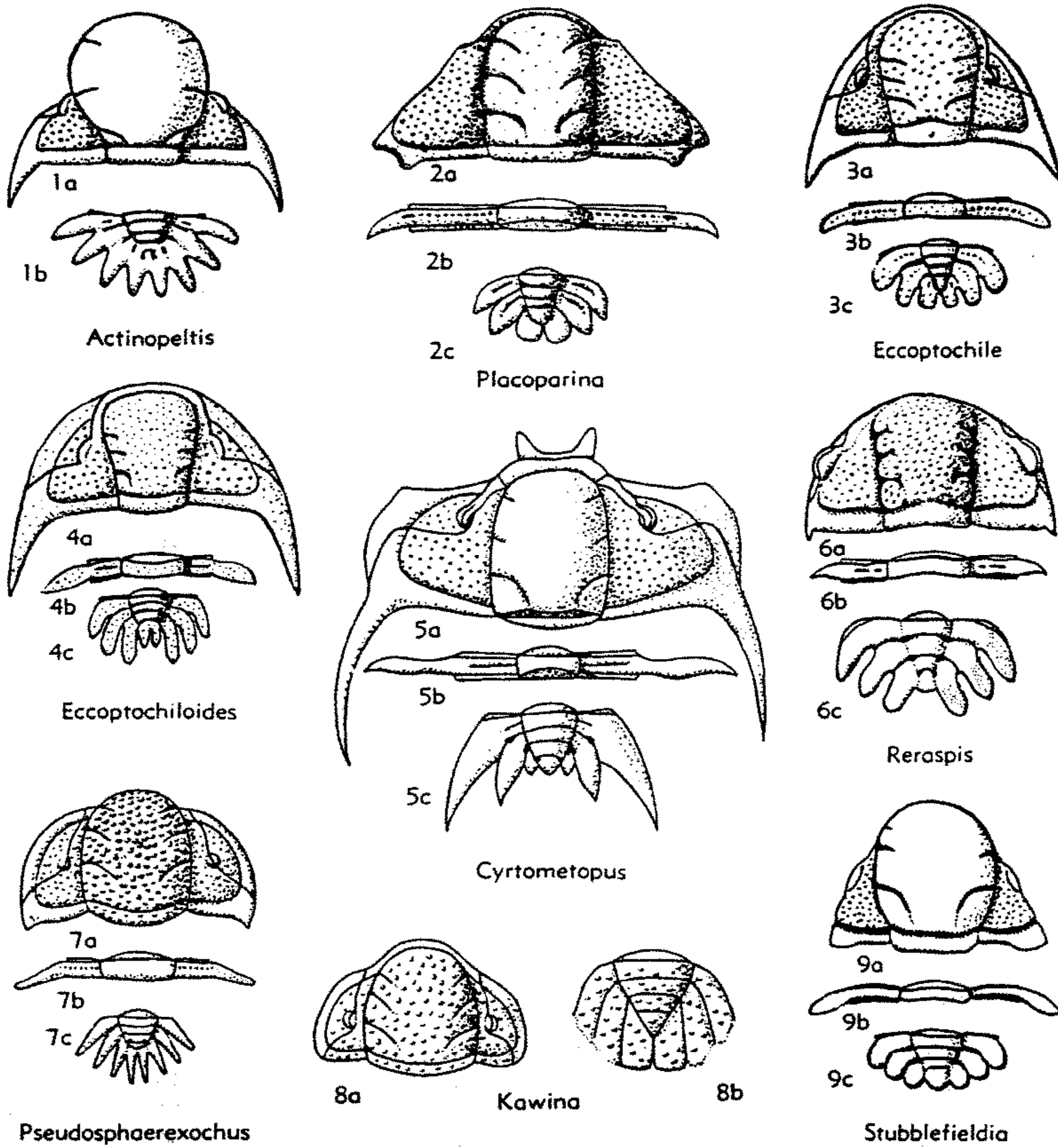
FIG. 337. Cheiruridae (Cyrtometopinae) (p. 0434-0435).
