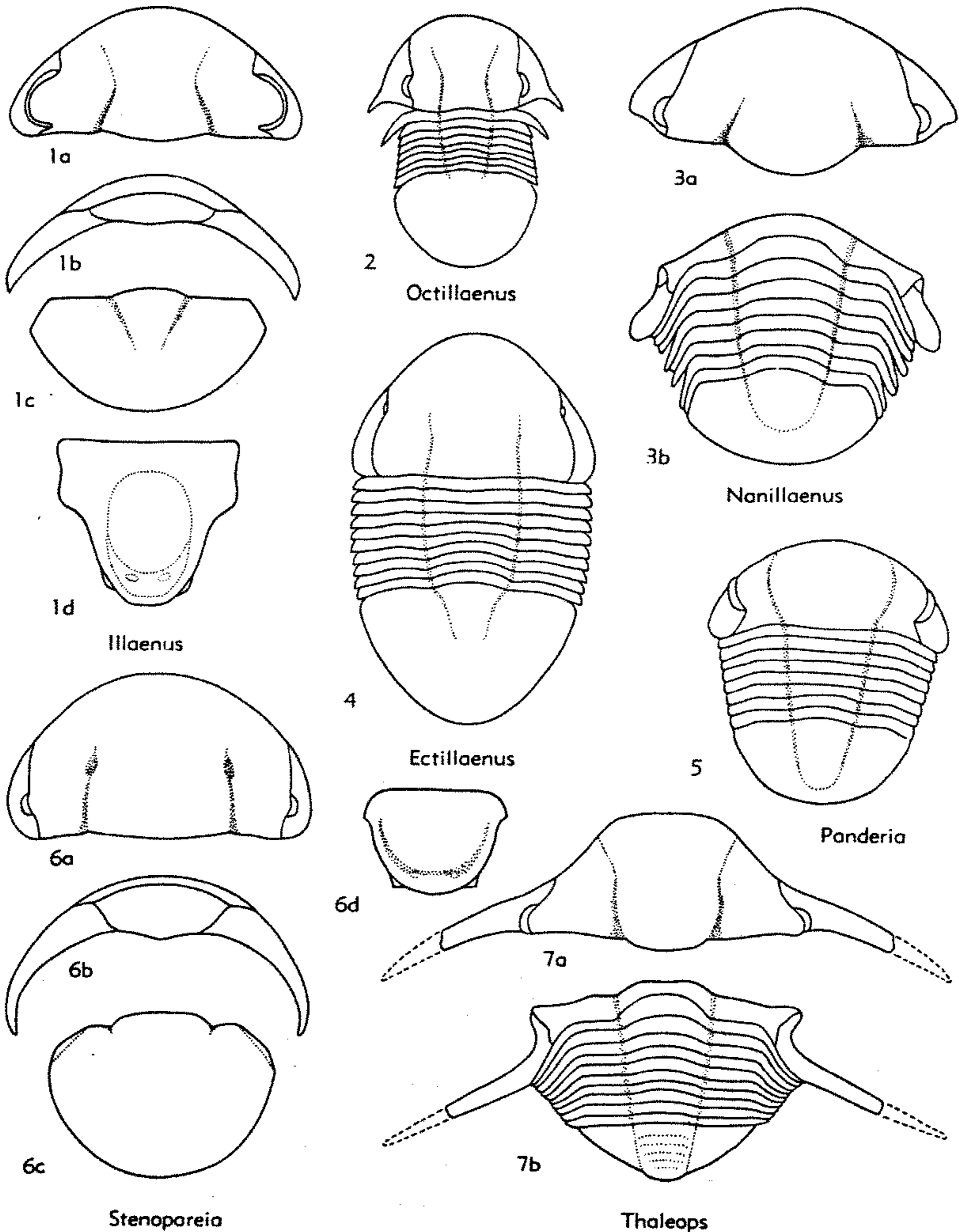
FIG. 282. Illaenidae (Illaeninae) (p. 0372-0374).
