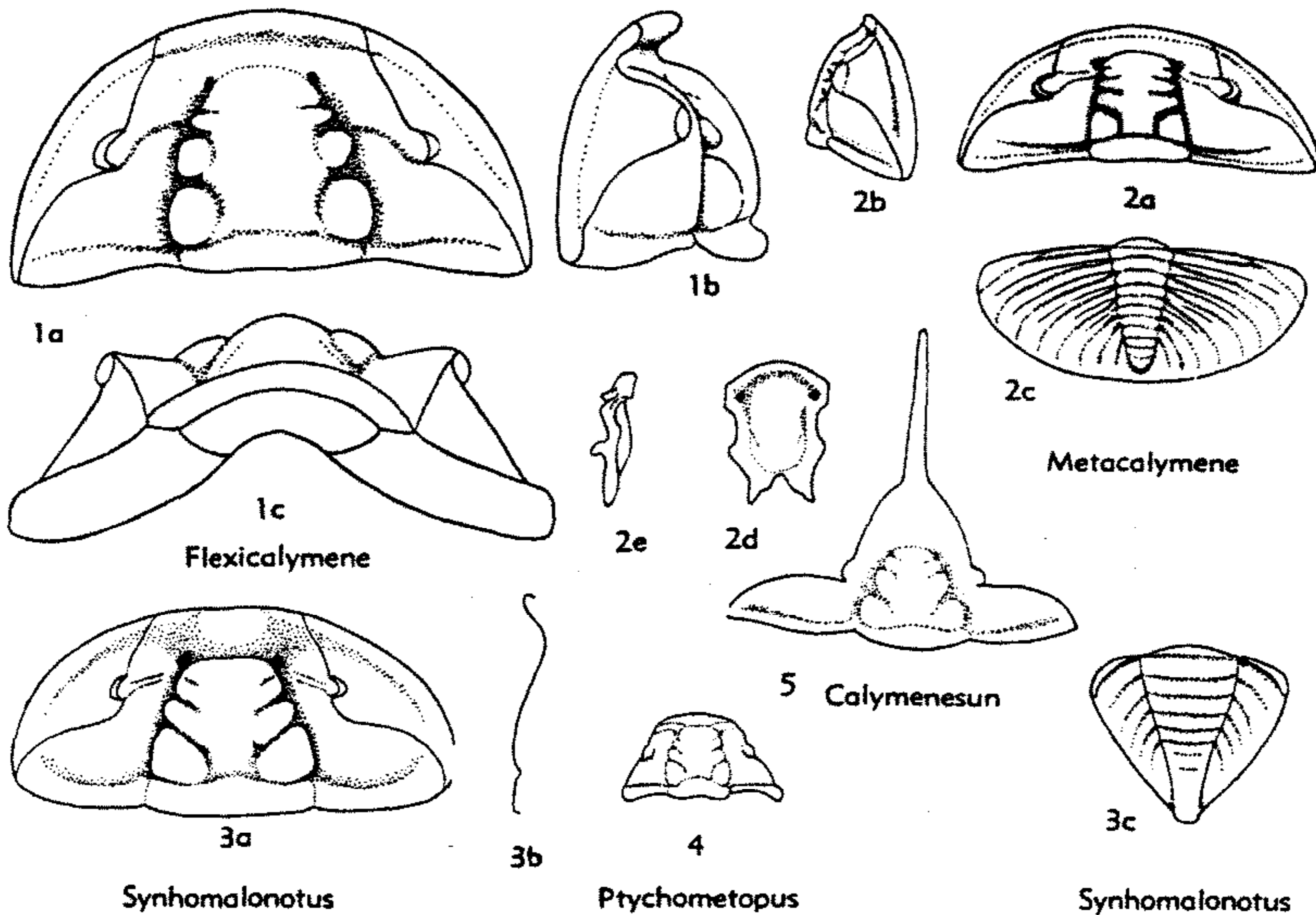
FIG. 354. Calymenidae (Calymeninae) (p. 0452-0453).
