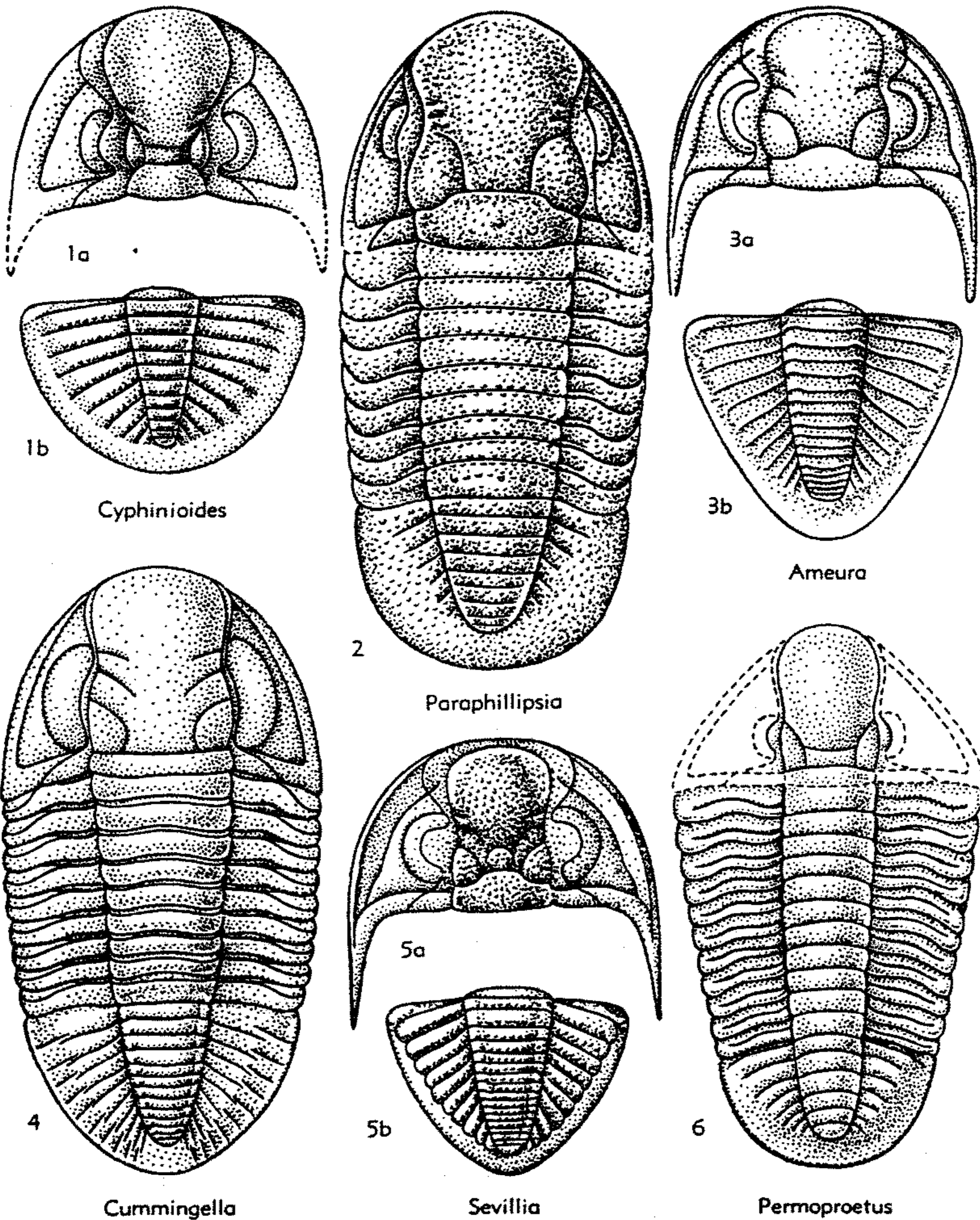
FIG. 308. Phillipsiidae (p. O401).
