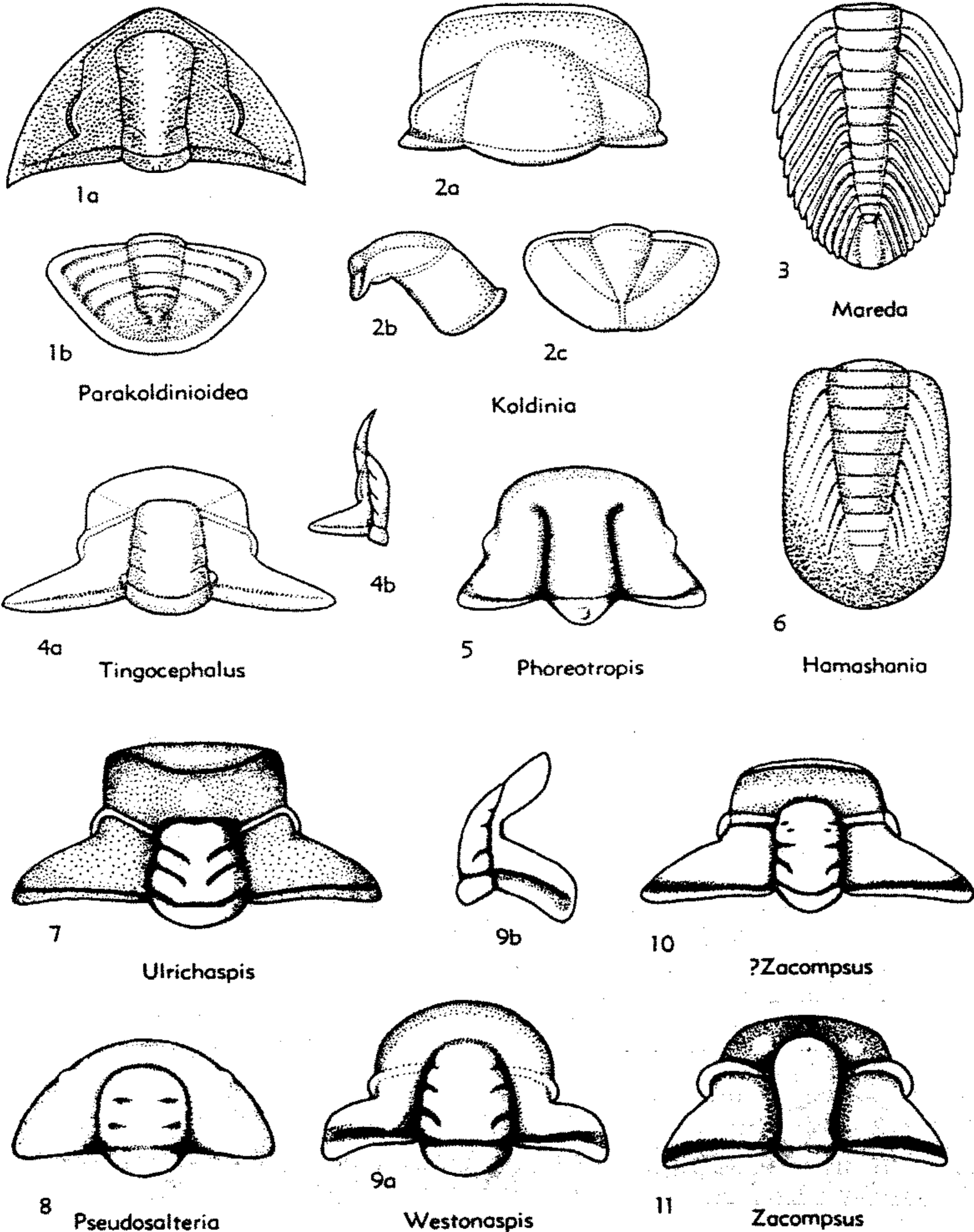
FIG. 411. Incertae sedis. Upper Cambrian genera (p. 0517-0521).
