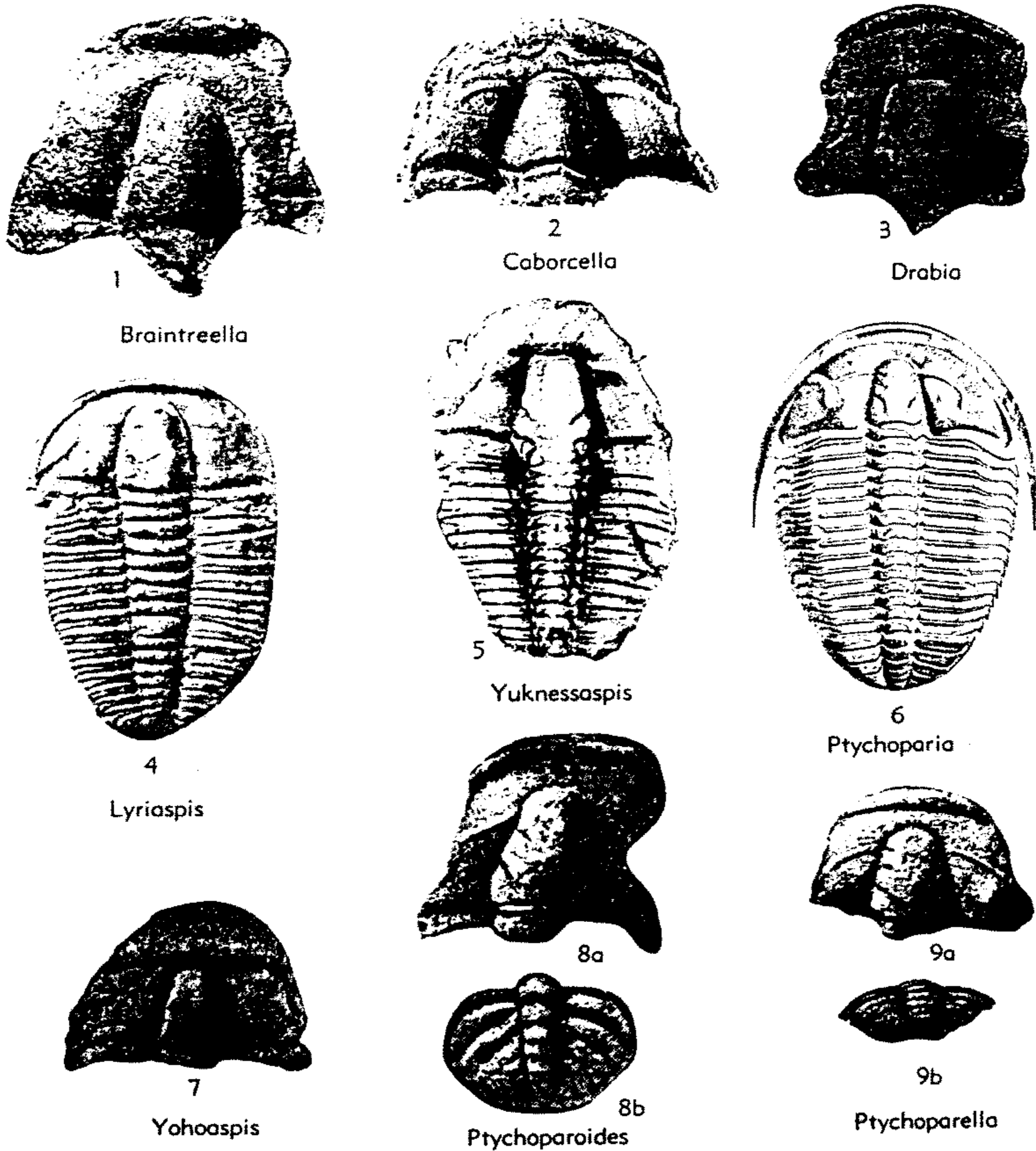
FIG. 170. Ptychopariidae ( Ptychopariinae ) (p. 0233, 0234).
