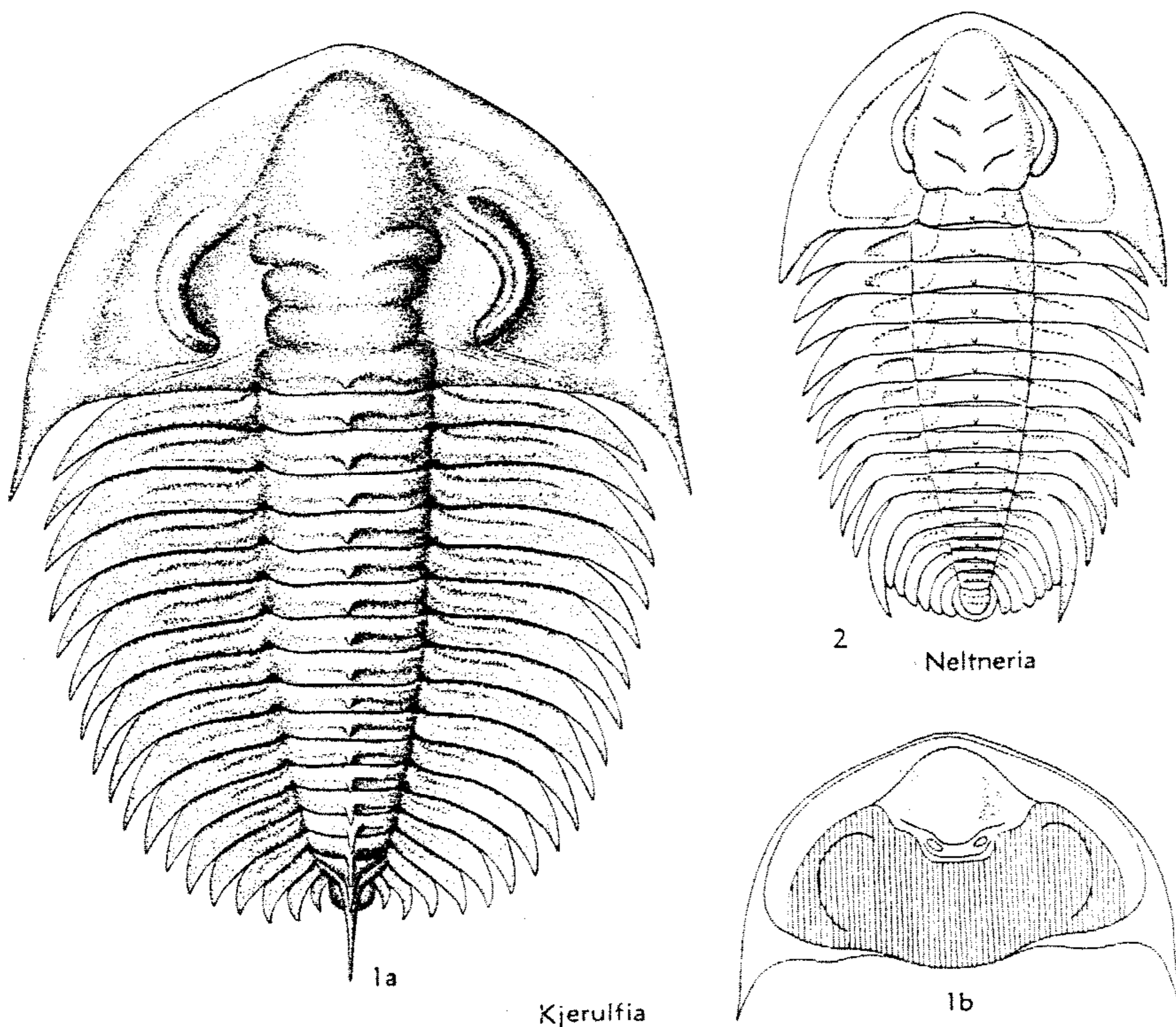
FIG. 137. Olenellidae (Callaviinae, Neltneriinae) (p. 0193-0196).
