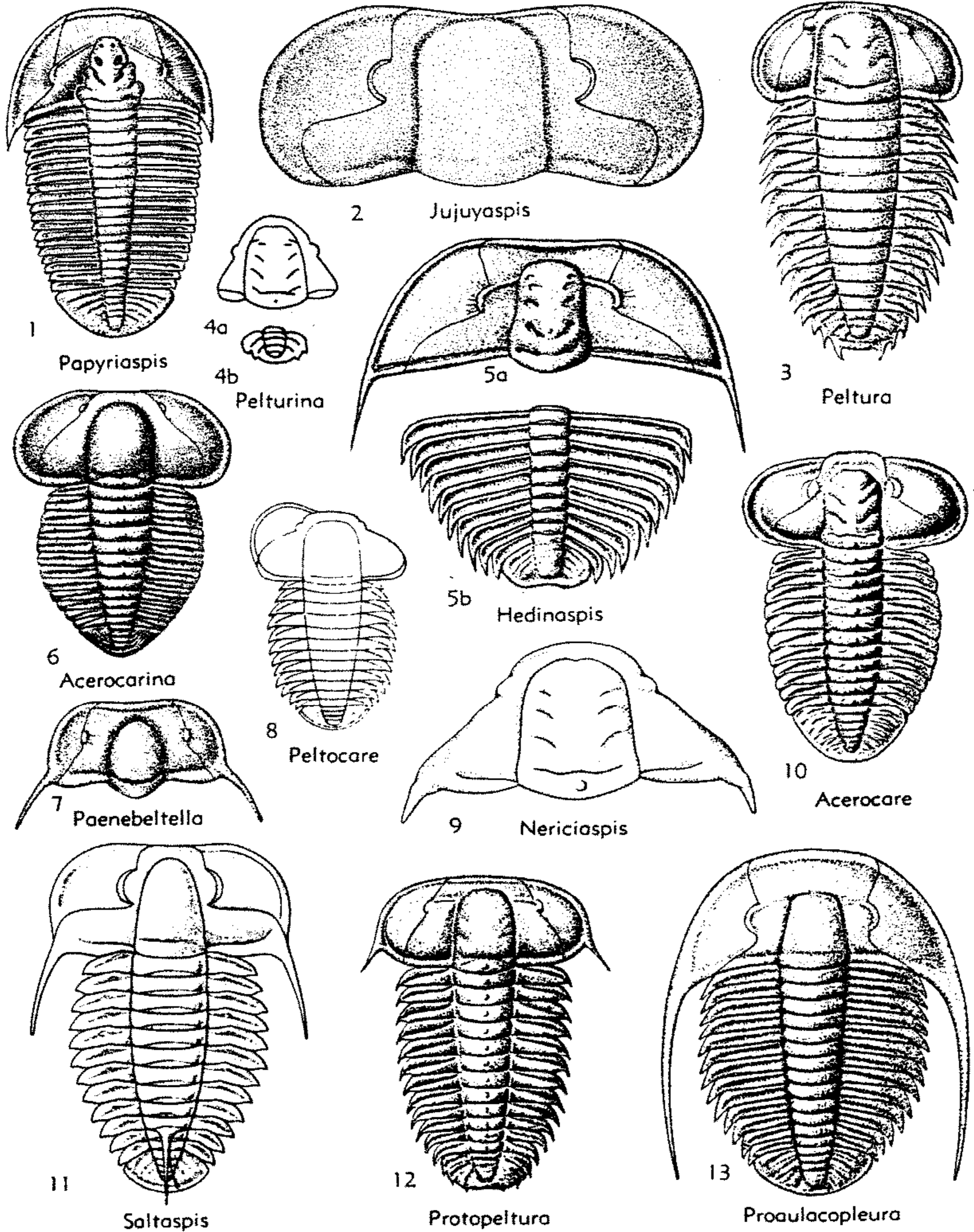
FIG. 196. Olenidae (Pelturinae), Papyriaspididae (p. 0265, 0266, 0269).
