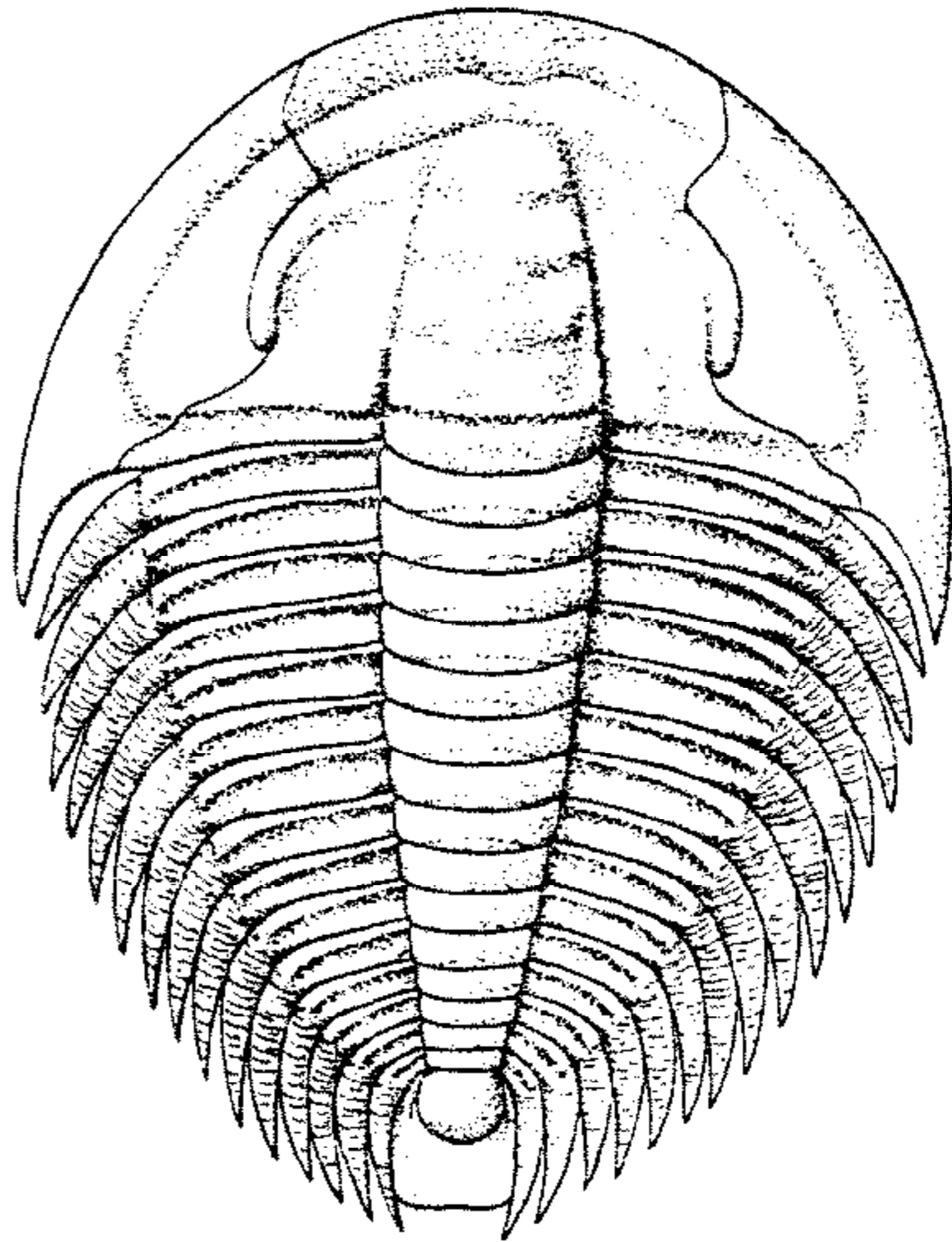
FIG. 147. Dolerolenus zoppii (MENECHINI) LEANZA ( Dolerolenidae ), M.Cam. , Sardinia, \times 3 (380, 488).
