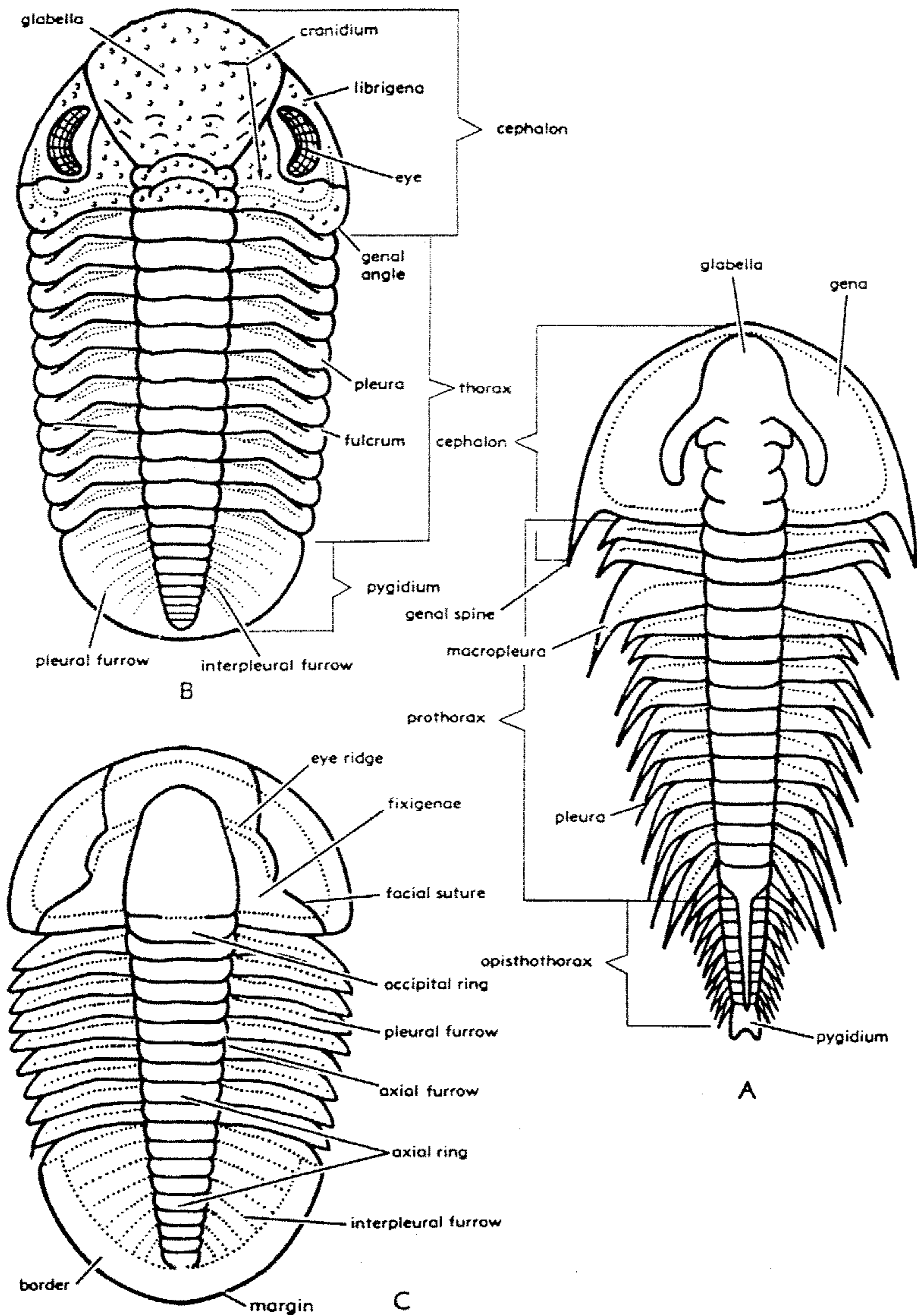
FIG. 28. Nomenclature of exoskeleton.—A. Olenellus vermontanus (HALL) HALL, L.Cam., USA (Vermont), \times 1 (64).—B. Phacops fecundus BARRANDE, Dev., Bohemia, \times 1 (2).—C. Asaphiscus wheeleri MEEK, U.Cam., USA (Utah), \times 1 (488).
