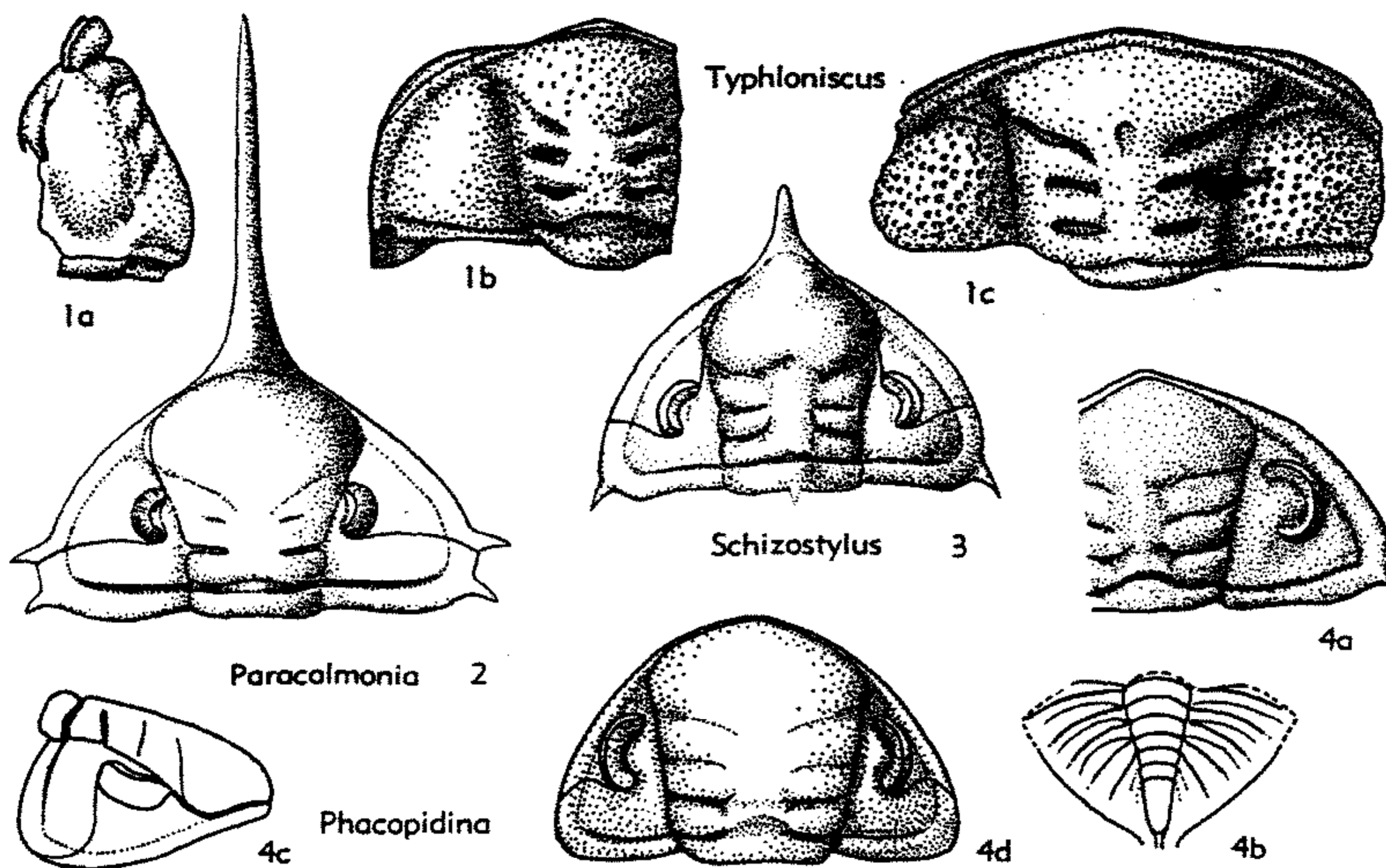
FIG. 385. Calmoniidae (Calmoniinae) (p. 0486-0487).
