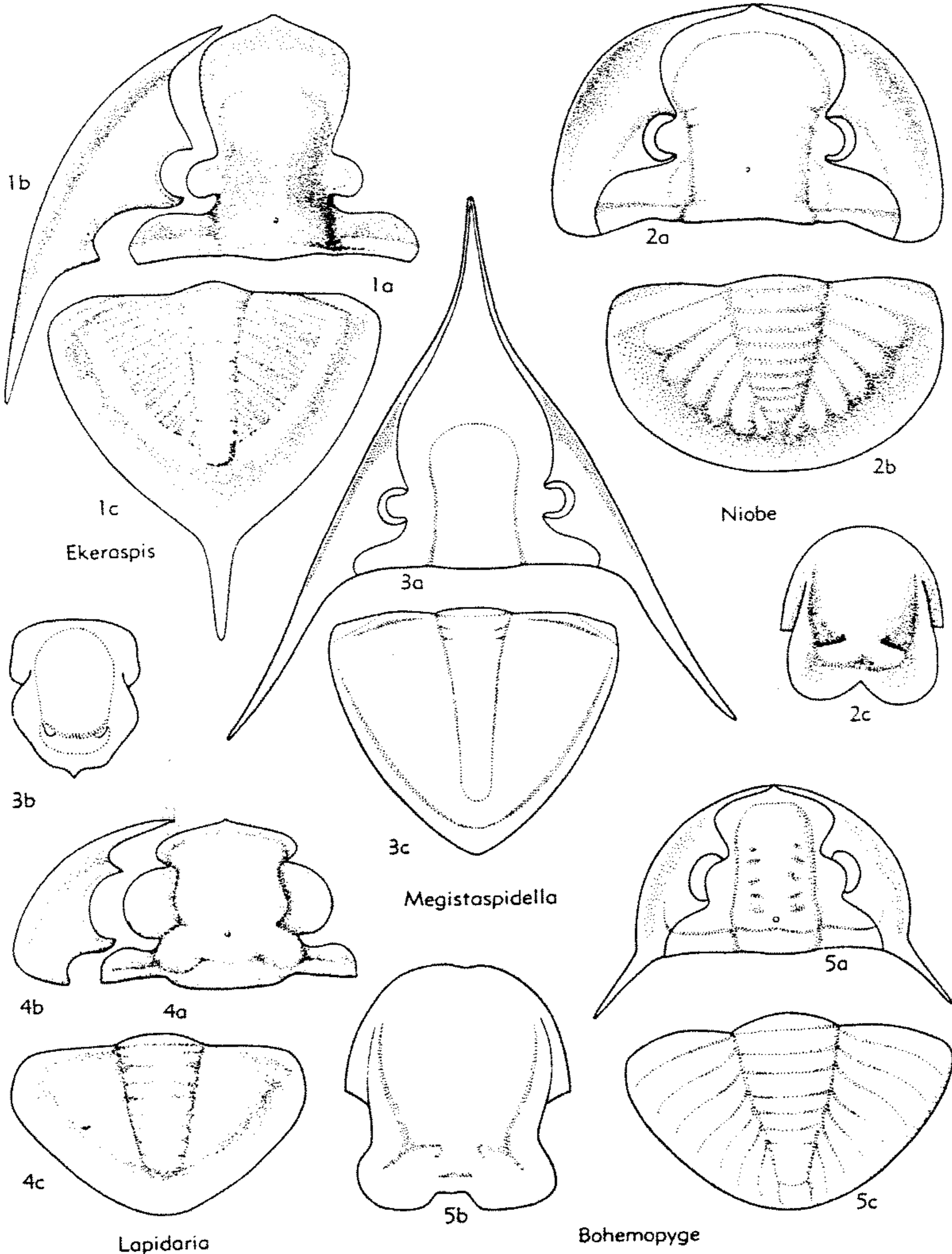
FIG. 259. Asaphidae (Isotelinae, Niobinae) (p. 0349-0350).
