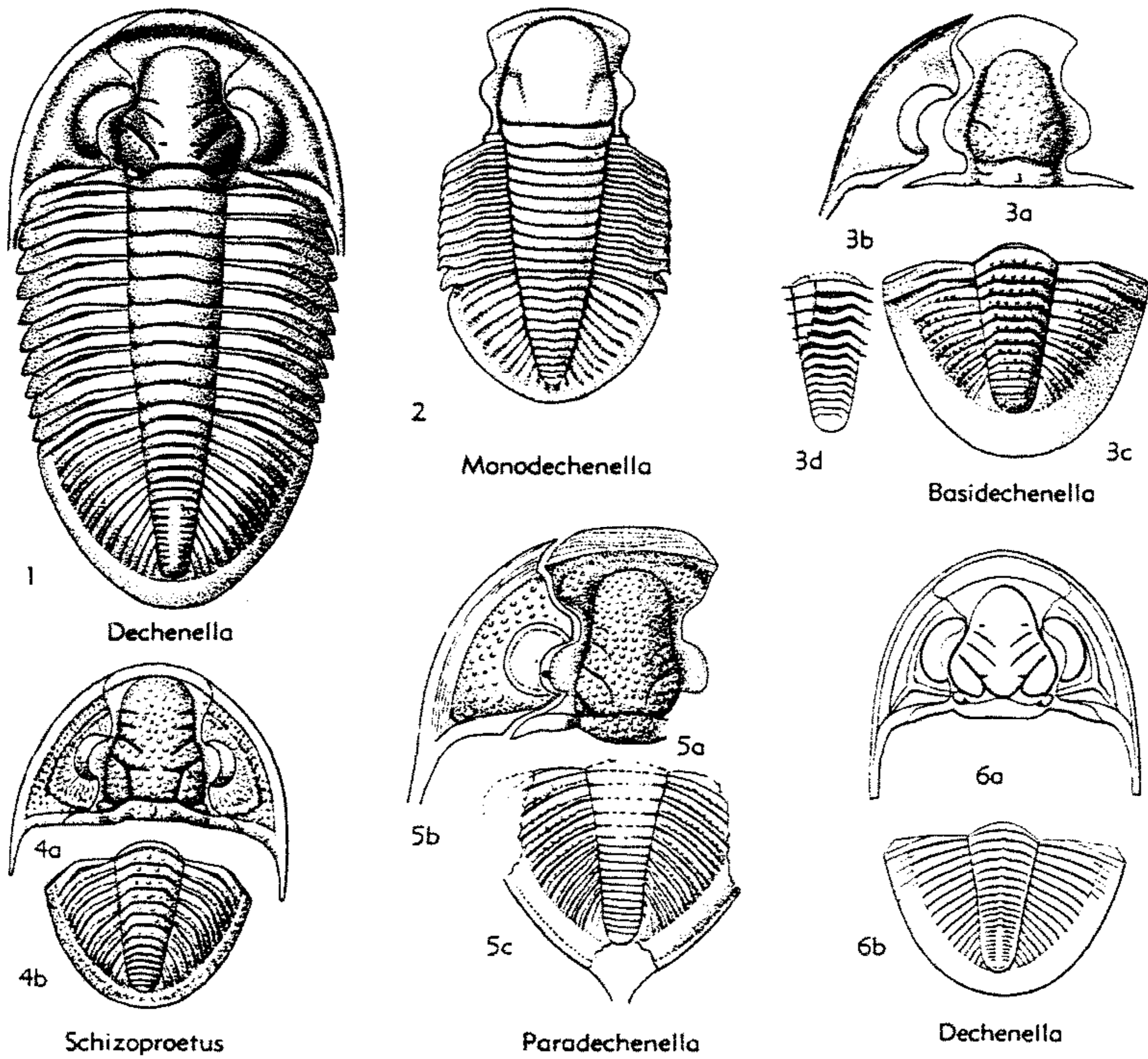
FIG. 297. Proctidae (Dechenellinae) (p. 0388-0389).
