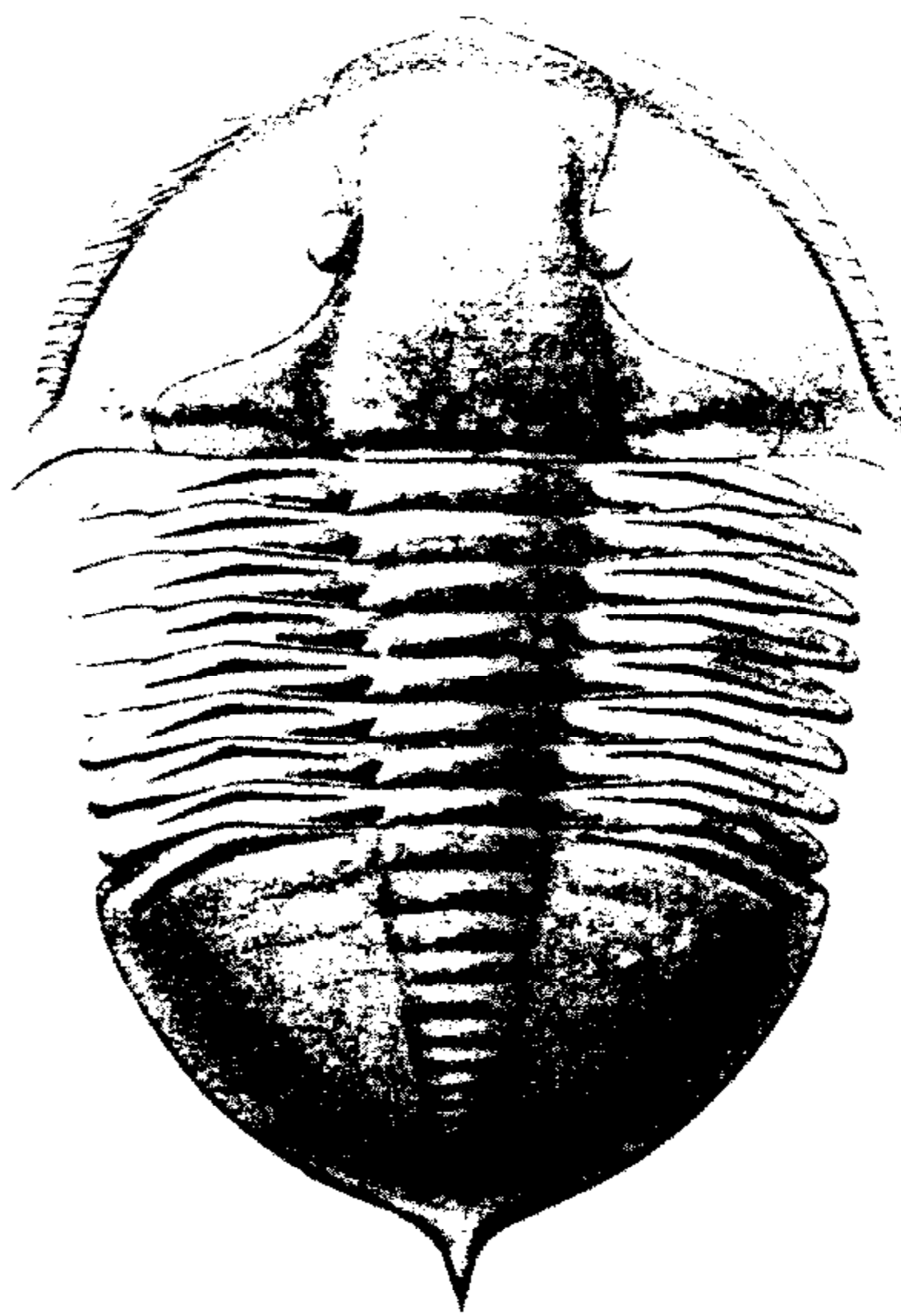
FIG. 258. * Megalaspidella (Kayseraspis) asaphelloides (HARRINGTON) (Asaphidae), L.Ord.(Arenig.), Arg.; carapace (reconstr.), \times 1.8 (59*).
