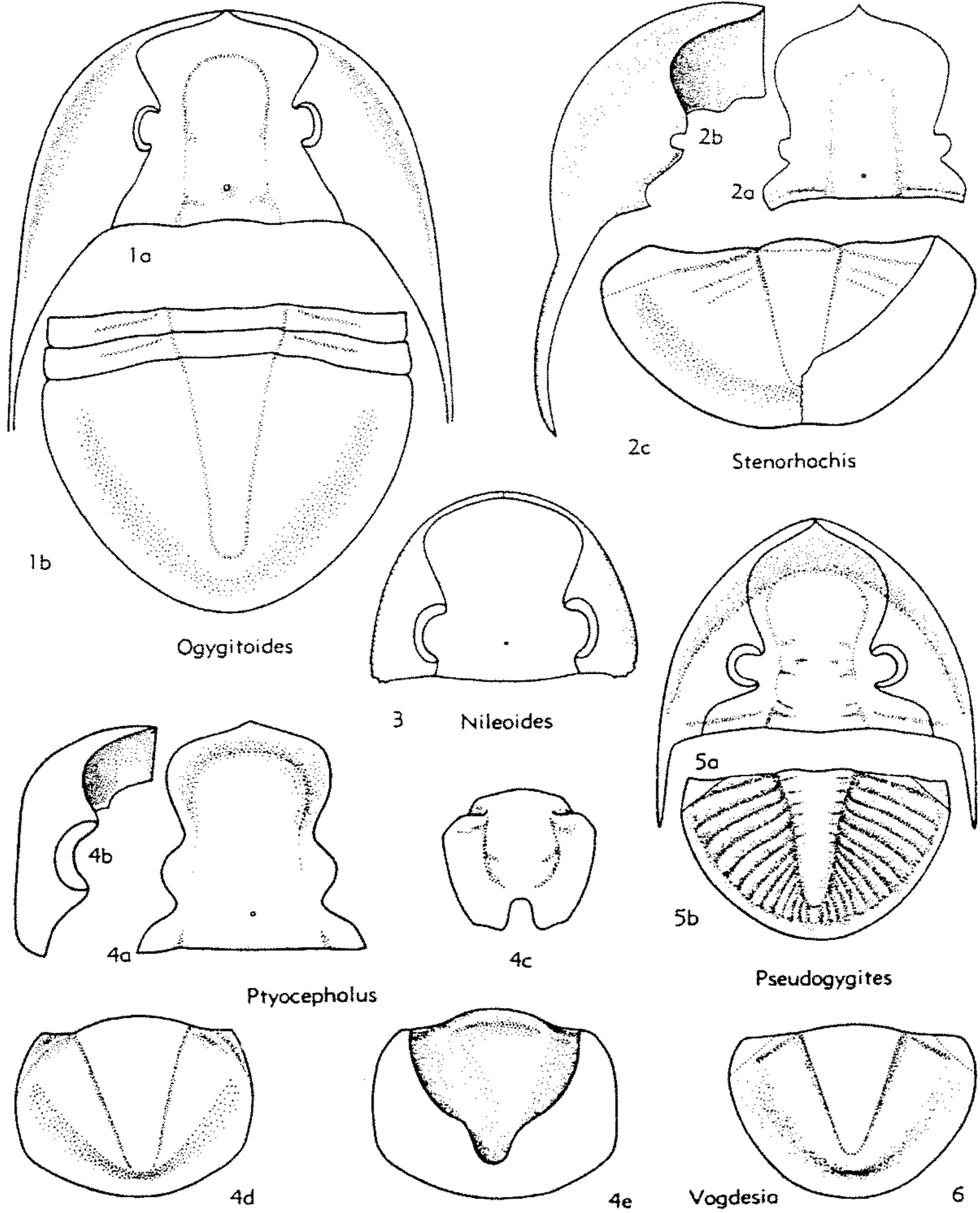
FIG. 253. Asaphidae (Isotelinae) (p. 0341-0344).
