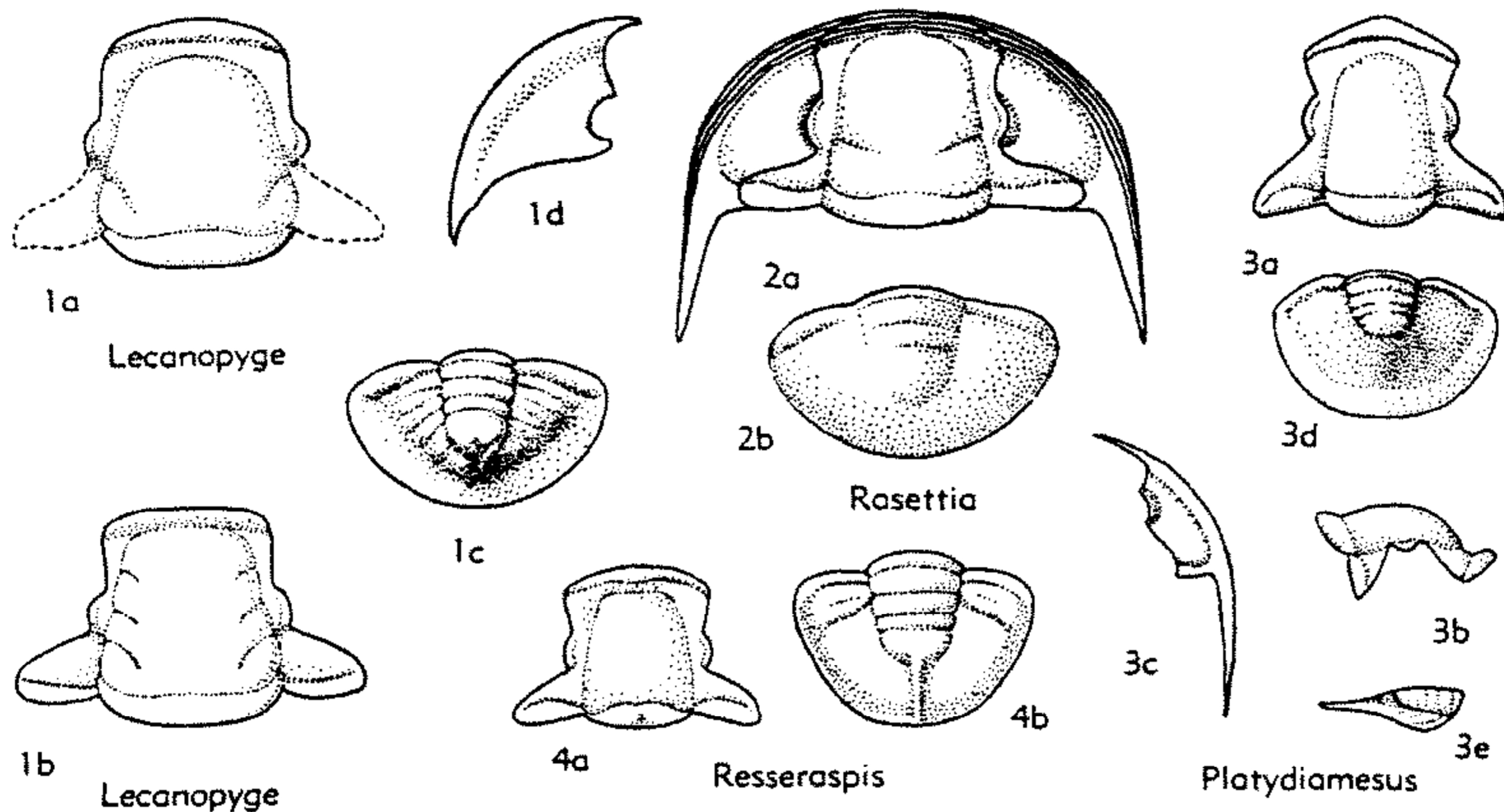
FIG. 287. Lecanopygidae (p. O380-O381).
