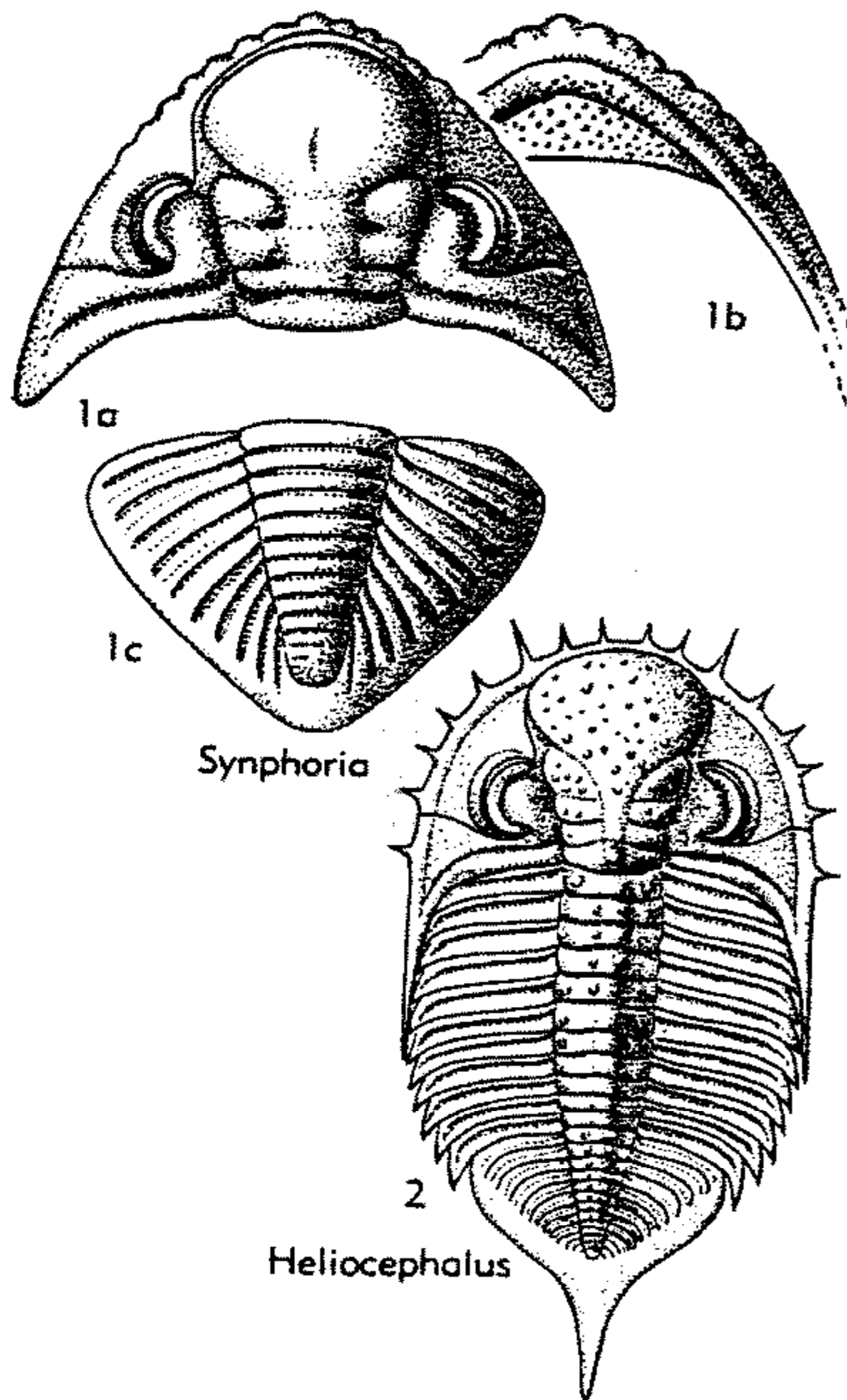
FIG. 373. Dalmanitidae (Dalmanitinae) (p. 0470-0472).
