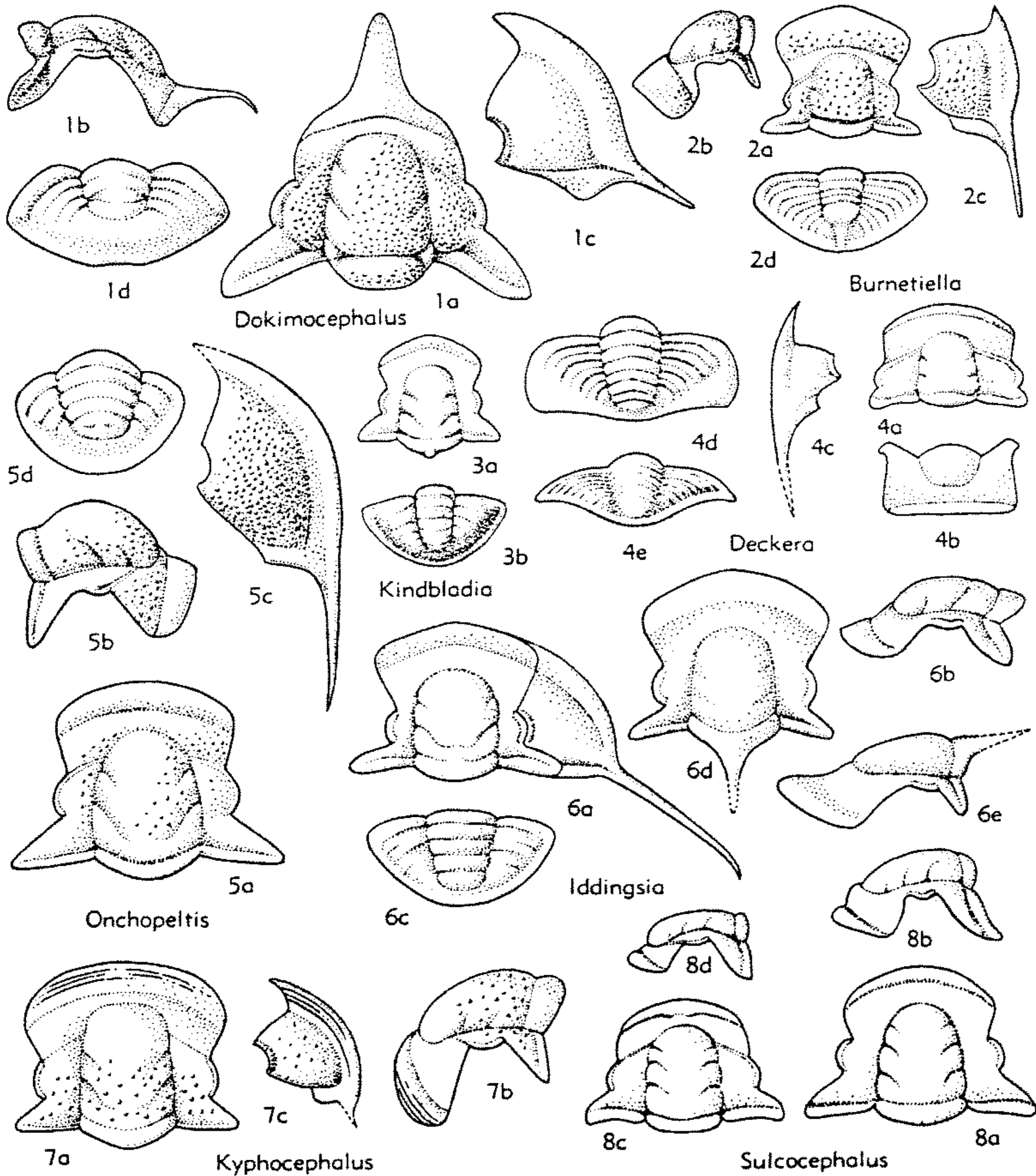
FIG. 208. Dokimocephalidae (p. O281-O283).
