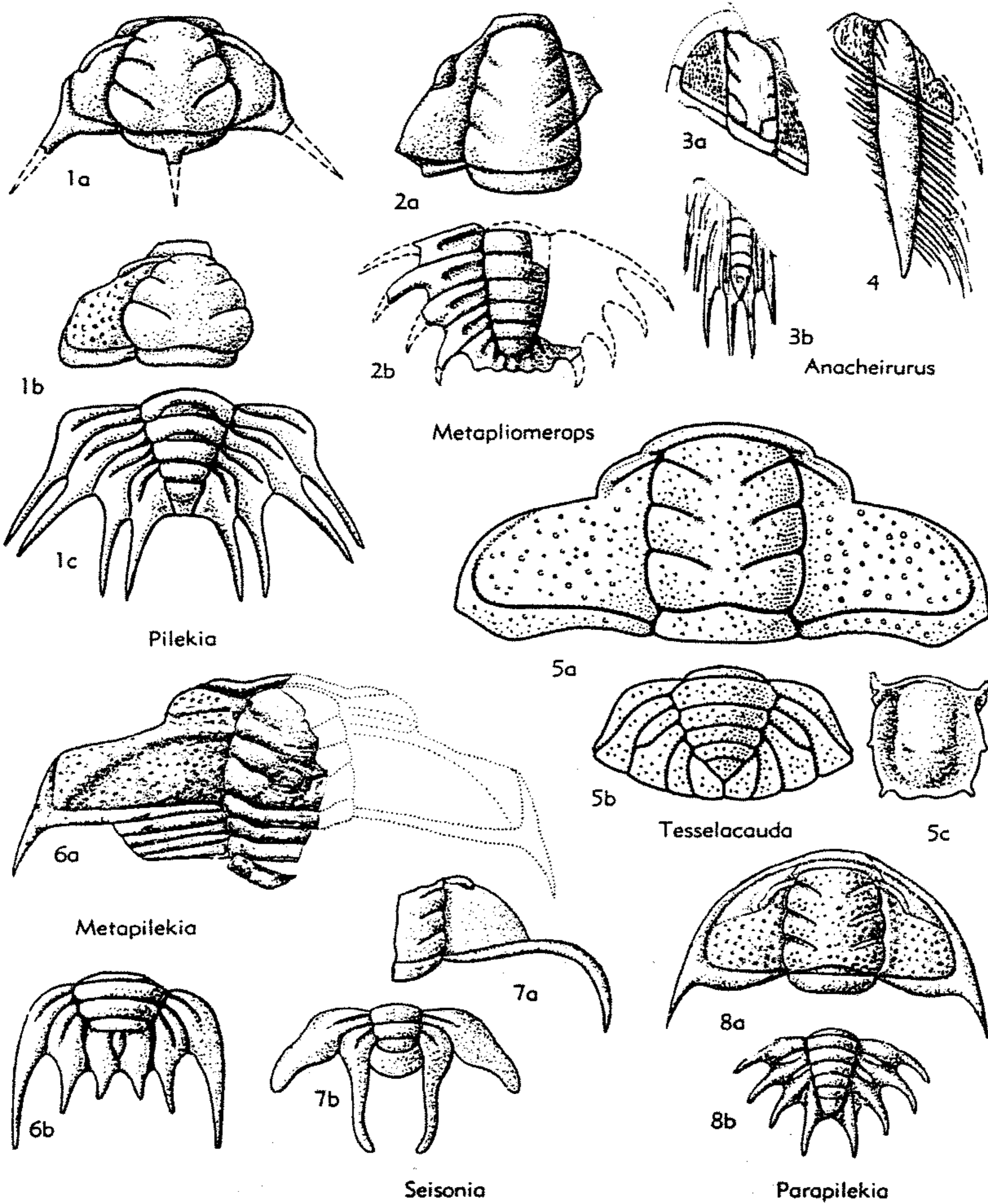
FIG. 346. Pliomeridae (Pilekiinae) (p. 0441).
