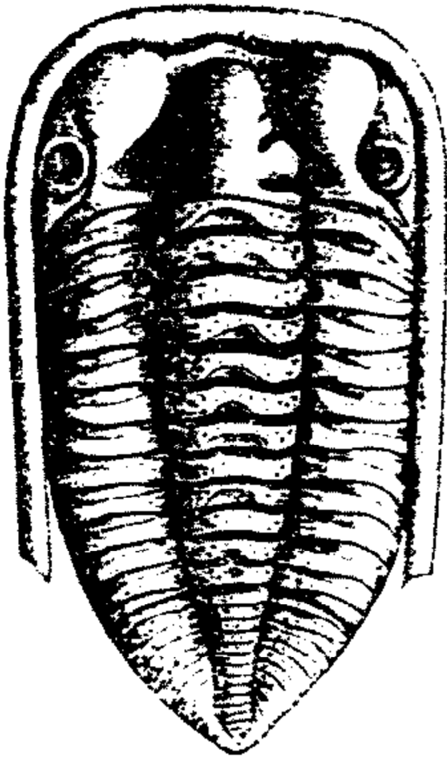
FIG. 355. * Bathyscheilus perplexus (BARRANDE) (Calymenidae), M.Ord. (Llanvirn.), Boh.; exoskel., \times 2 (66).
