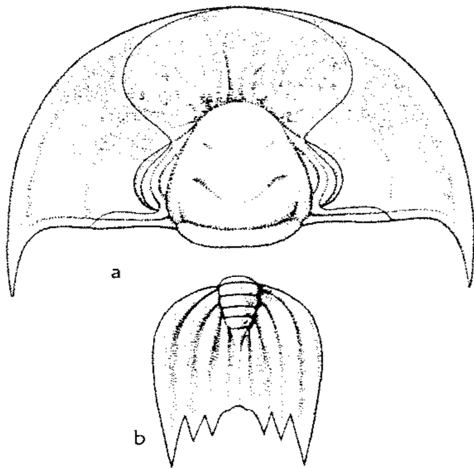
FIG. 247. * Hungaia magnifica (BILLINGS) (Hungaiidae), U.Cam.(Trempeal.), Que.; a,b, ceph., pyg., \times 0.7 (79).
