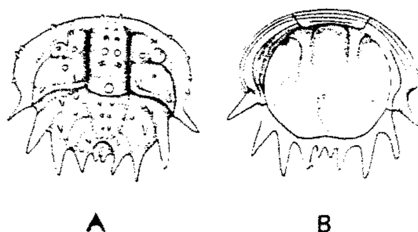
FIG. 95. Lichid protaspis, L.Dev., E.USA (N.Y.); A,B, dorsal, ventral, \times 20 (35*).
