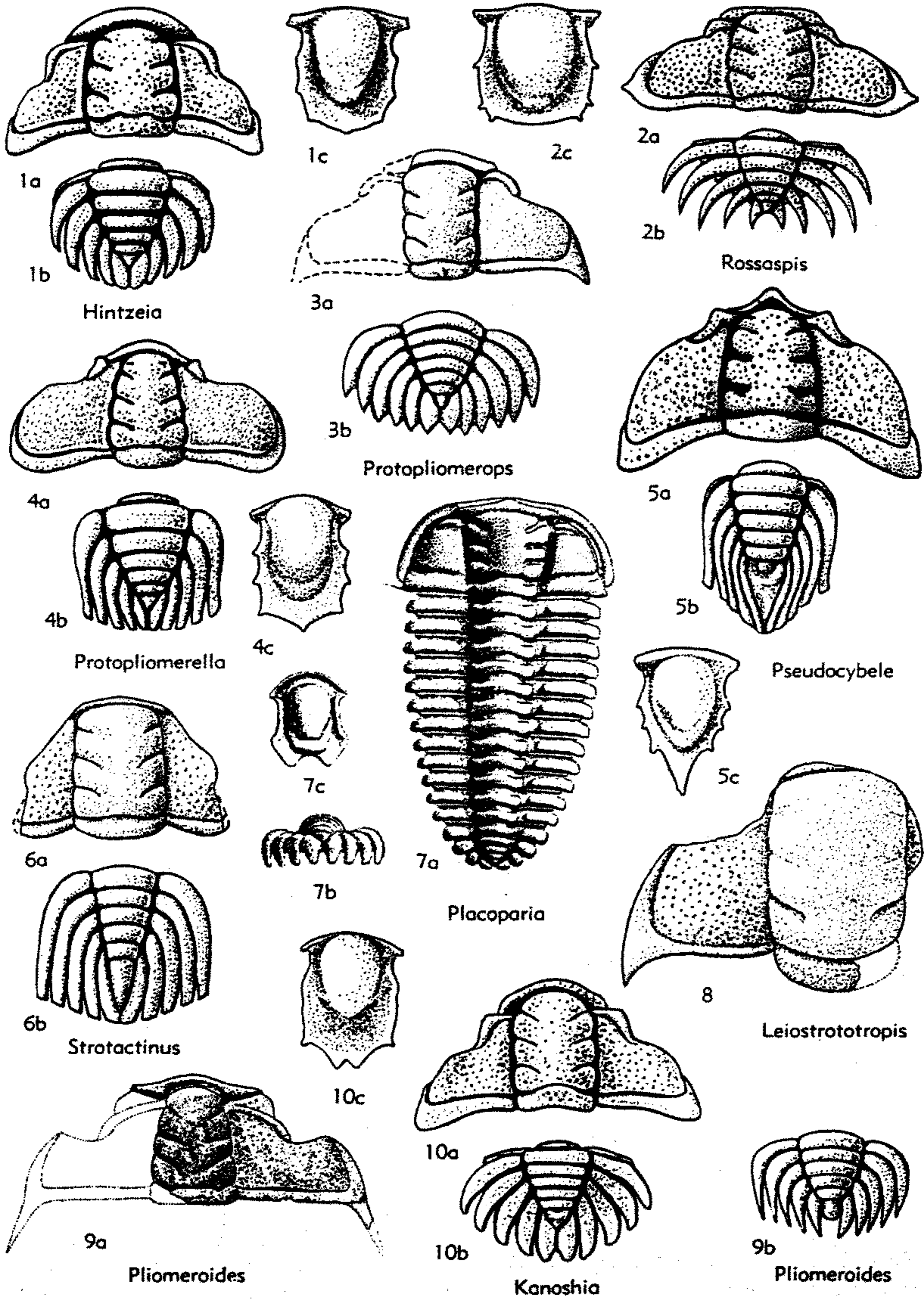
FIG. 347. Pliomeridae (Protopliomeropinae, Placopariinae) (p. 0444-0445).
