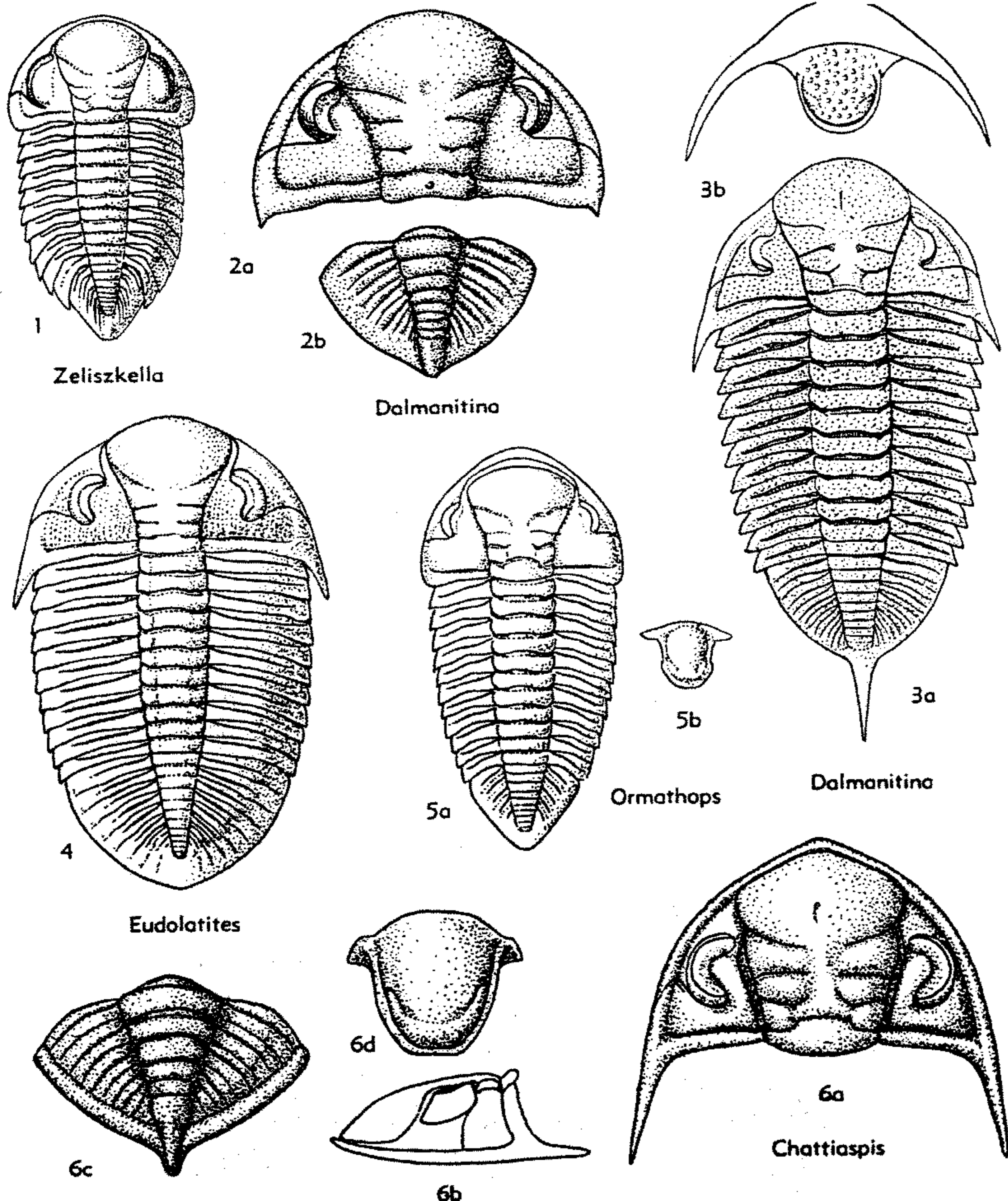
FIG. 375. Dalmanitidae (Zeliszellinae) (p. 0473-0475).
