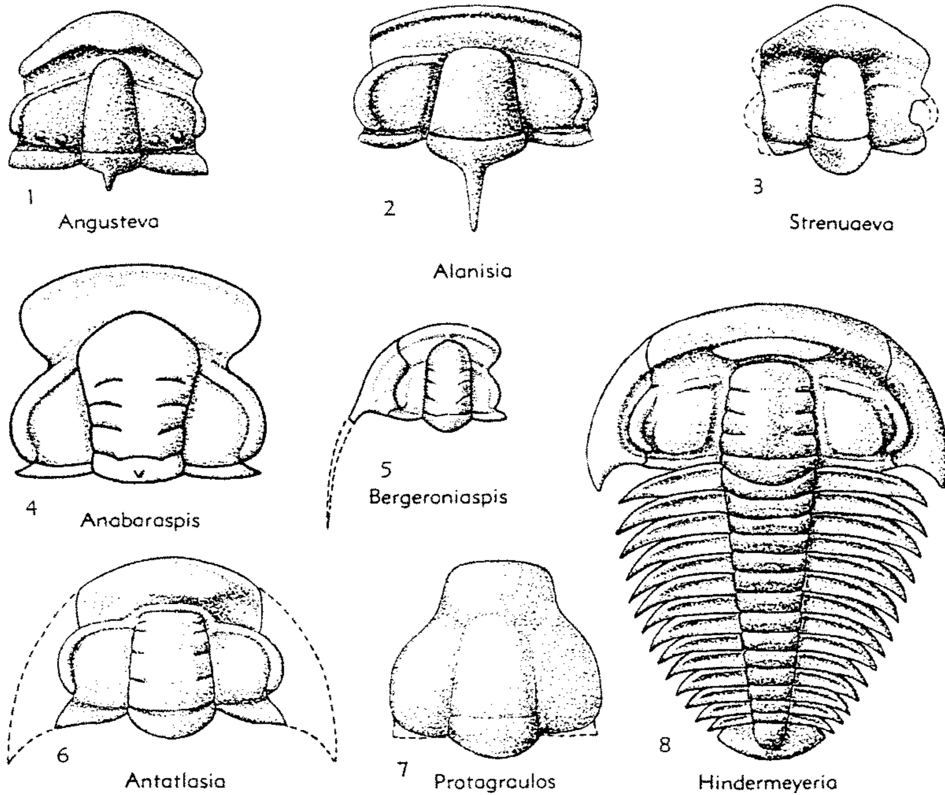
FIG. 149. Ellipsocephalidae (Antatlasinae, Ellipsocephalinae), Protolenidae (Protoleninae) (p. O207-O212).
