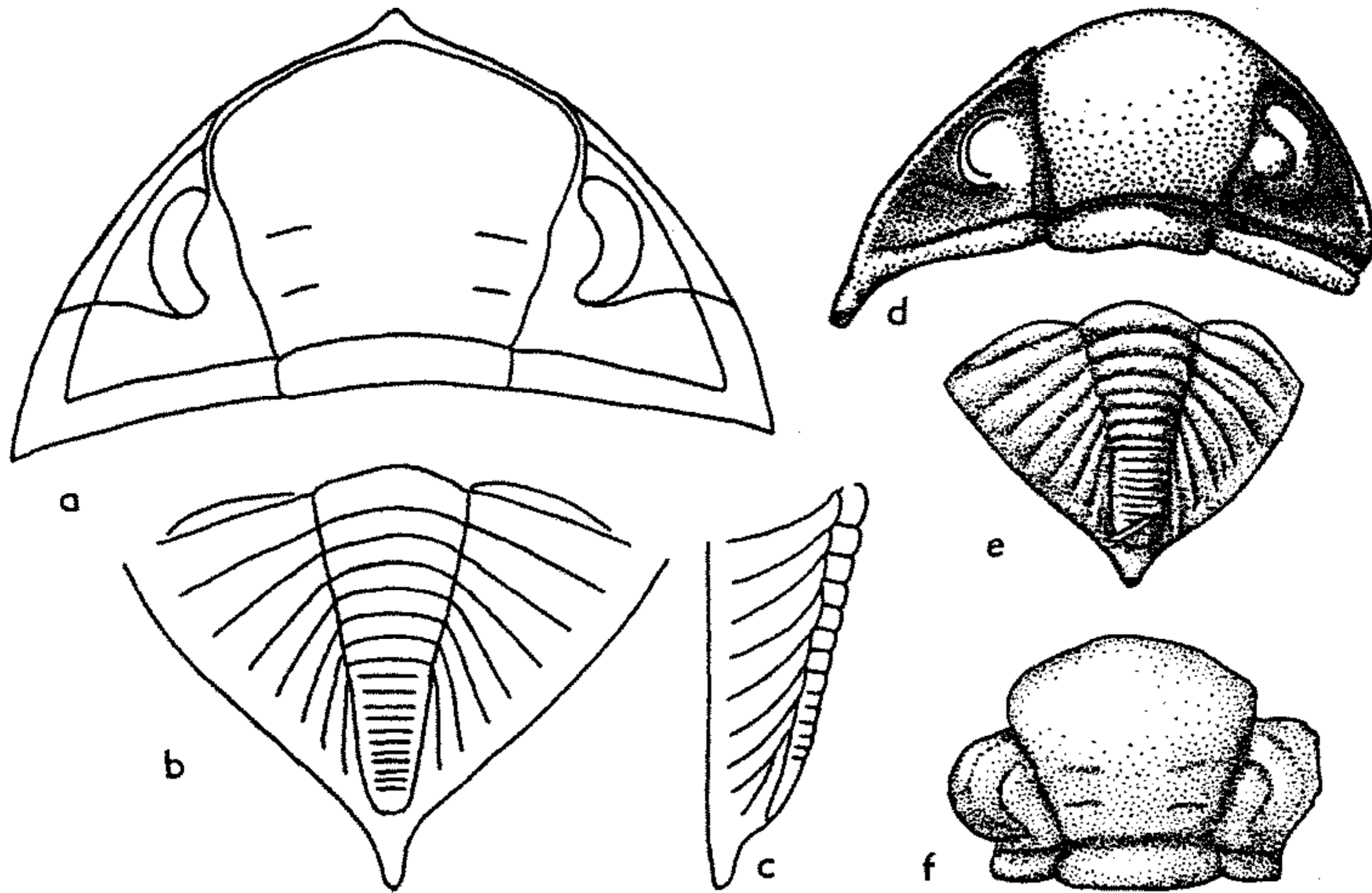
FIG. 384. Dalmaniturus (Calmoniidae) (p. O485).
