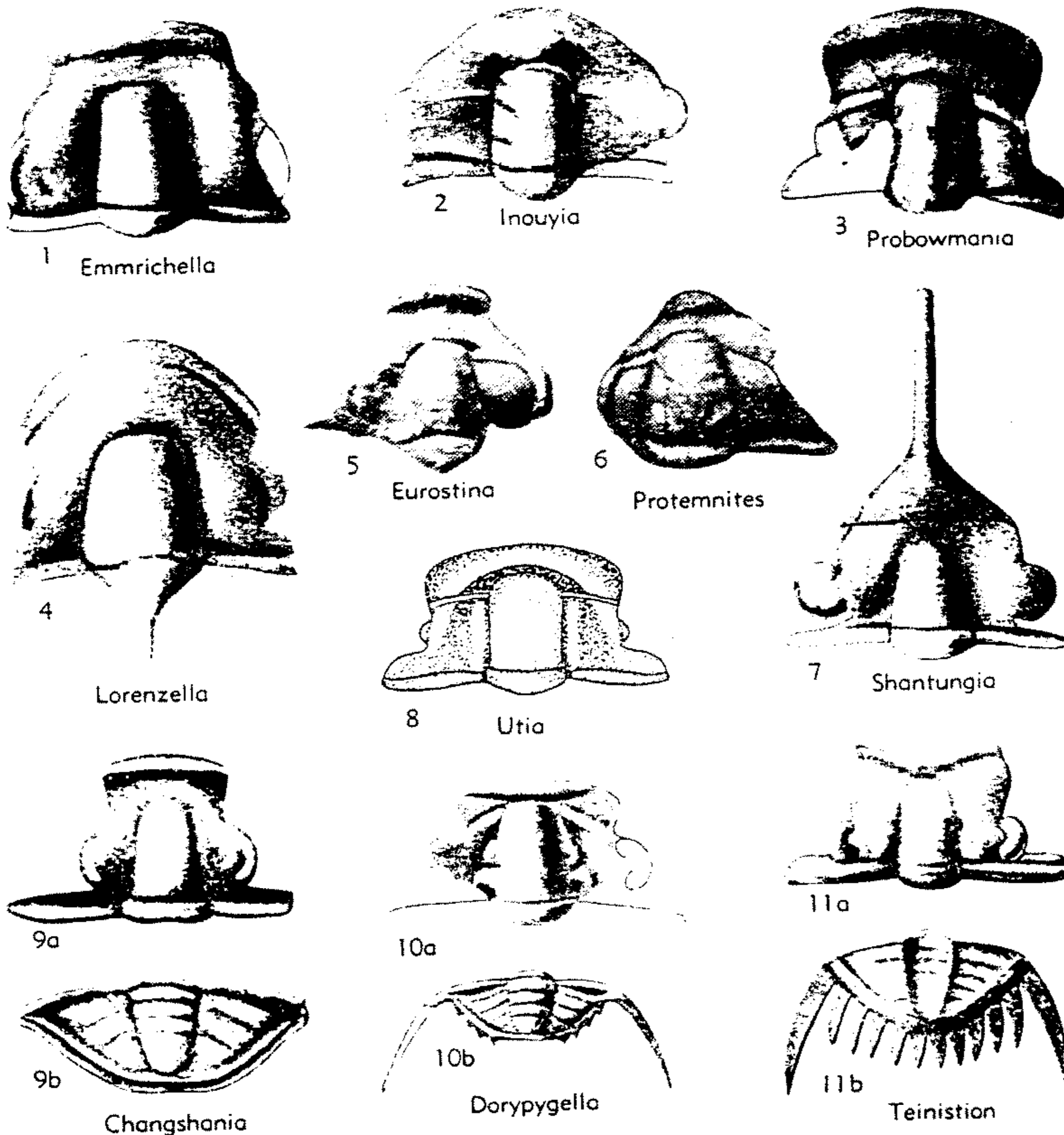
FIG. 185. Emmrichellidae (p. O247, O248).
