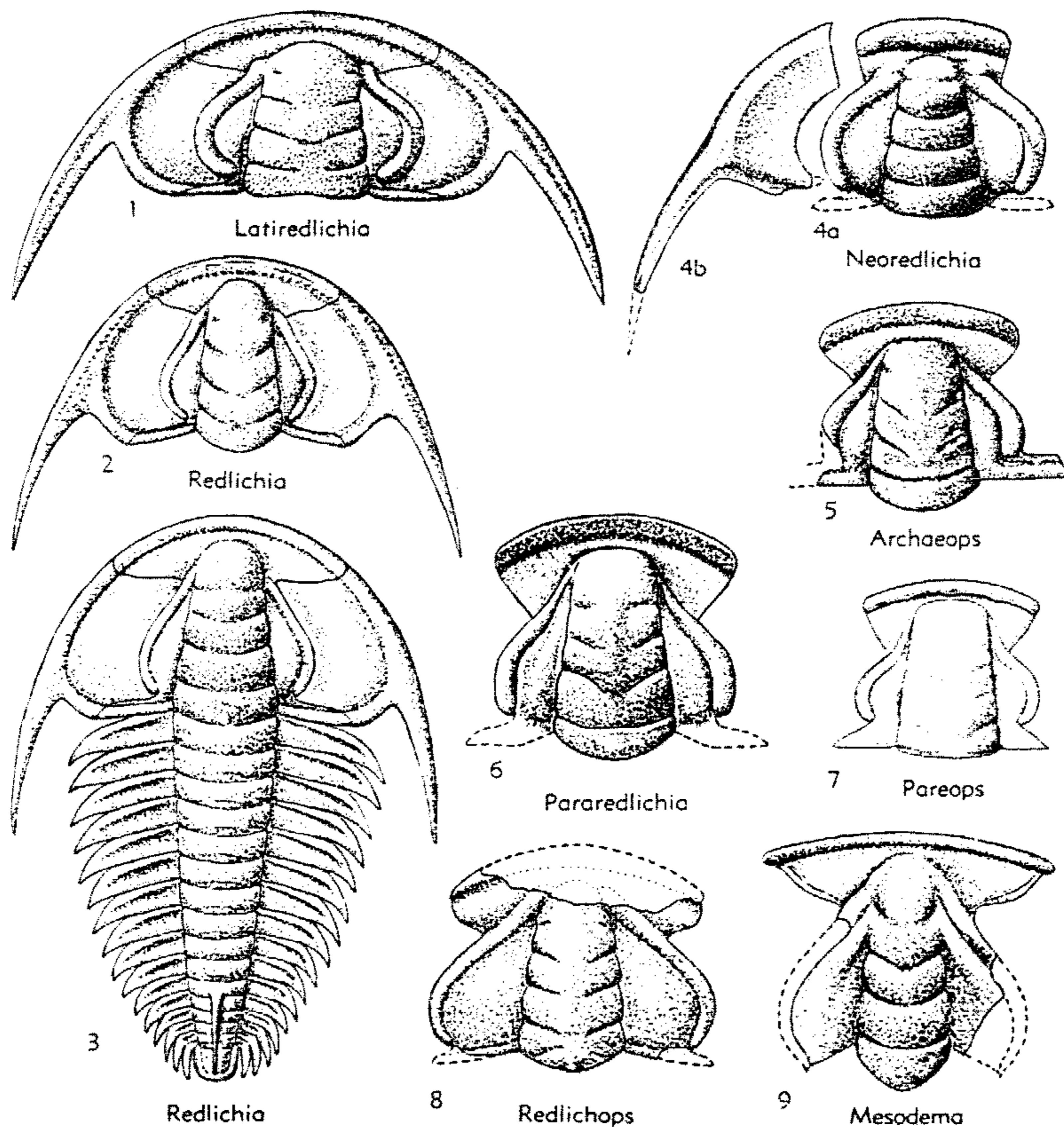
FIG. 141. Redlichiidae (Redlichiinae, Pararedlichiinae), Neoredlichiidae (p. 0200, 0201).
