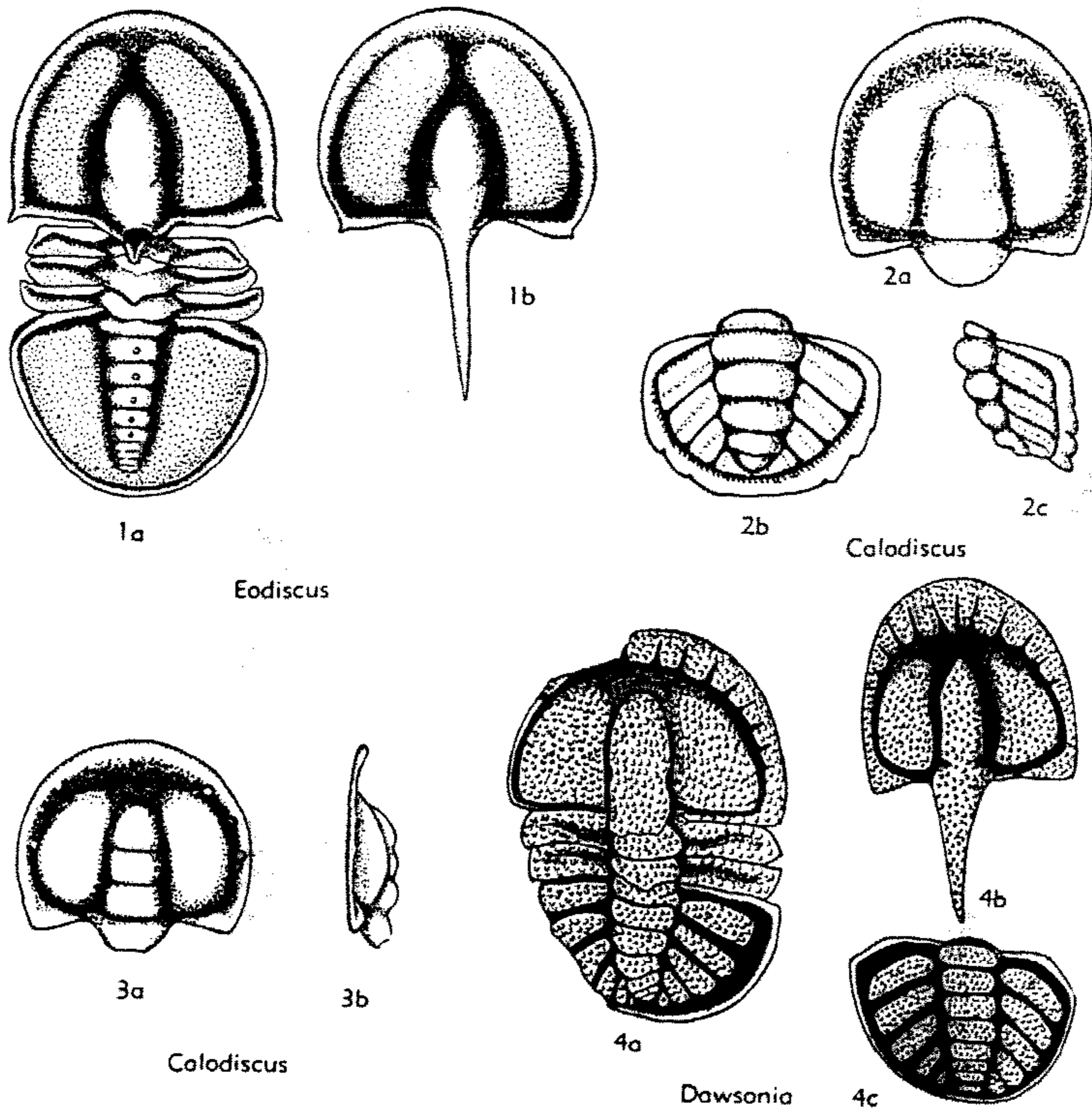
FIG. 129. Eodiscidae (p. O188).
