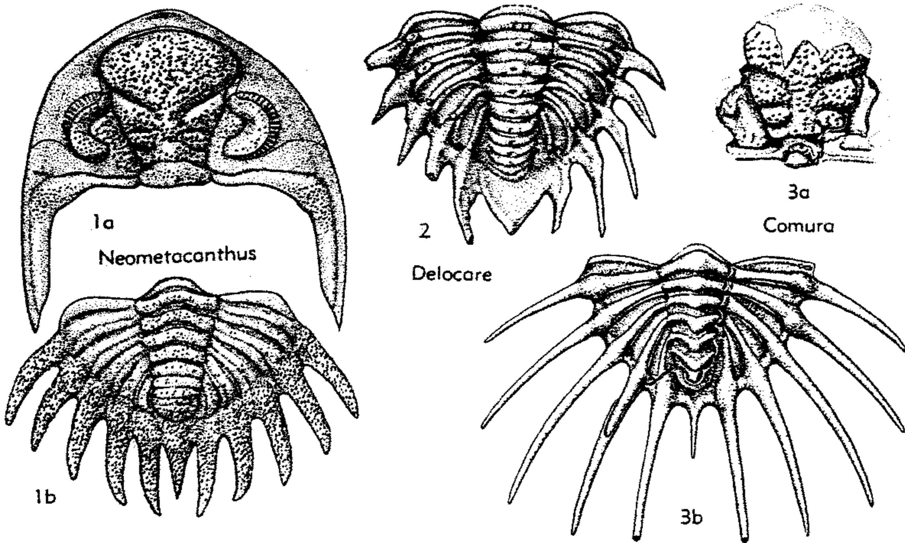
FIG. 380. Dalmanitidae (Asteropyginae) (p. 0479-0480).
