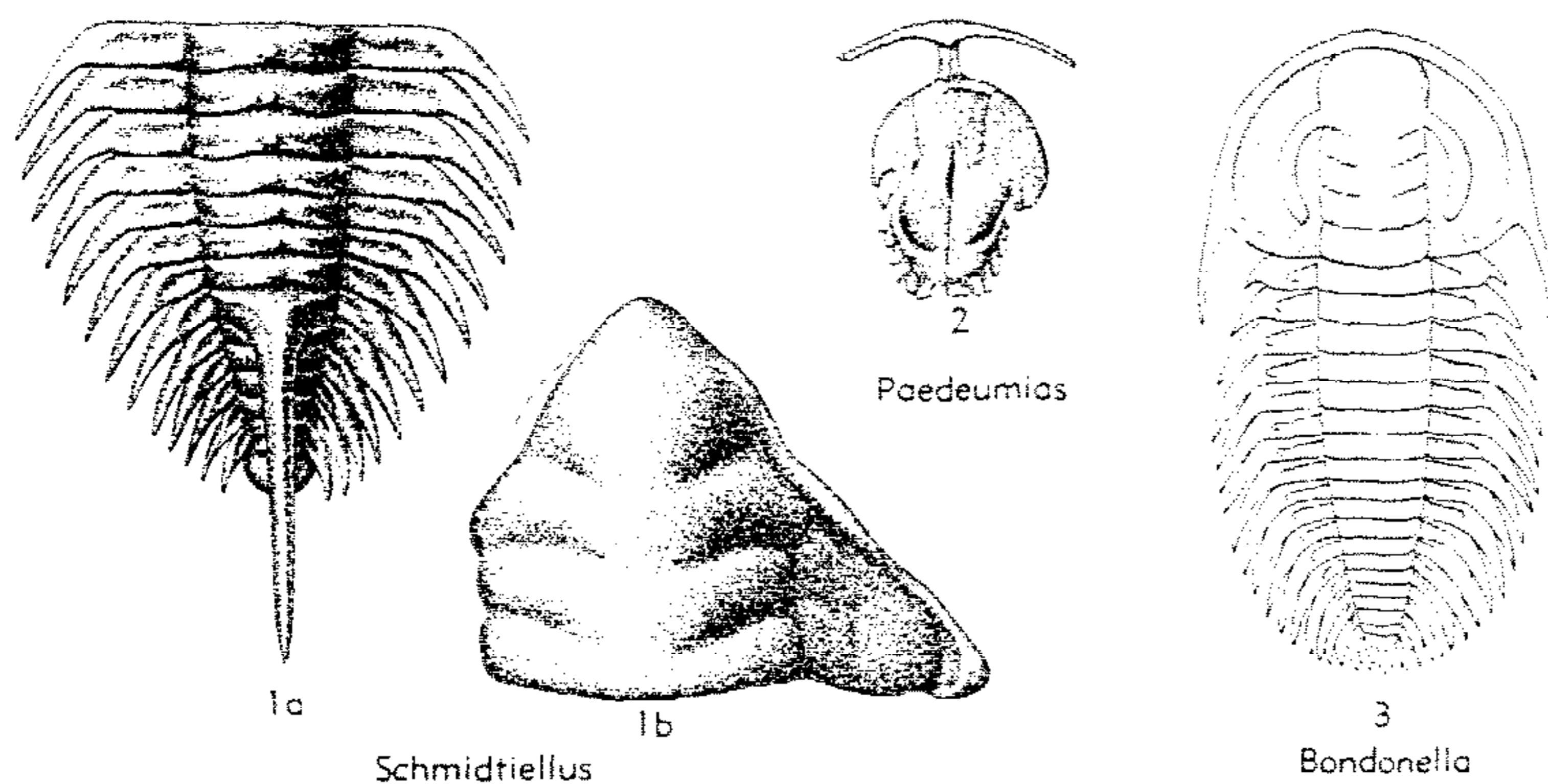
FIG. 138. Olenellidae (Olenellinae, Holmiinae) (p. 0192-0195).
