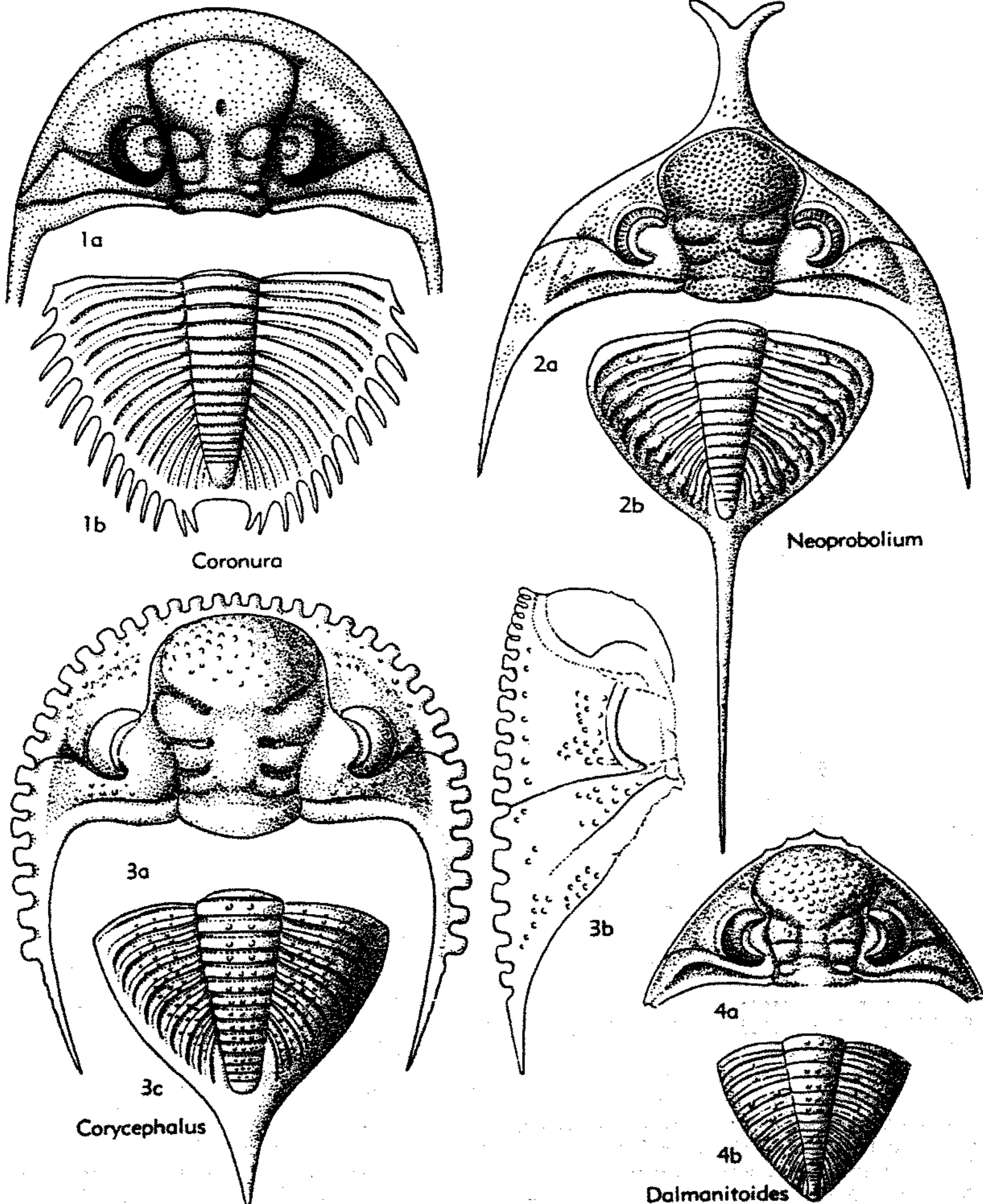
FIG. 372. Dalmanitidae (Dalmanitinae) (p. 0470-0472).
