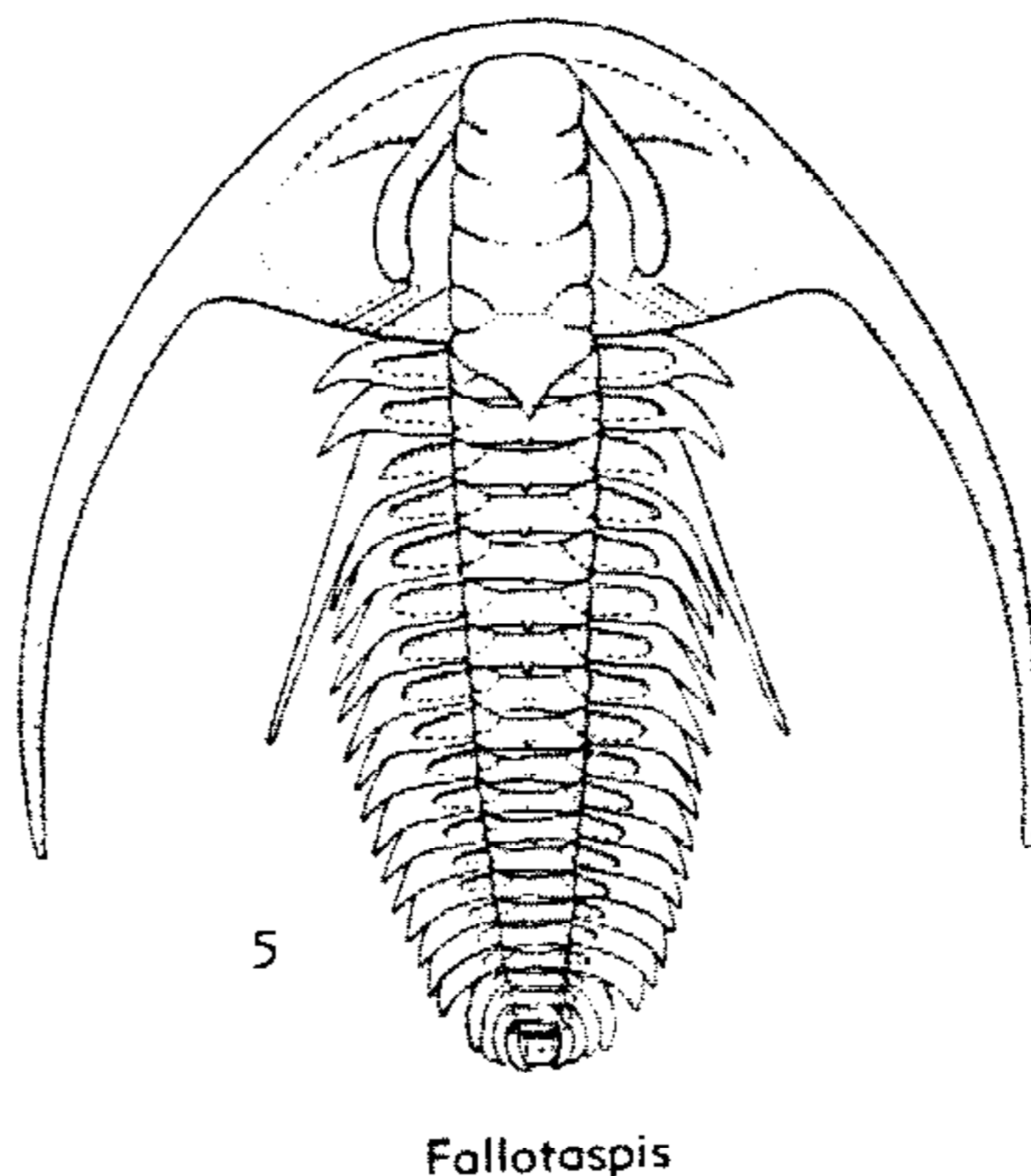
FIG. 133. Olenellidae (Olenellinae, Callaviinae, Fallotaspidinae) (p. 0192-0194).
