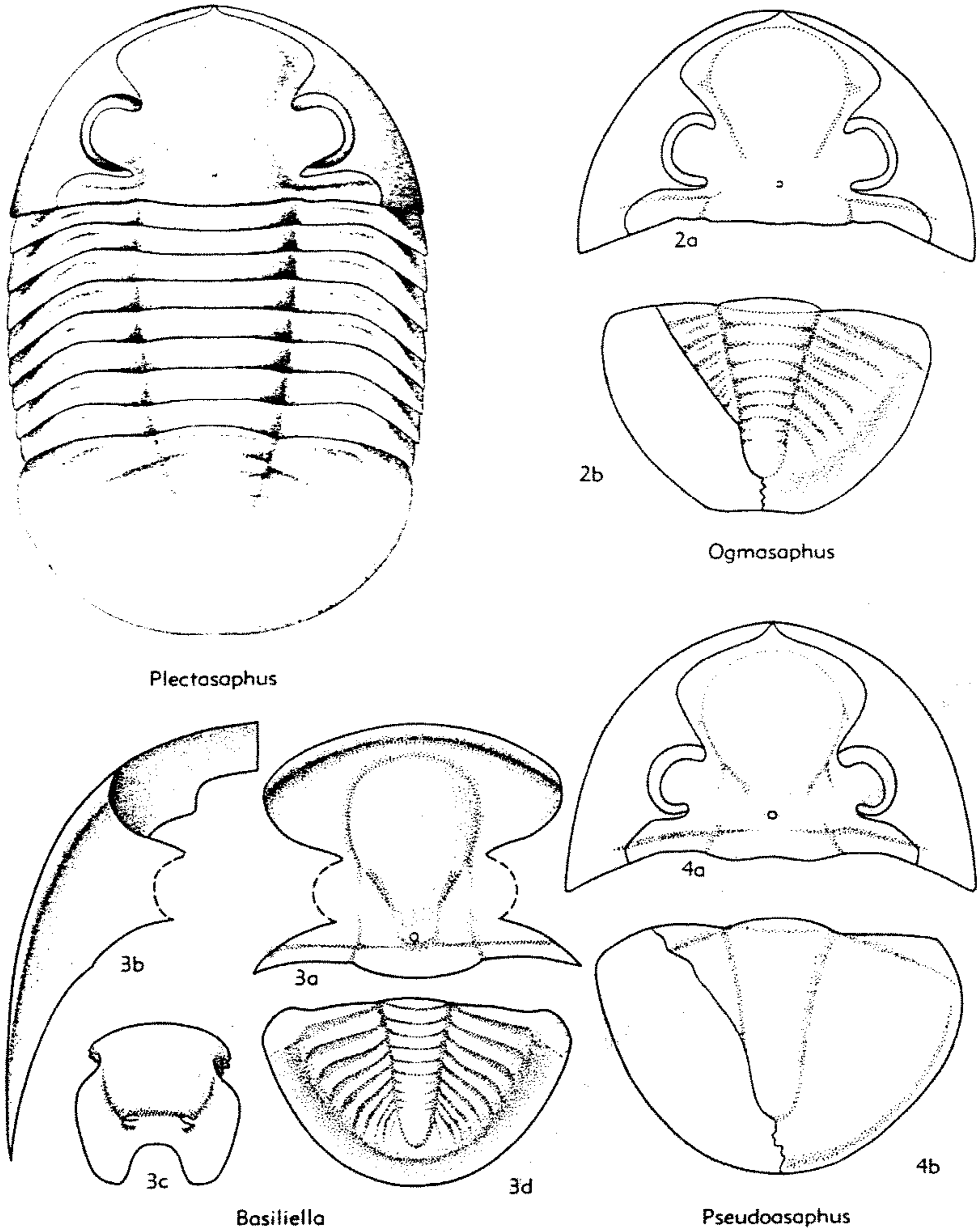
FIG. 249. Asaphidae (Asaphinae) (p. 0336-0337).
