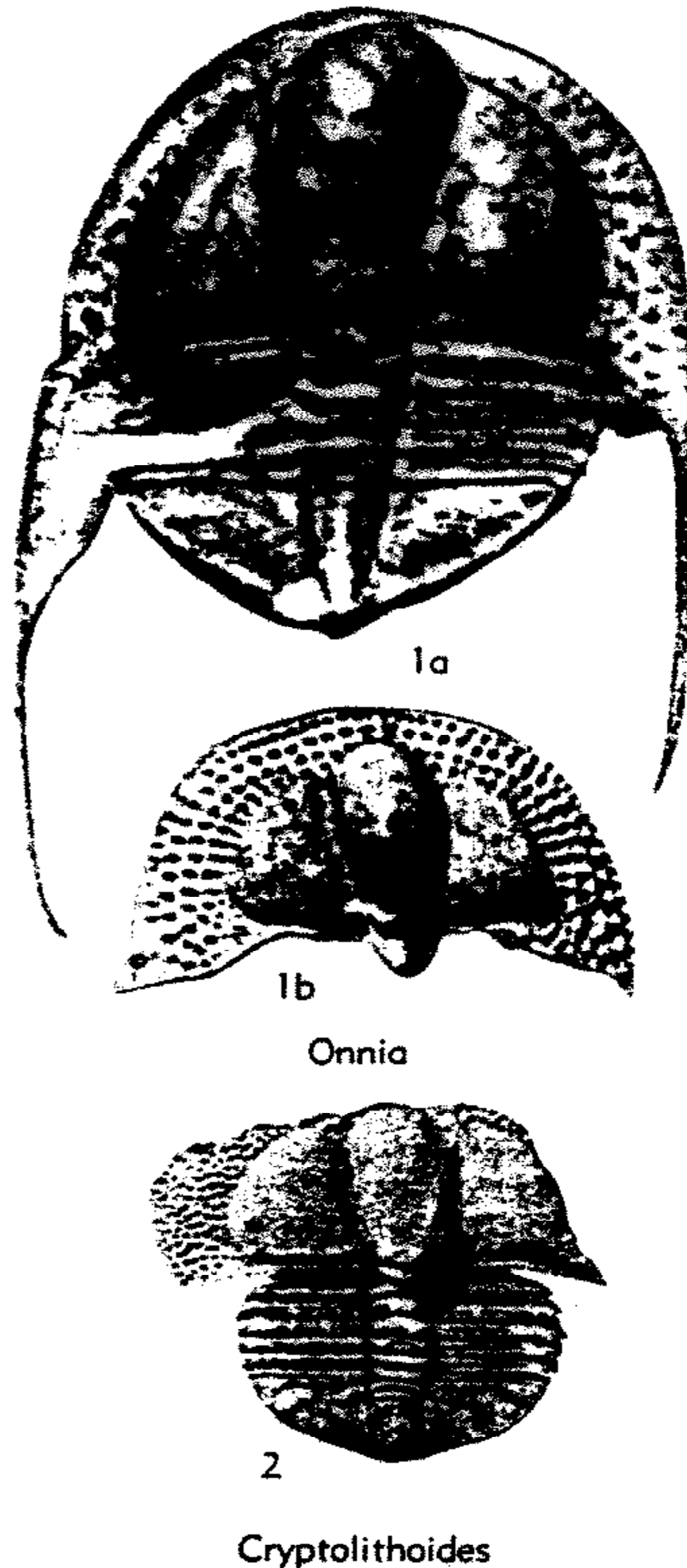
FIG. 325. Trinucleidae (Cryptolithinae) (p. 0422).
