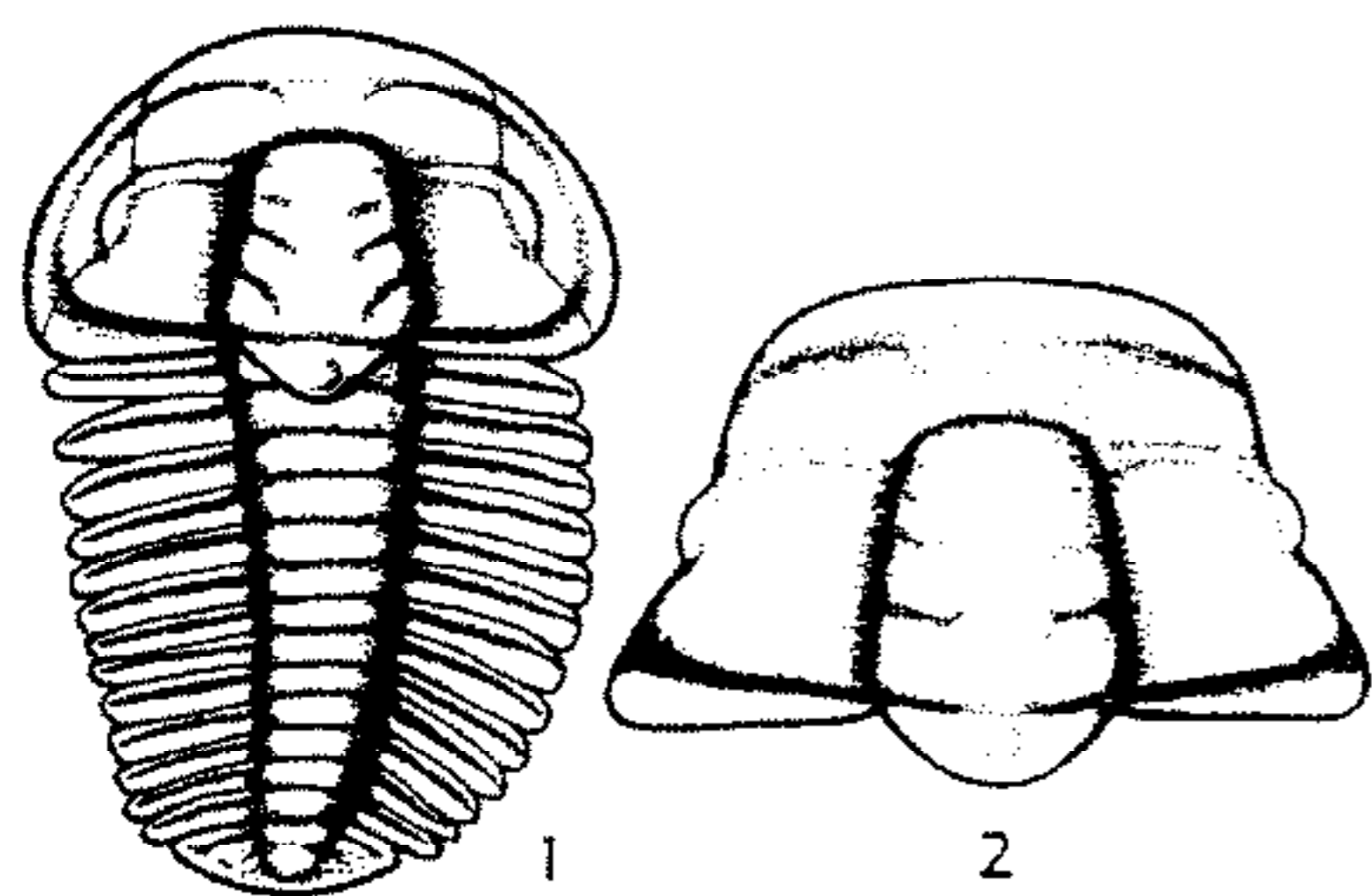
FIG. 171. Ptychopariidae (Antagminae). 1, Syspancephalus gregarius RASETTI, M.Cam., W.Can.(B.C.); exoskel., \times 5 (448n). 2, S. charops (WALCOTT), L.Cam., W.Can.(B.C.); cran., \times 6 (448n).
