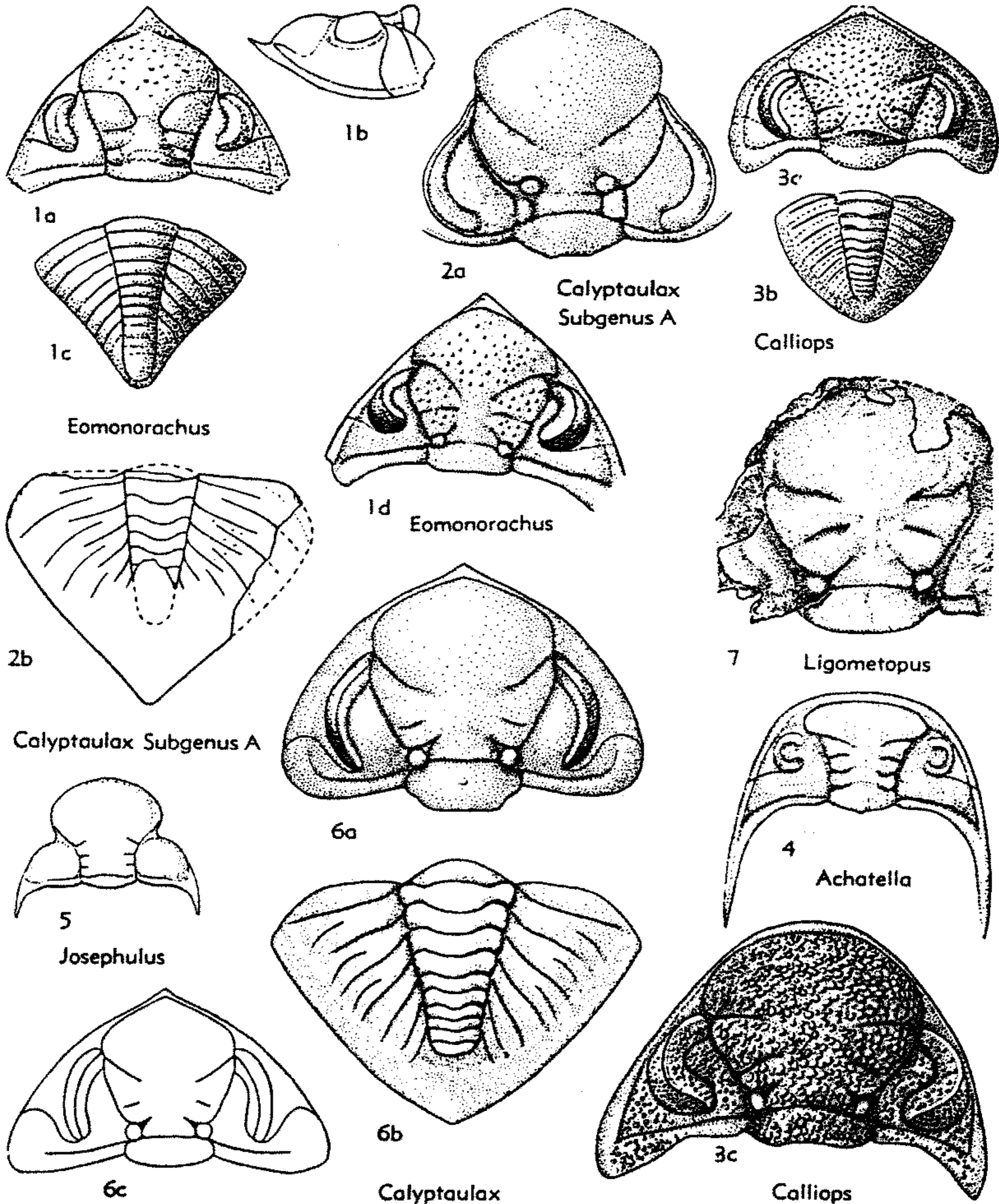
FIG. 389. Pterygometopidae (Pterygometopinac) (p. 0491-0492).
