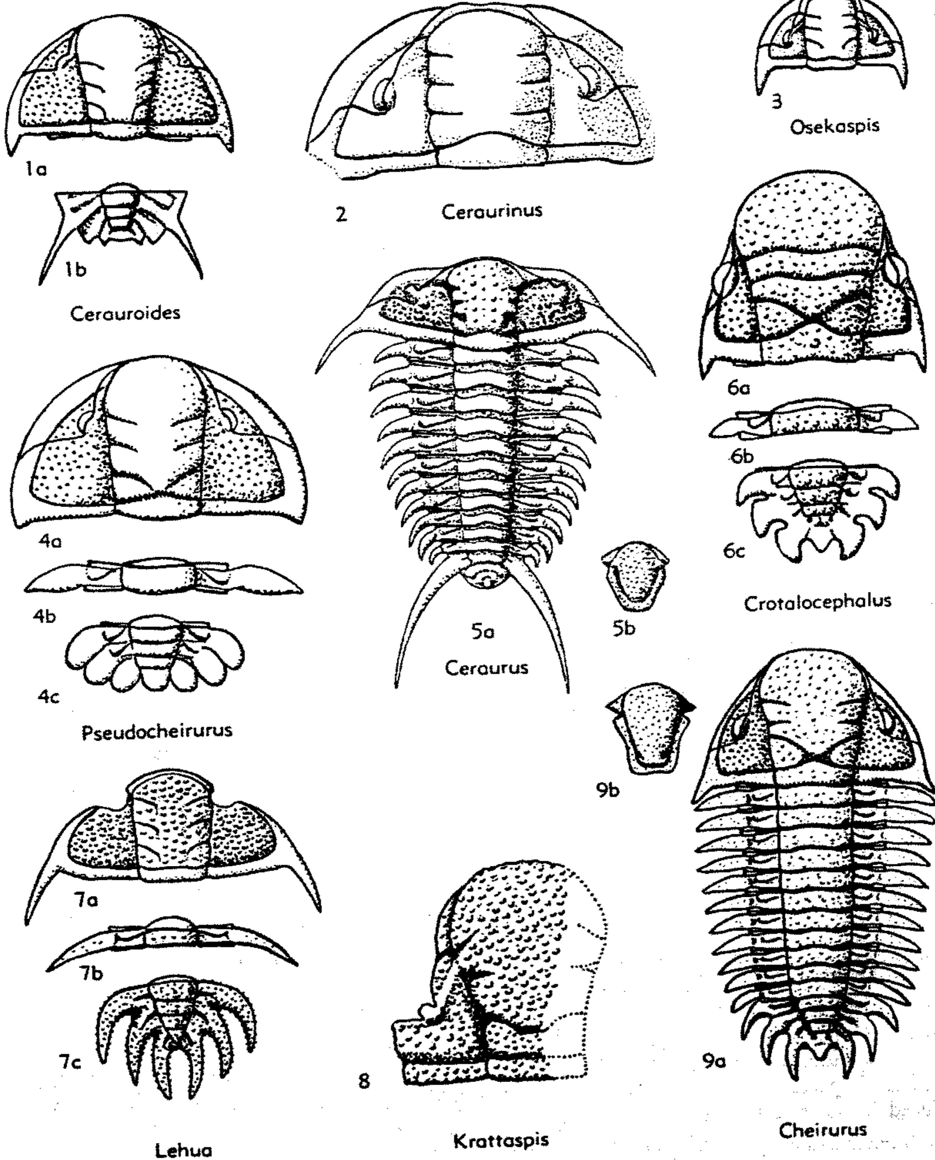
FIG. 335. Cheiruridae (Cheirurinae) (p. 0431-0433).
