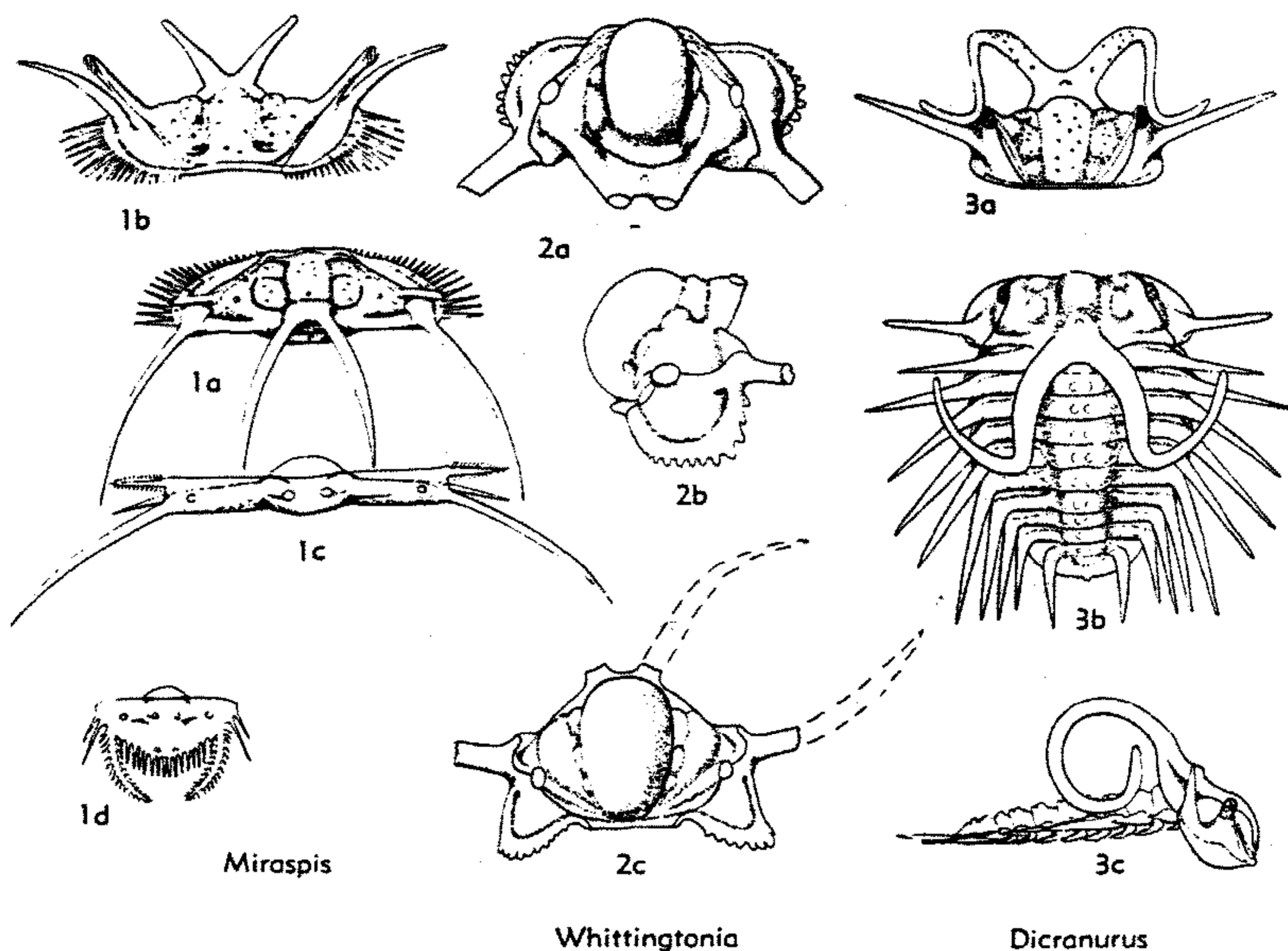
FIG. 399. Odontopleuridae (Miraspidinae) (p. 0506-0508).
