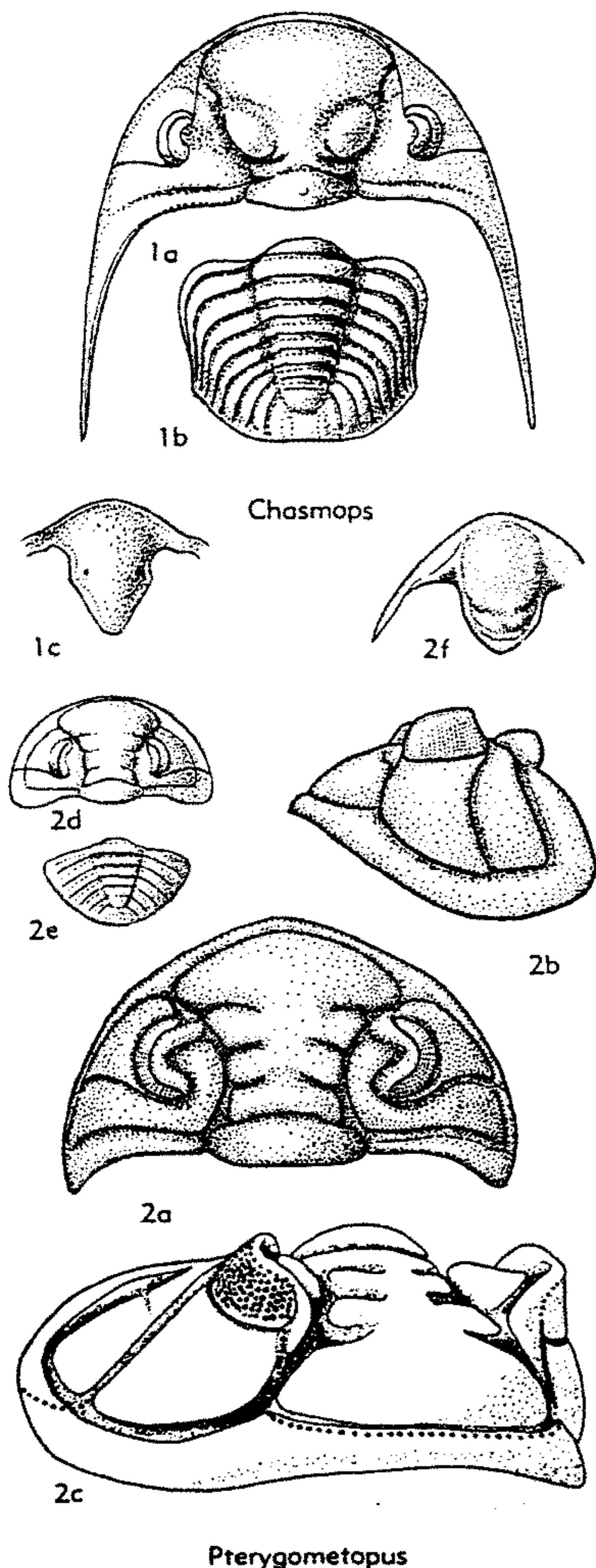
FIG. 388. Pterygometopidae (Pterygometopinae, Chasmopinae) (p. 0490-0493).
