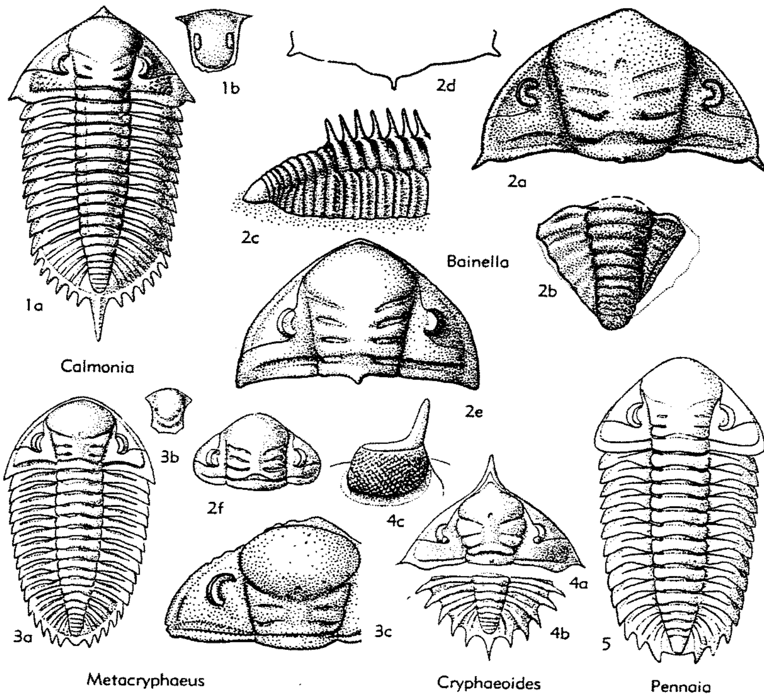
FIG. 383. Calmoniidae (Calmoniinae) (p. 0484-0486).
