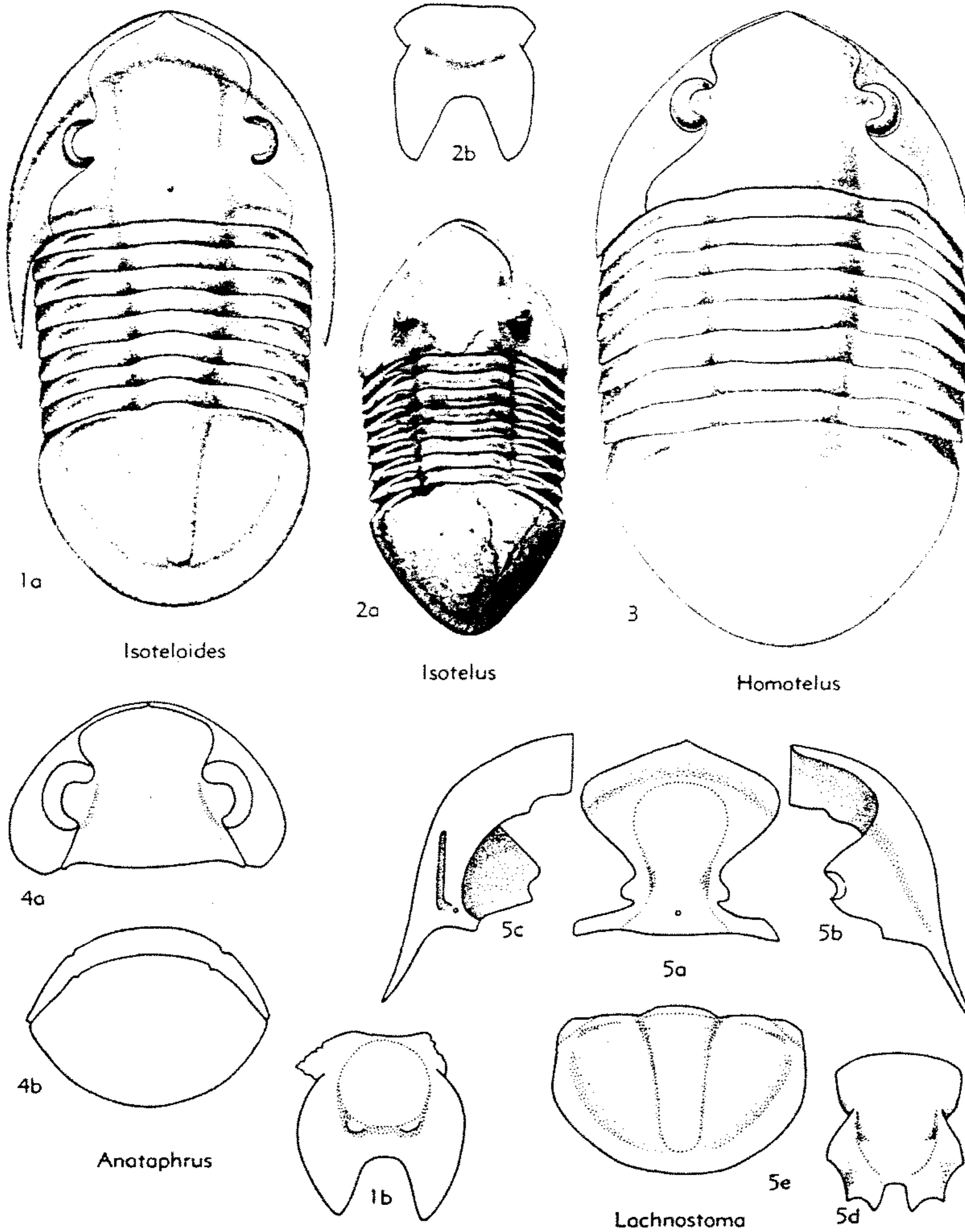
FIG. 251. Asaphidae (Isotelinae) (p. 0339-0340).
