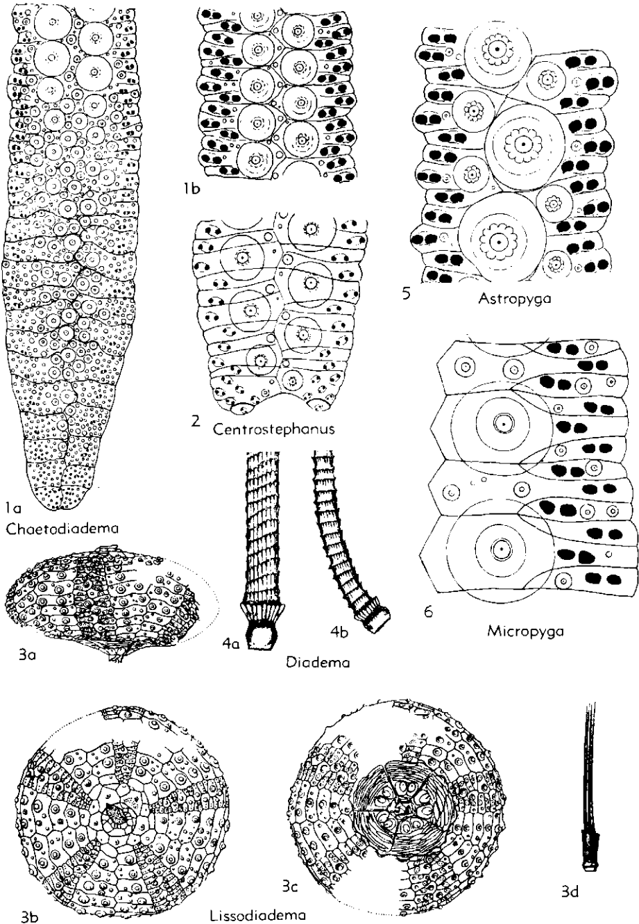
FIG. 259. Diadematacea (1-2,4-5); Lissodiadematacea (3); Micropygidae (6) (p. U350, U352).
