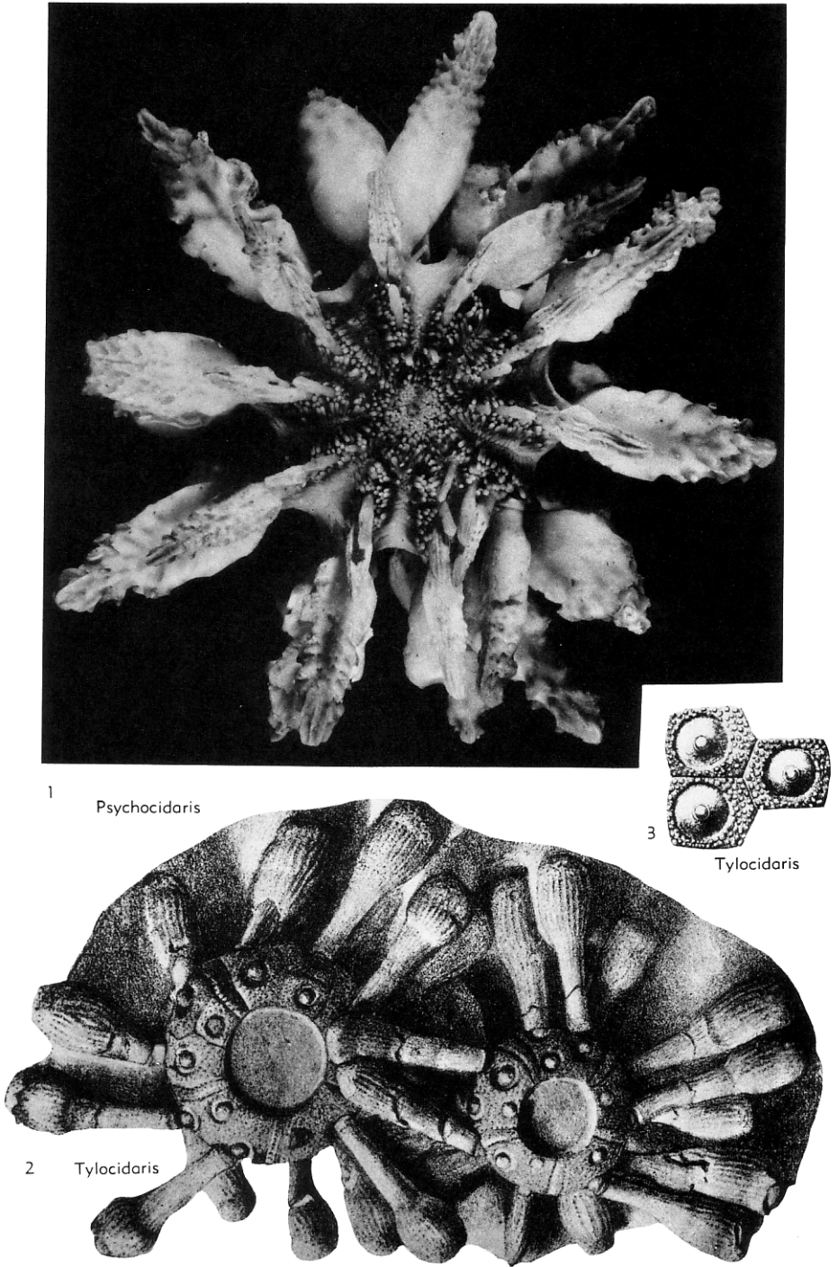
FIG. 252. Psychocidaridae (p. U338-U339).
