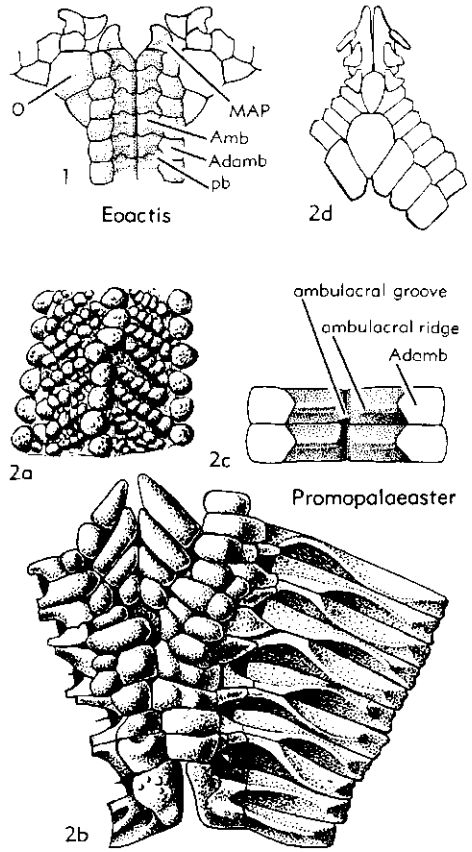
FIG. 50. Promopalaeasteridac (2); Eoactinidac (1). [Explanation: Adamb , adambulacrals; Amb , ambulacrals; MAP , mouth-angle plate; O , odontophore; pb , podial basin.] (p. U53).
