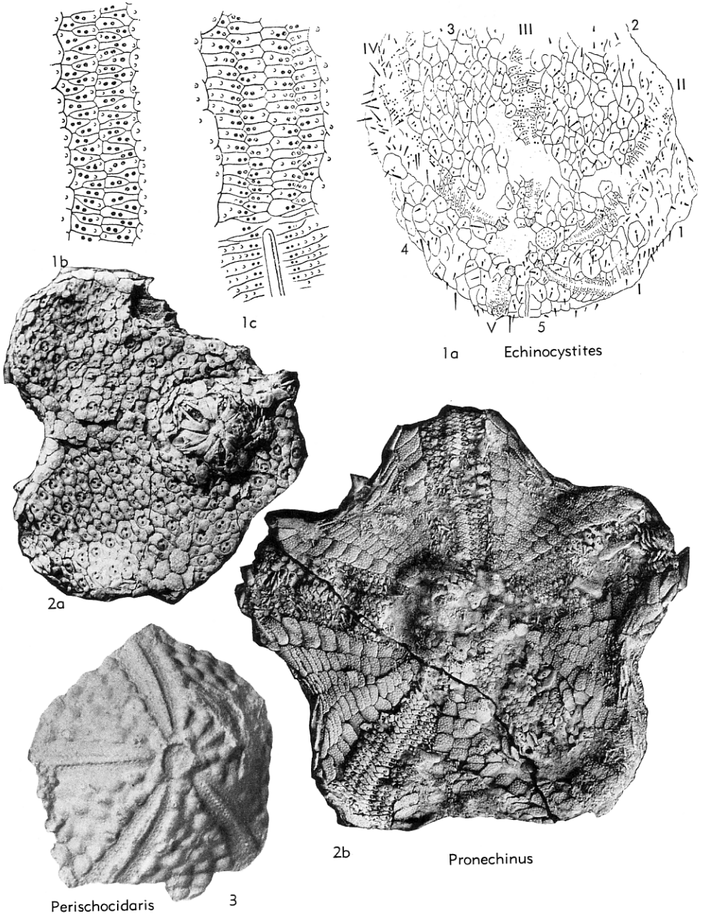
FIG. 223. Echinocystitidae (p. U301).
