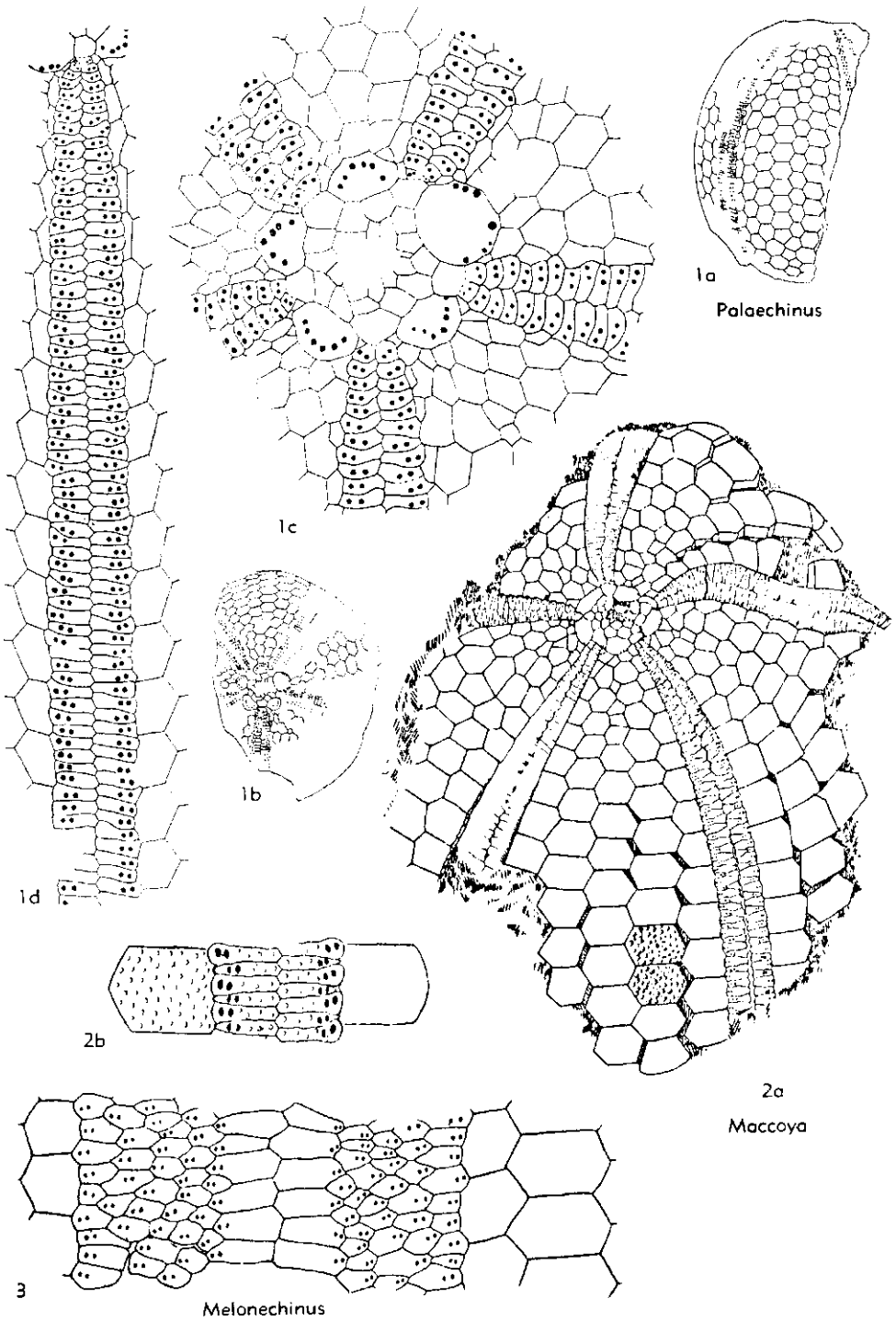
FIG. 231. Palaechinidae (p. U309).
