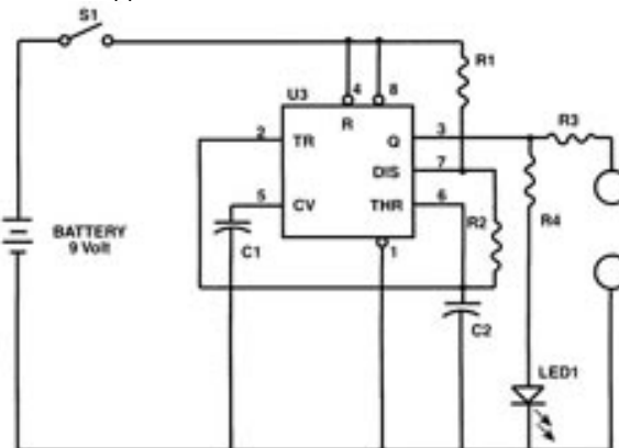
Circuito zapper Dra. Clark
