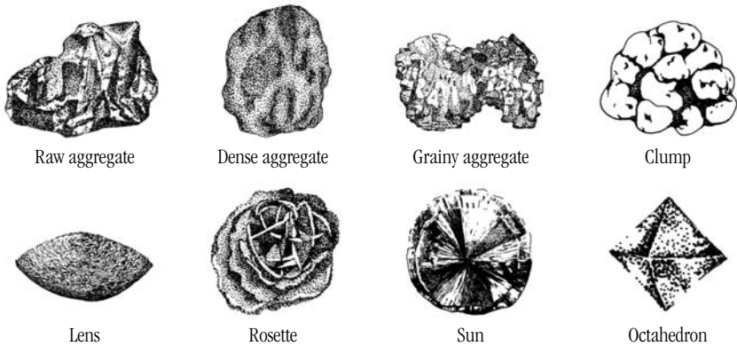
Fig. 22: Crystals
