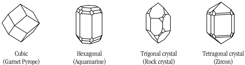
Fig. 22: Crystals
