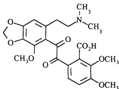
narceinone
