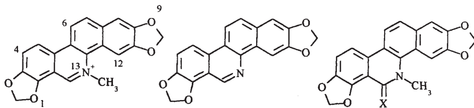
sanguinarine
