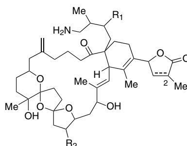
18 R 1 = H, R 2 = CH 3 , Δ 2,3
