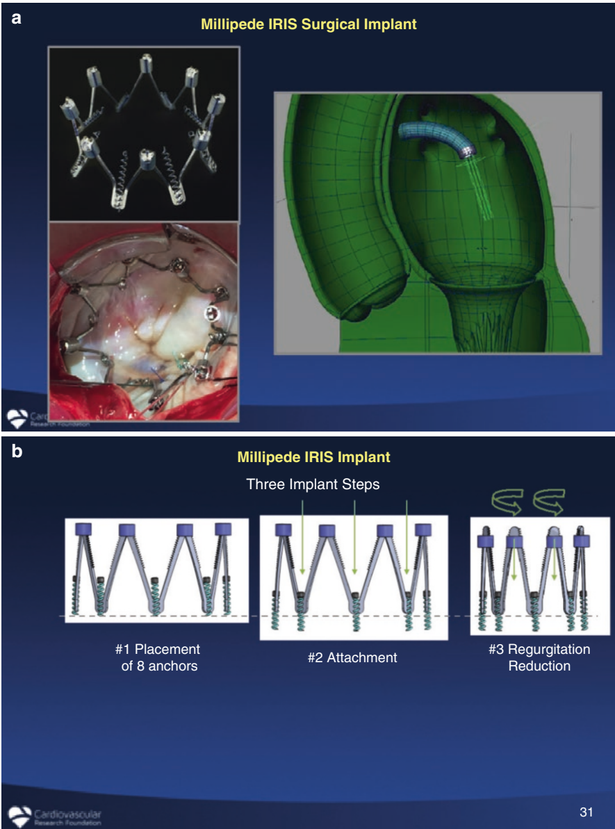
Fig. 15.13 Millipede implant
