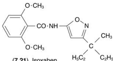
(7.21) Isoxaben
