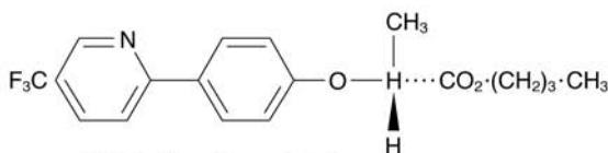
(7.20) Fluzifop-p-butyl
