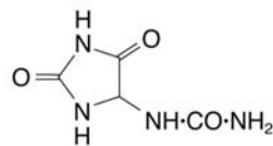
(4.61) Allantoin
