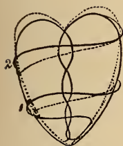
Fig. 148. Thermal or Encasing Atom.
