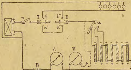
ASSEMBLAGE POUR L'ALIMENTATION DE LAMPES À INCANDESCENCE PAR ACCUMULATEURS Figure spécimen du Manuel de montage des appareils d'Eclairage électrique .
