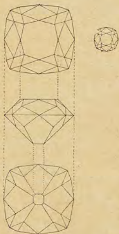
Fig. 37. — Vue en plan (par-dessus et par-dessous) et en élévation d'un diamant taillé en brillant.
