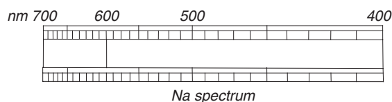
Na spectrum
