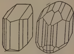
2. Realgar p. 100 (Felsöbanya, Rumania)
