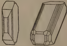
2. Realgar p. 100 (Felsöbanya, Rumania)
