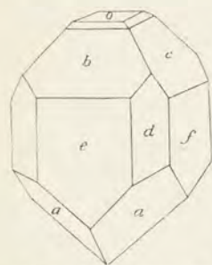
Obr. 71. Různopolární krystal kalamínu. a jehlan, b střečan příčný, c střečan podélný, d hranol, e dvojice stěn příčných, f dvojice stěn podélných, o plocha spodová.
