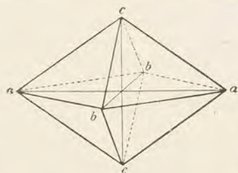
Obr. 17. Jehlanec kosočtverečný. Osy aa , bb , cc jsou nestejně délky. Příčný, podélný i vodorovný řez dávají kosočtverce.
