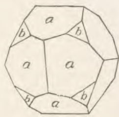
Obr. 26. Spojka 12stěnu pětiúhelníkového a s osmistěnem b.
