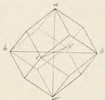
Obr. 6. Dvanáctistěn kosočtverečný, do něhož jsou vrýsovány osy aa' , bb' , cc' .
