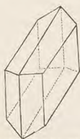
Obr. 56. Krystal sody.
