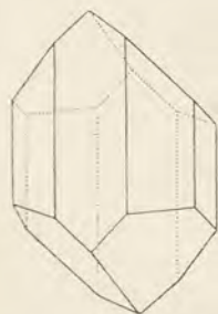
Obr. 72. Krystal augitu.
