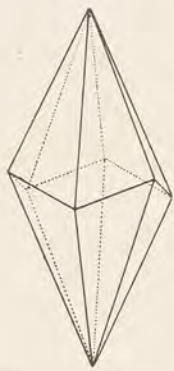
Obr. 31. Jehlanec klencový.
