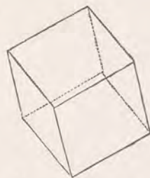
Obr. 22. Klenec.
