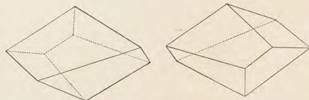
Obr. 37. Klencový lichostěň.
