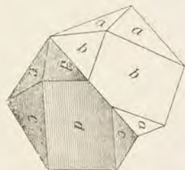
Obr. 42. Srostlice dvou krystalů cínovce. a jehlanec jednoho, c jehlanec druhého krystalu, b hranol jednoho, d hranol druhého krystalu.
