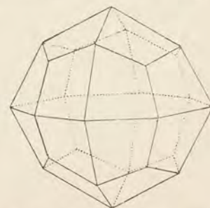
Obr. 8. Čtyřiadvacetistěn deltooidový.
