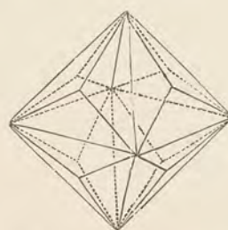
Obr. 7. Čtyřiadvacetistěn trojúhelníkový.
