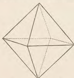
Obr. 5. Osmistěn.
