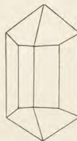
Obr. 67. Krystal topasový.
