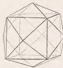
Obr. 48. Čtyřiadvacetistěn krychlový.
