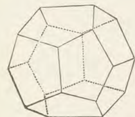
Obr. 25. Dvanáctistěn pětiúhelníkový.
