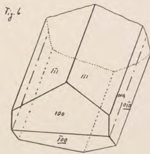
Fig. 1 & 2 Columbit. Fig. 3 Mossit. Fig. 4—6 Ilmenorutil. Fig. 7 Euxenit.
