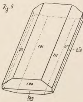
Fig. 1 & 2 Columbit. Fig. 3 Mossit. Fig. 4—6 Ilmenorutil. Fig. 7 Euxenit.
