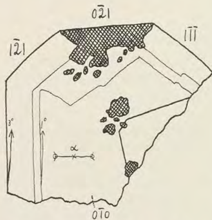
Fig. 3. Thalenit von Hundholmen; Schnitt parallel 010 . Orthis ist dunkel schraffiert.
