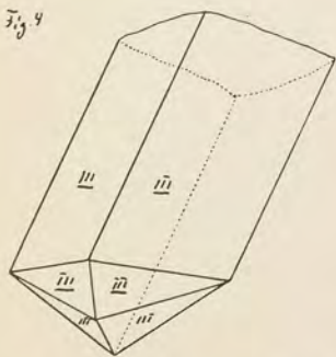
Fig. 1 & 2 Columbit. Fig. 3 Mossit. Fig. 4—6 Ilmenorutil. Fig. 7 Euxenit.
