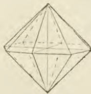
Fig. 54. Ditoeder.
