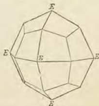
Fig. 9. Kristalltetraeder. Anatim.
