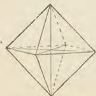
Fig. 7. Oktaeder. Magnetkies.
