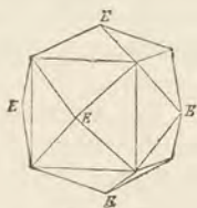
Fig. 12. Pyramidenwürfel. Flußspat.
