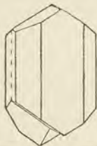
Fig. 124. Augit. Zwilling.
