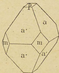
Fig. 3. — Cristal octaédrique.
