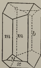
Fig. 292.
