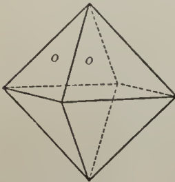
Fig. 213. Octahedron.
