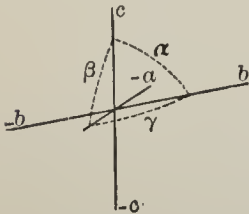
Fig. 183. Triclinic Axes.
