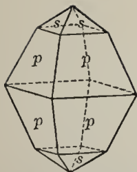
Fig. 154. Sulphur.
