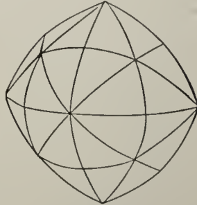
Fig. 207.
