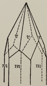
Fig. 137. Calcite.
