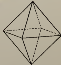
Fig. 19. Octahedron.
