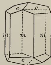
Fig. 277.
