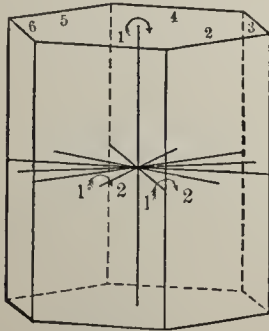
Fig. 106.
