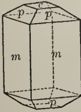
Fig. 92. Vesuvianite.
