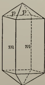
Fig. 89. Zircon.
