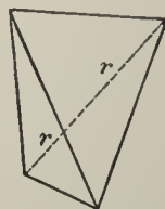
Fig. 228.
