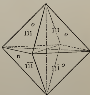
Fig. 32. Octahedron.
