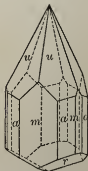
Fig. 143. Tourmaline.
