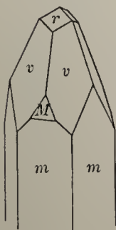
Fig. 138. Calcite.
