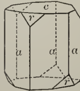
Fig. 132. Corundum.
