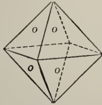
Fig. 14. Octahedron.
