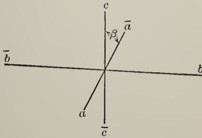
Fig. 166. Monoclinic Axes.
