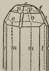
Fig. 159. Topaz.
