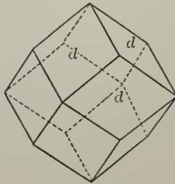
Fig. 214. Dodecahedron.
