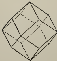
Fig. 21. Dodecahedron.
