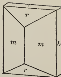
Fig. 156. Staurolite.
