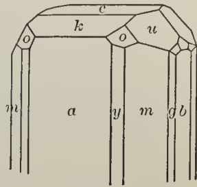
Fig. 347.
