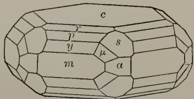
Fig. 118. Apatite.
