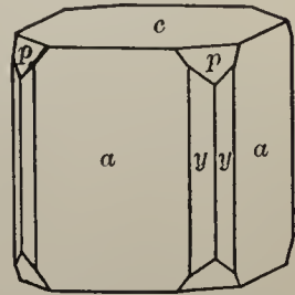
Fig. 97. Apophyllite.
