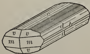
Fig. 223.
