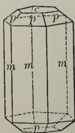
Fig. 349.
