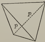
Fig. 101. Sphenoid.
