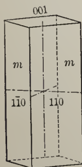
Fig. 82.
