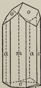
Fig. 140. Tourmaline.
