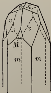
Fig. 139. Calcite.
