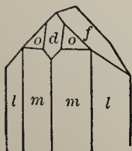
Fig. 157. Topaz.
