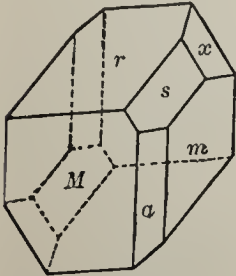
Fig. 189. Axinite.
