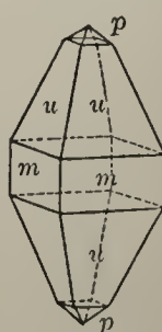
Fig. 90. Zircon.
