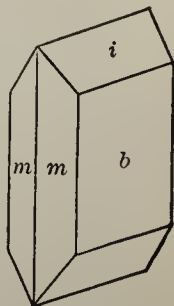
Fig. 290.
