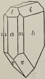
Fig. 165. Calamine.
