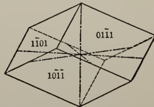
Fig. 124. Negative Rhombohedron.
