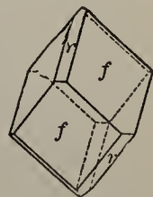
Fig. 127. Calcite.
