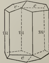
Fig. 130. Calcite.
