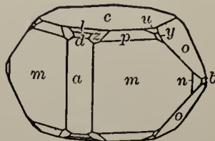
Fig. 161. Anglesite.
