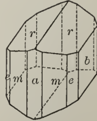
Fig. 178.
