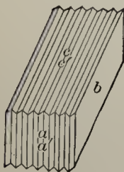
Fig. 300.
