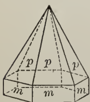
Fig. 119. Zincite.
