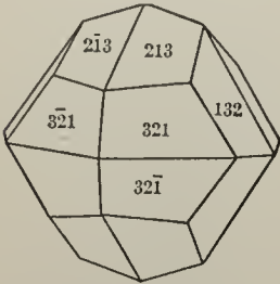
Fig. 57. Diploid.
