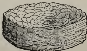
Fig. 260.
