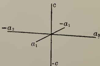
Fig. 79. Tetragonal Axes.
