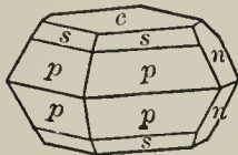
Fig. 155. Sulphur.
