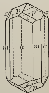
Fig. 103. Scapolite.
