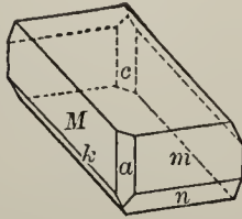
Fig. 190. Rhodonite.
