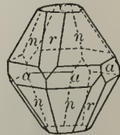
Fig. 133. Corundum.
