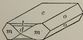
Fig. 356.
