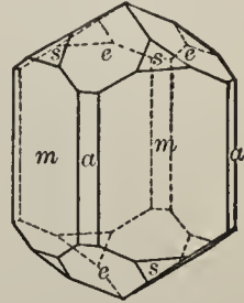
Fig. 94. Rutile.
