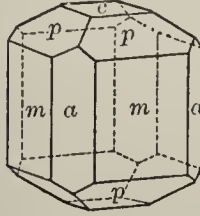
Fig. 93. Vesuvianite.
