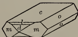
Fig. 164. Celestite.
