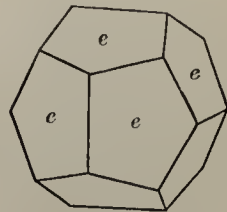
Fig. 230. Pyritohedron.
