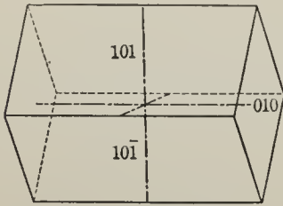
Fig. 151.
