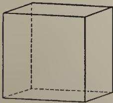
Fig. 17. Cube.
