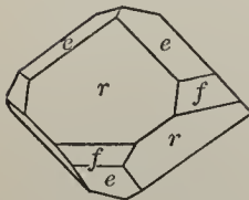
Fig. 131. Chabazite.
