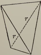
Fig. 100. Sphenoid.
