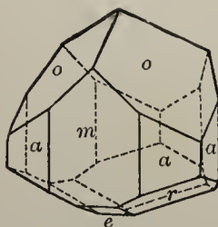
Fig. 142. Tourmaline.
