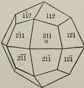
Fig. 42. Trapezohedron.
