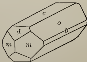
Fig. 357.
