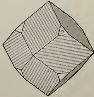
Fig. 266.
