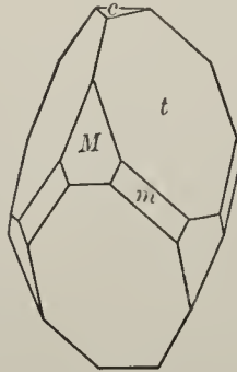
Fig. 129. Calcite.
