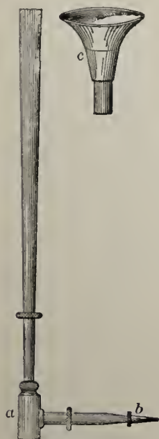
Fig. 200
