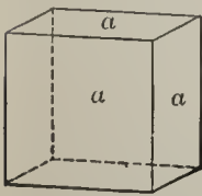
Fig. 13. Cube.
