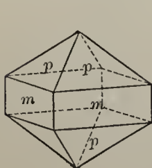
Fig. 88. Zircon.
