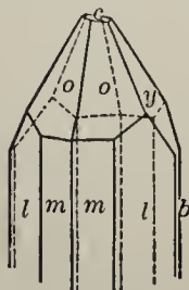
Fig. 158. Topaz.
