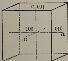
Fig. 31. Cube.
