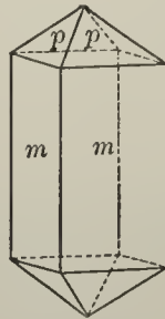
Fig. 321.
