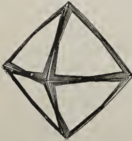
Fig. 206.
