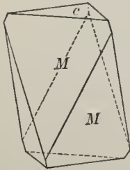
Fig. 128. Calcite.
