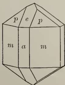
Fig. 267.
