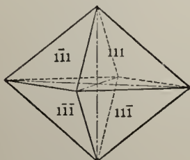
Fig. 149. Pyramid.
