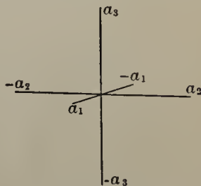
Fig. 25. Isometric Axes.
