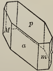
Fig. 191. Chalcantite.
