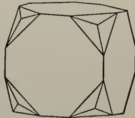
Fig. 344.
