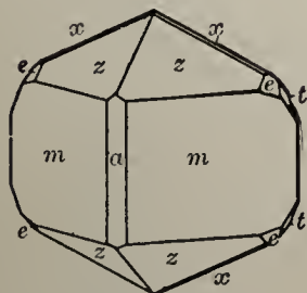
Fig. 160. Brookite.
