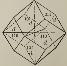
Fig. 35. Dodecahedron.
