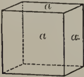
Fig. 220. Cube.
