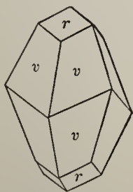
Fig. 136. Calcite.
