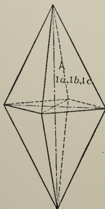
Fig. 9. Orthorhombic Pyramid.
