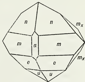
Fig. 550. Datolite.
