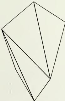
Fig. 225. Tetragonal Scalenohedron.
