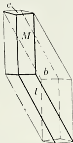
Fig. 520. Gypsum.
