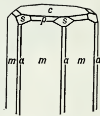
Fig. 565. Epidote.
