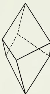
Fig. 35. Trigonal Trapezohedron.
