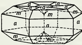
Fig. 305. Rutile.
