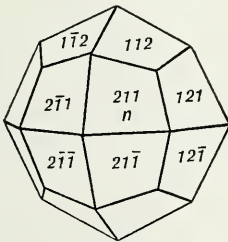
Fig. 86. Trapezohedron.
