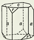
Fig. 174. Corundum.
