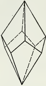
Fig. 219. Tetragonal Trapezohedron.
