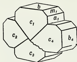
Fig. 436. Bournonite.
