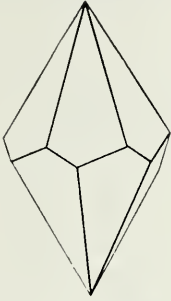
Fig. 37. Hexagonal Trapezohedron.
