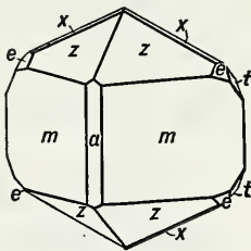
Fig. 254. Brookite.
