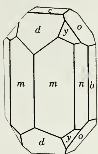
Fig. 59. Anglesite.
