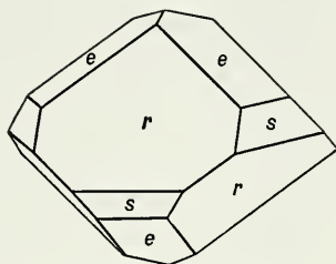
Fig. 632. Chabazite.
