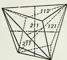
Fig. 107. Tristetrahedron.
