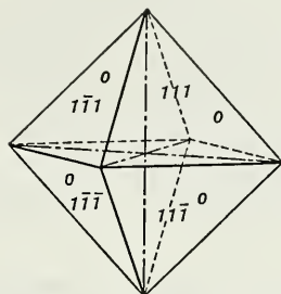
Fig. 76. Octahedron.
