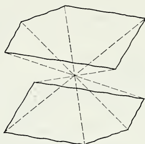
Fig. 292. Pinacoid.
