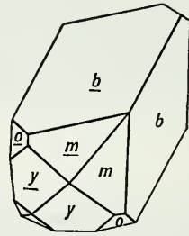
Fig. 620. Baveno Twin.
