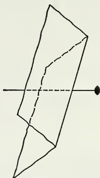
Fig. 286. Sphenoid.
