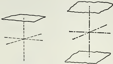
Fig. 18. Pedion. Fig. 19. Pinacoid.
