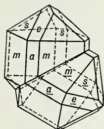
Fig. 319. Cassiterite.
