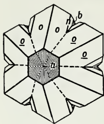
Fig. 461. Chrysoberyl.
