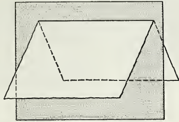
Fig. 20. Dome.
