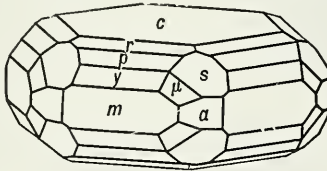
Fig. 155. Apatite.
