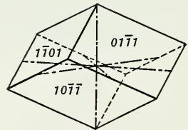
Fig. 166. Negative Rhombohedron.
