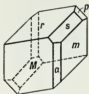
Fig. 563. Axinite.
