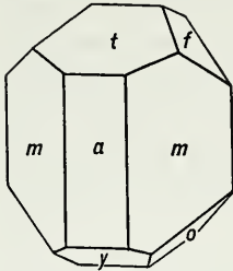
Fig. 527. Wolframite.
