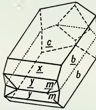
Fig. 619. Manebach Twin.
