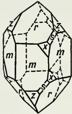
Fig. 185. Right-Hand Quartz.
