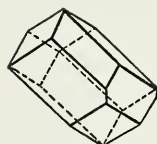
Fig. 51. Malformed Dodecahedron.
