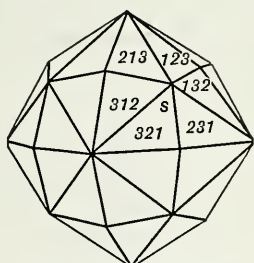
Fig. 92. Hexoctahedron.
