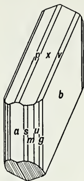
Fig. 418. Orpiment.
