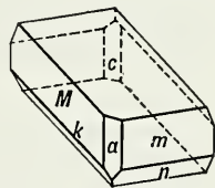
Fig. 578. Rhodonite.
