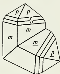
Fig. 320. Rutile.
