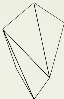
Fig. 33. Tetragonal Scalenohedron.
