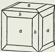
Fig. 392. Copper Crystal.
