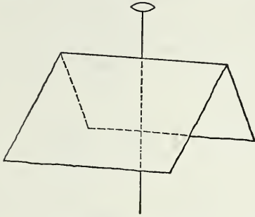
Fig. 21. Sphenoid.
