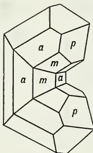
Fig. 320. Rutile.
