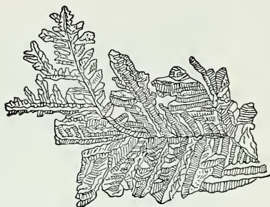
Fig. 391. Dendritic Gold.
