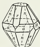
Fig. 175. Corundum.
