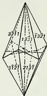
Fig. 178. Negative Scalenohedron.
