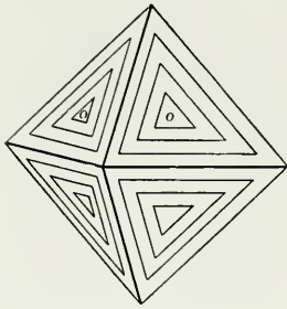
Fig. 457. Gahnite.
