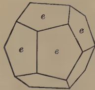
Fig. 230. Pyritohedron.
