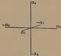
Fig. 25. Isometric Axes.
