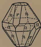
Fig. 135. Corundum.
