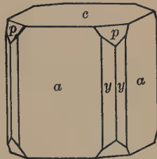
Fig. 97. Apophyllite.
