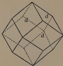
Fig. 214. Dodecahedron.
