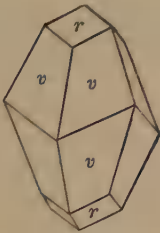
Fig. 136. Calcite.
