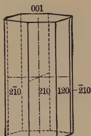
Fig. 84. Ditetragonal Prism.
