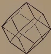
Fig. 21. Dodecahedron.
