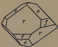
Fig. 131. Chabazite.
