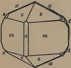
Fig. 160. Brookite.
