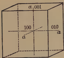
Fig. 31. Cube.
