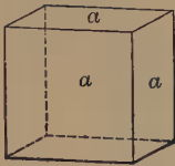
Fig. 13. Cube.
