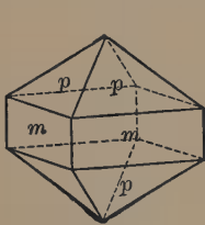
Fig. 88. Zircon.
