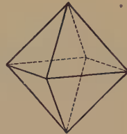
Fig. 19. Octahedron.
