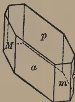
Fig. 191. Chalcantite.
