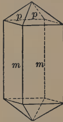
Fig. 89. Zircon.
