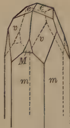
Fig. 139. Calcite.
