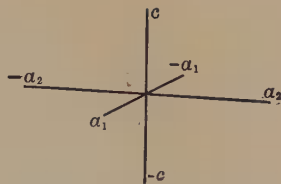
Fig. 79. Tetragonal Axes.
