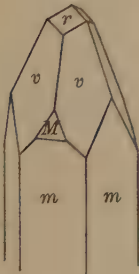
Fig. 138. Calcite.
