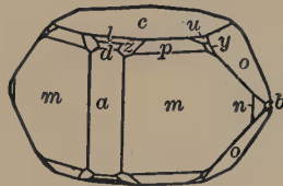
Fig. 161. Anglesite.
