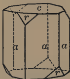
Fig. 132. Corundum.
