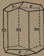
Fig. 130. Calcite.
