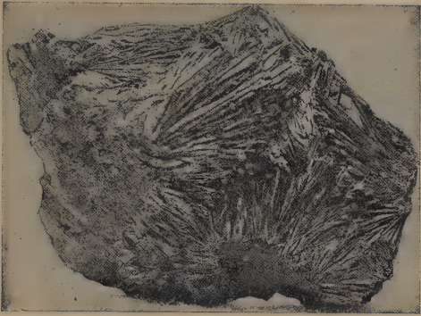
A. Pyrolusite, Negaunee, Michigan.
