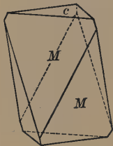
Fig. 128. Calcite.
