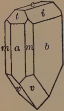
Fig. 165. Calamine.
