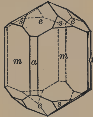
Fig. 94. Rutile.
