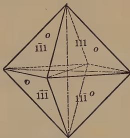
Fig. 32. Octahedron.
