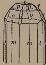
Fig. 159. Topaz.
