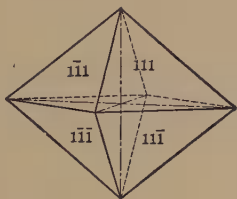
Fig. 149. Pyramid.
