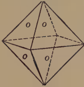
Fig. 14. Octahedron.
