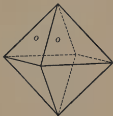
Fig. 213. Octahedron.
