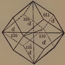
Fig. 35. Dodecahedron.
