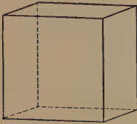
Fig. 17. Cube.
