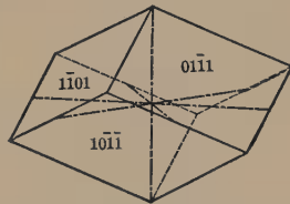
Fig. 124. Negative Rhombohedron.
