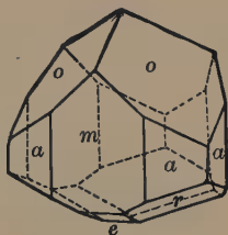
Fig. 142. Tourmaline.
