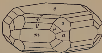
Fig. 118. Apatite.
