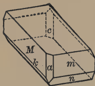
Fig. 190. Rhodonite.
