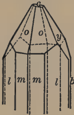
Fig. 158. Topaz.
