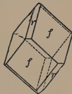
Fig. 127. Calcite.
