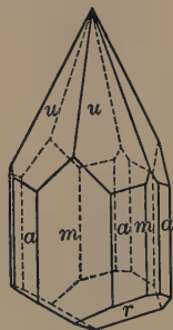
Fig. 143. Tourmaline.
