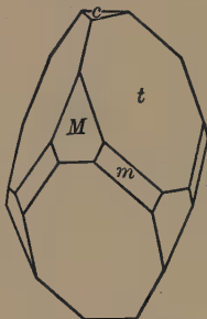
Fig. 129. Calcite.
