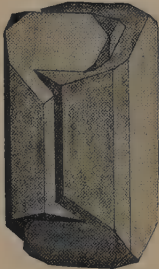
Fig. 294. Carlsbad Twin.
