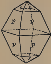
Fig. 154. Sulphur.
