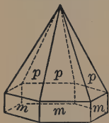
Fig. 119. Zincite.
