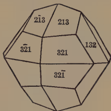
Fig. 57. Diploid.
