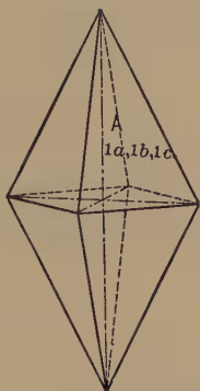
Fig. 9. Orthorhombic Pyramid.
