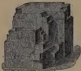
Fig. 192. Cubic Cleavage — Galena.
