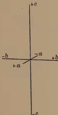
Fig. 8. Orthorhombic Crystal Axes.
