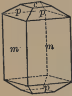
Fig. 92. Vesuvianite.
