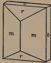
Fig. 156. Staurolite.
