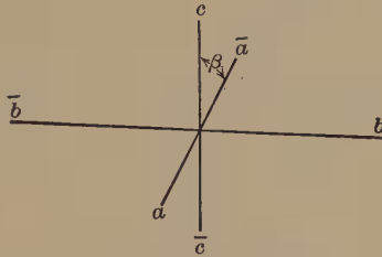
Fig. 166. Monoclinic Axes.
