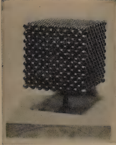
A. Cube.
