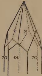
Fig. 137. Calcite.
