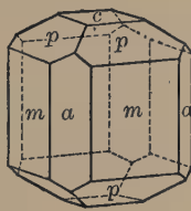
Fig. 93. Vesuvianite.
