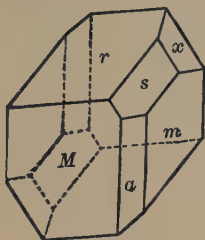
Fig. 189. Axinite.
