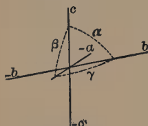
Fig. 183. Triclinic Axes.
