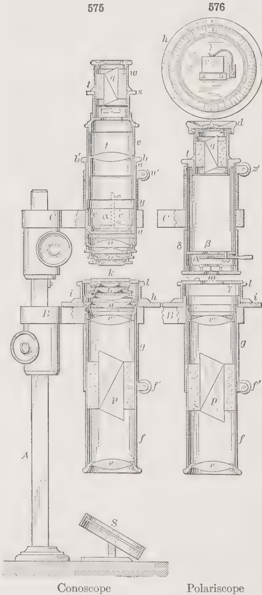
Conoscope
