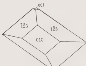
Figs. 941, 942, Chondrodite , Brewster, N. Y.
