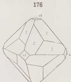
Cuprite
