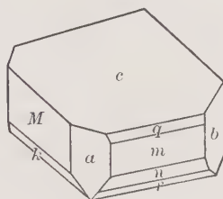
Rhodonite
