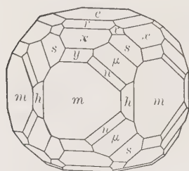
Apatite
