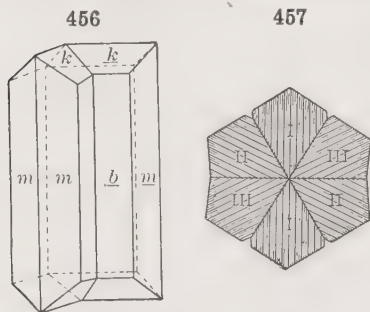
Aragonite
