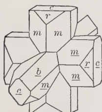
Staurolite
