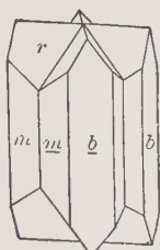
Staurolite
