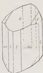
Nagy-Ág
