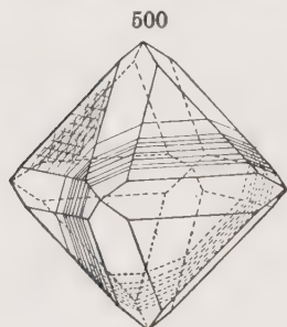
Magnetite
