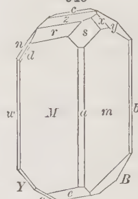
Bethlehem, Pa.
