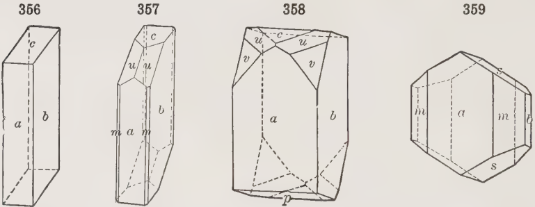
Pyroxene
