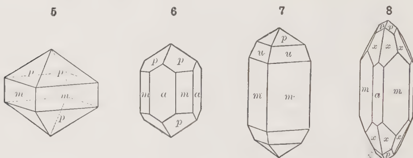
Zircon
