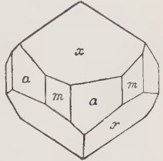
Mt. Antero, Col., Pfd.
