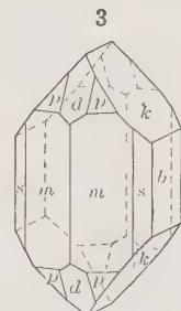
Chrysolite
