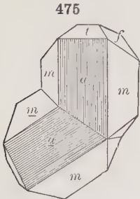
Wolframite
