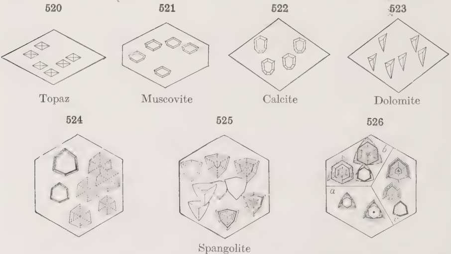
Spangolite
