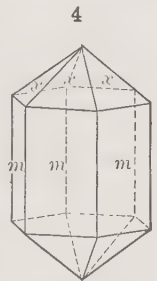
Apatite
