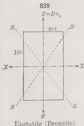
Enstatite (Bronzite)
