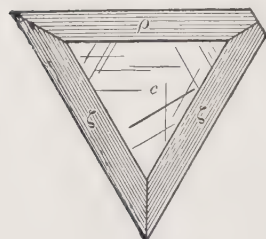
Biotite
