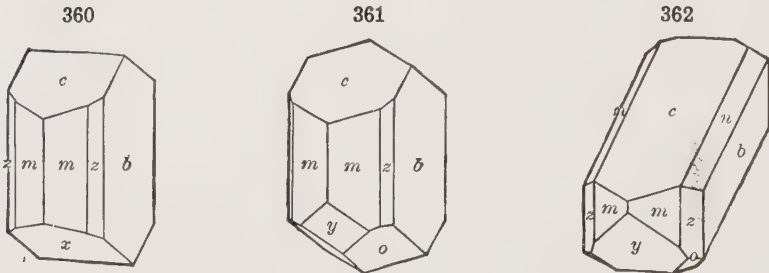
Orthoclase
