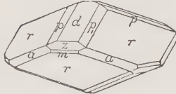
Florissant, Col.
