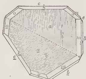
Columbite
