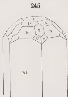
Beryl
