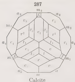
Calcite
