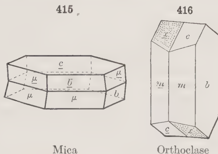
Mica
