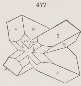
Pyroxene
