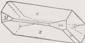
Pericline
