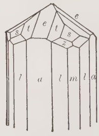
Rutile
