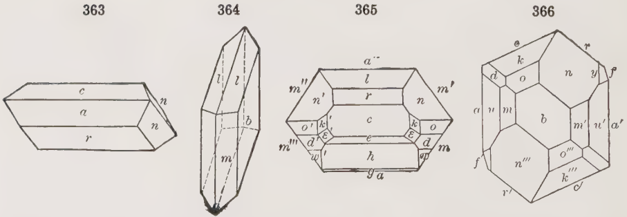
Epidote
