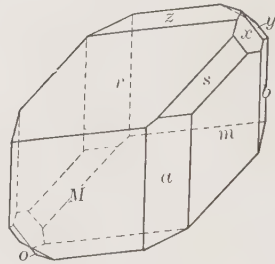
Axinite
