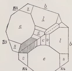
Marcasite
