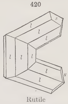
Rutile
