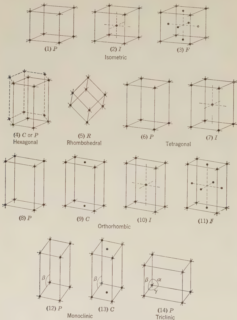
Fig. 1. 14 Bravais Space Lattices.
