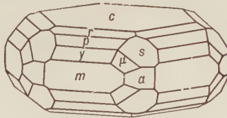
Fig. 155. Apatite.
