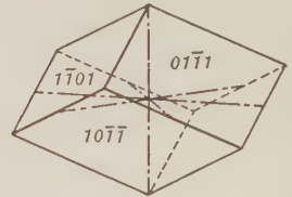
Fig. 166. Negative Rhombohedron.
