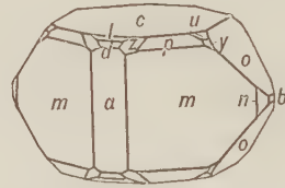
Fig. 255. Anglesite.
