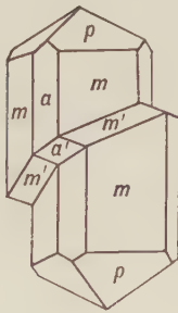
Fig. 320. Rutile.
