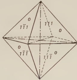
Fig. 76. Octahedron.
