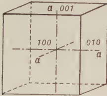
Fig. 75. Cube.
