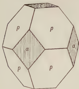
Fig. 16. Apophyllite.
