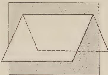
Fig. 20. Dome.
