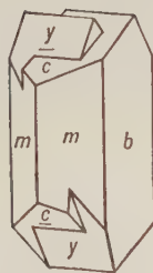
Fig. 618. Carlsbad Twin.
