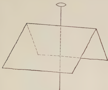
Fig. 21. Sphenoid.
