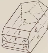
Fig. 330. Manebach Twin.
