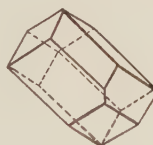
Fig. 51. Malformed Dodecahedron.
