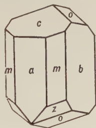
Fig. 510. Borax.
