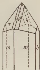
Fig. 419. Stibnite.
