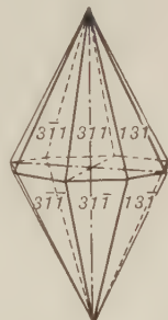
Fig. 208. Ditetragonal Dipyramid.
