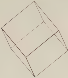
Fig. 193. Rhombohedron.
