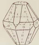
Fig. 175. Corundum.
