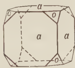
Fig. 470. Sylvite.
