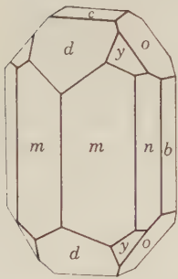
Fig. 59. Anglesite.
