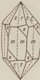
Fig. 317. Dauphiné Twin.
