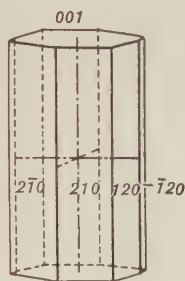
Fig. 205. Ditetragonal Prism.
