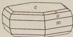
Fig. 416. Pyrrhotite.
