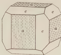
Fig. 17. Pyrite.
