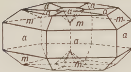
Fig. 305. Rutile.
