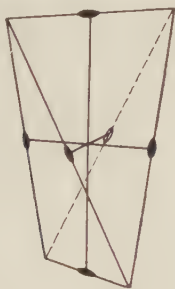
Fig. 223. Symmetry Axes.
