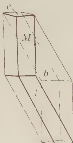
Fig. 520. Gypsum.
