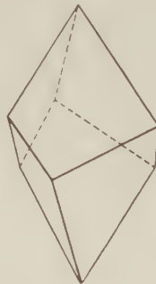
Fig. 35. Trigonal Trapezohedron.
