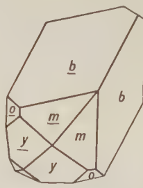
Fig. 620. Baveno Twin.
