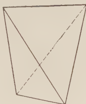
Fig. 22. Disphenoid.
