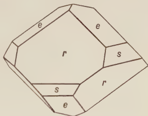
Fig. 632. Chabazite.
