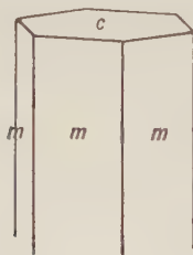
Fig. 564. Beryl.
