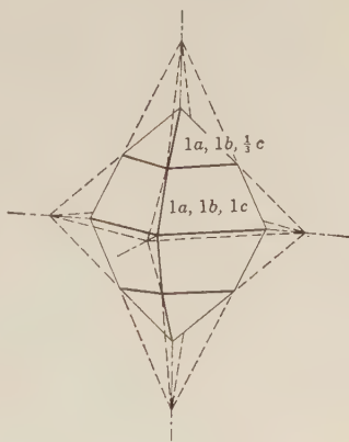
Fig. 13. Sulfur.
