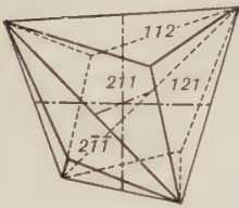
Fig. 107. Tristetrahedron.
