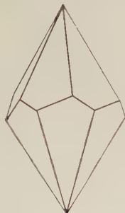
Fig. 146. Hexagonal Trapezohedron.
