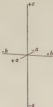
Fig. 238. Orthorhombic Crystal Axes.
