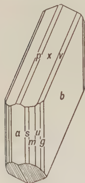
Fig. 418. Orpiment.
