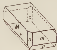
Fig. 578. Rhodonite.
