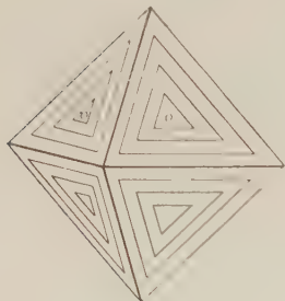
Fig. 457. Gahnite.
