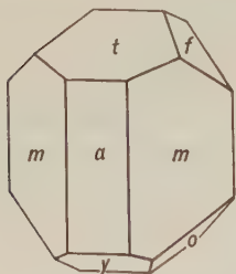
Fig. 527. Wolframite.
