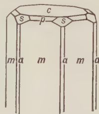
Fig. 565. Epidote.
