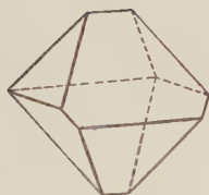
Fig. 49. Malformed Octahedron.
