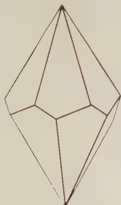
Fig. 37. Hexagonal Trapezohedron.
