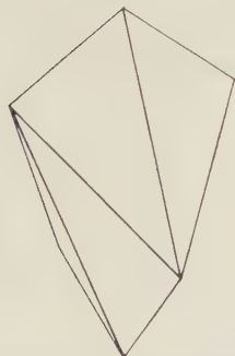
Fig. 225. Tetragonal Scalenohedron.
