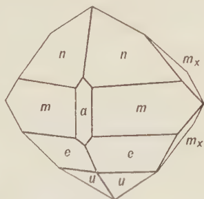
Fig. 550. Datolite.
