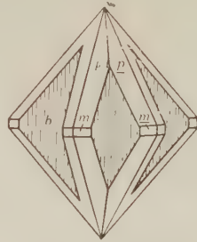
Fig. 325. Cerussite.
