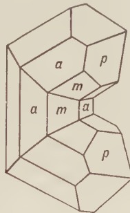
Fig. 321. Rutile.
