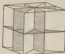
Fig. 200. Symmetry Planes.
