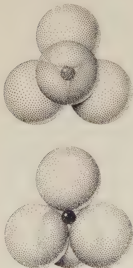
Fig. 531. \text{SiO}_4 Tetrahedra.
