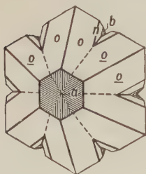
Fig. 461. Chrysoberyl.
