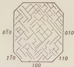
Fig. 574. Pyroxene Cleavage.
