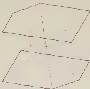
Fig. 292. Pinacoid.
