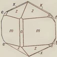
Fig. 254. Brookite.
