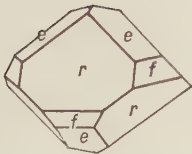
Fig. 173. Chabazite.
