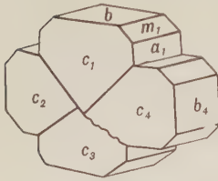
Fig. 436. Bournonite.
