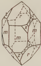
Fig. 185. Right-Hand Quartz.
