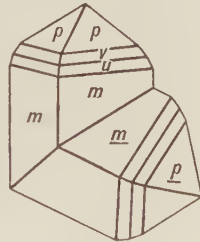
Fig. 322. Zircon.
