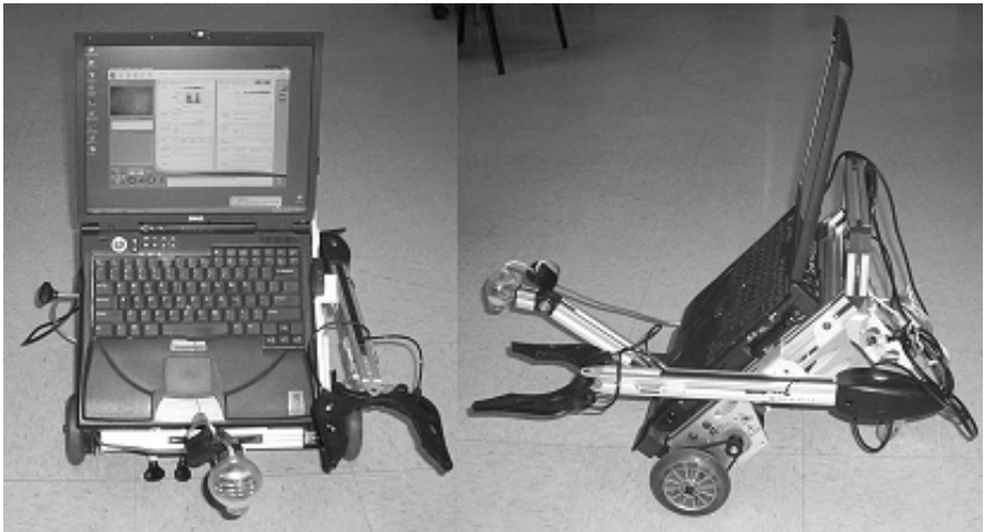
Fig. 2. ER1 robot
