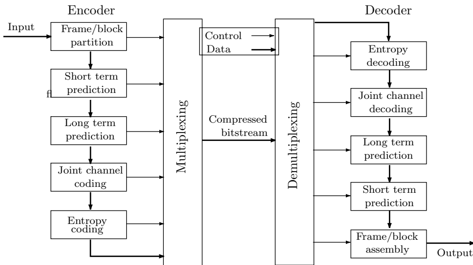
Figure 7.38: Organization of the ALS Encoder and Decoder.
