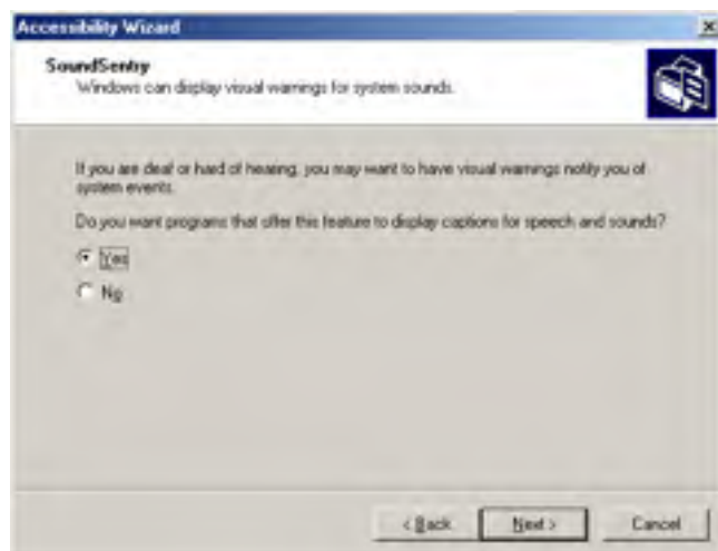
Fig. 24.28 SoundSentry dialog.
