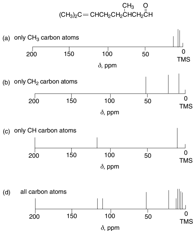
Fig. 10-24. 13 C NMR spectra of citronella.
