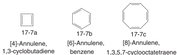
Fig. 17-7. Annulenes.
