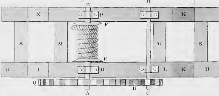
Fig. 2. Plan
