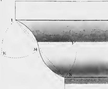
Fig. 7. Cyma Recta
