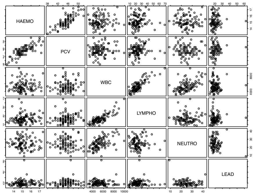
Fig. 59 Draughtsman’s plot.
