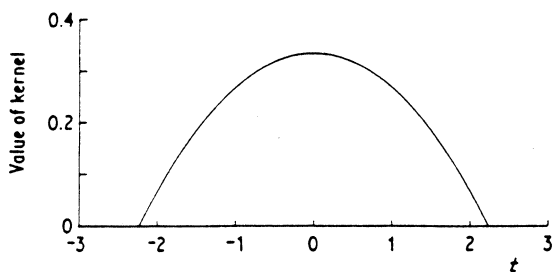
Fig. 79 Epanechnikov kernel.
