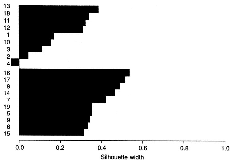
Fig. 121 Silhouette plot.
