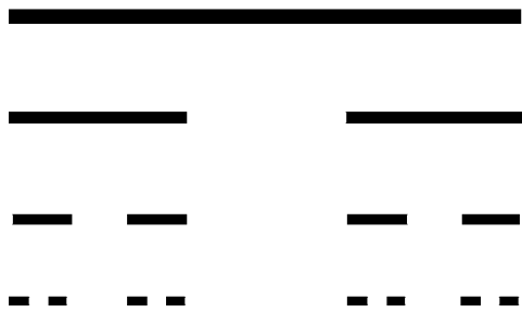
Cantor dust.
