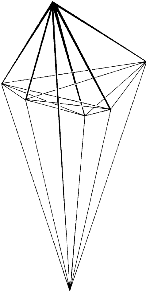
Császár polyhedron
