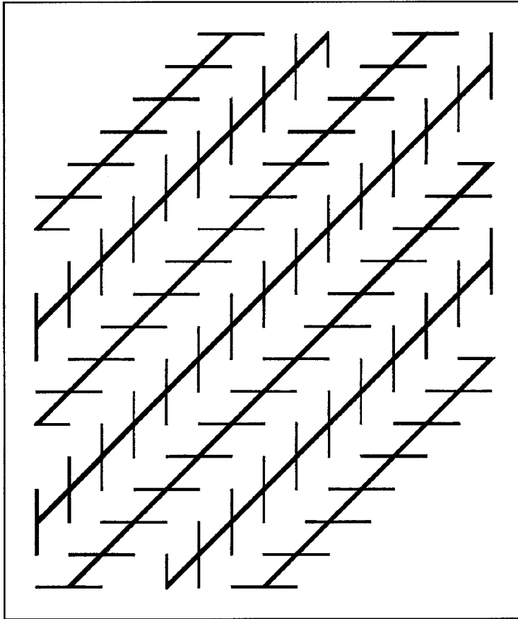
Zöllner illusion
