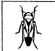
N. nigropictus
