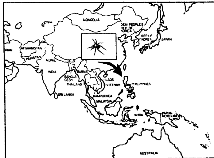
Predator
