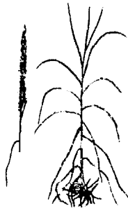
Pennisetum
