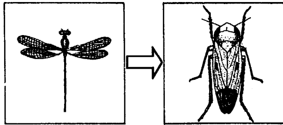
Predator
