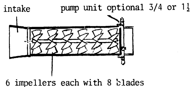
fig. 61: Nel Plata pumping unit.
