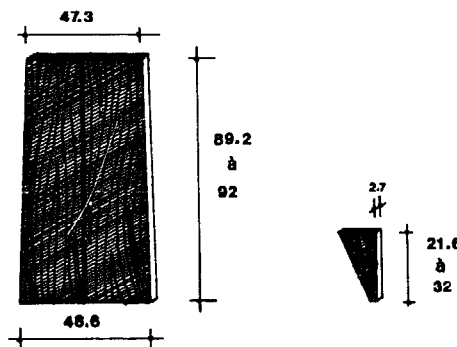
FIGURE 12 : FOND DE BANCHE ET COIN
