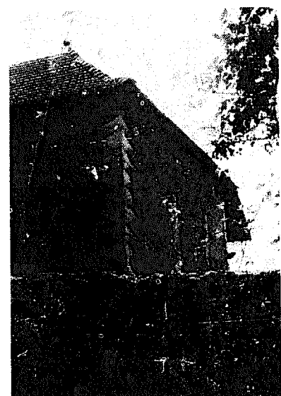
FIGURE 30 : RENFORCEMENT DE L'ANGLE EN « DRAPEAUX » (ISERE)
