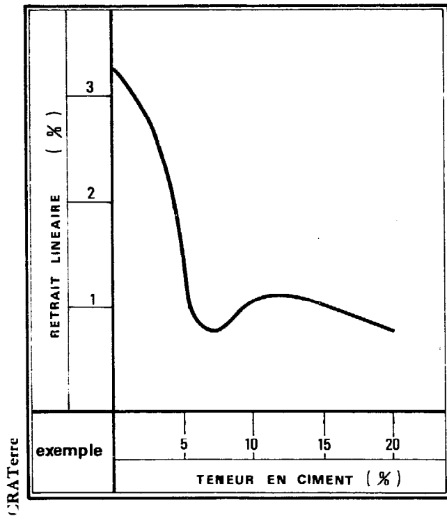
FIGURE 286 : VARIATION DU RETRAIT AVEC LA TENEUR EN CIMENT
