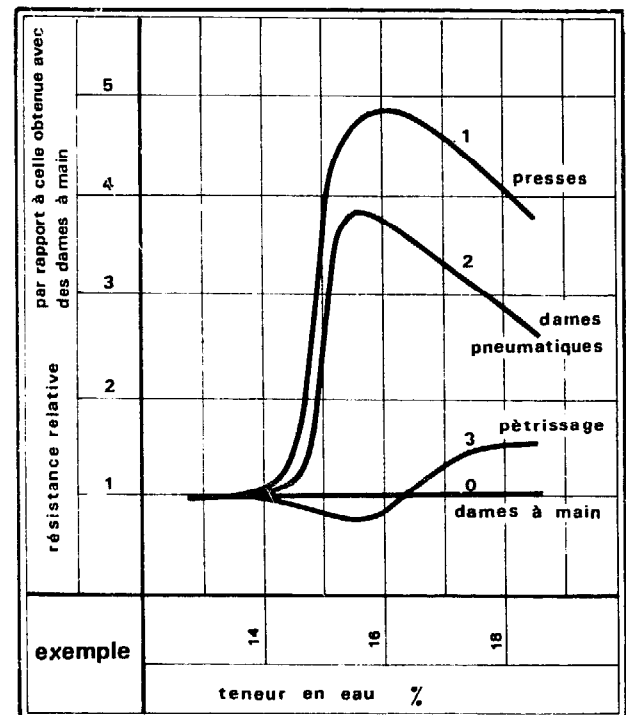
FIGURE 278 : RESISTANCES POUR UNE DEFORMATION DE L'ECHANTILLON DE 5%
