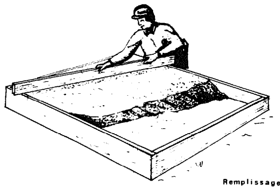
FIGURE 176 : ADOBE DECOUPEE
