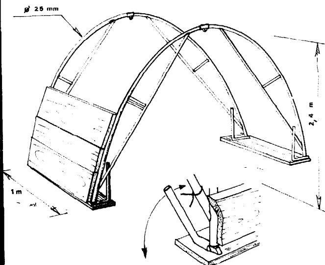
FIGURE 306 : COFFRAGE EXPERIMENTAL AVEC CAME FACILITANT LE DECOFFRAGE
