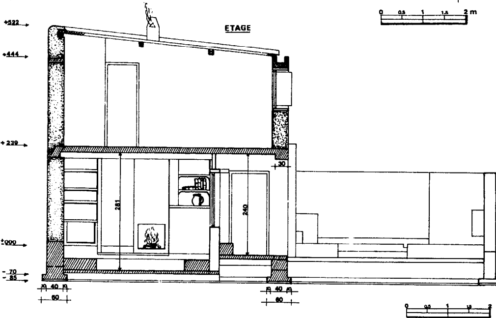
FIGURE 112 : COUPE TRANSVERSALE
