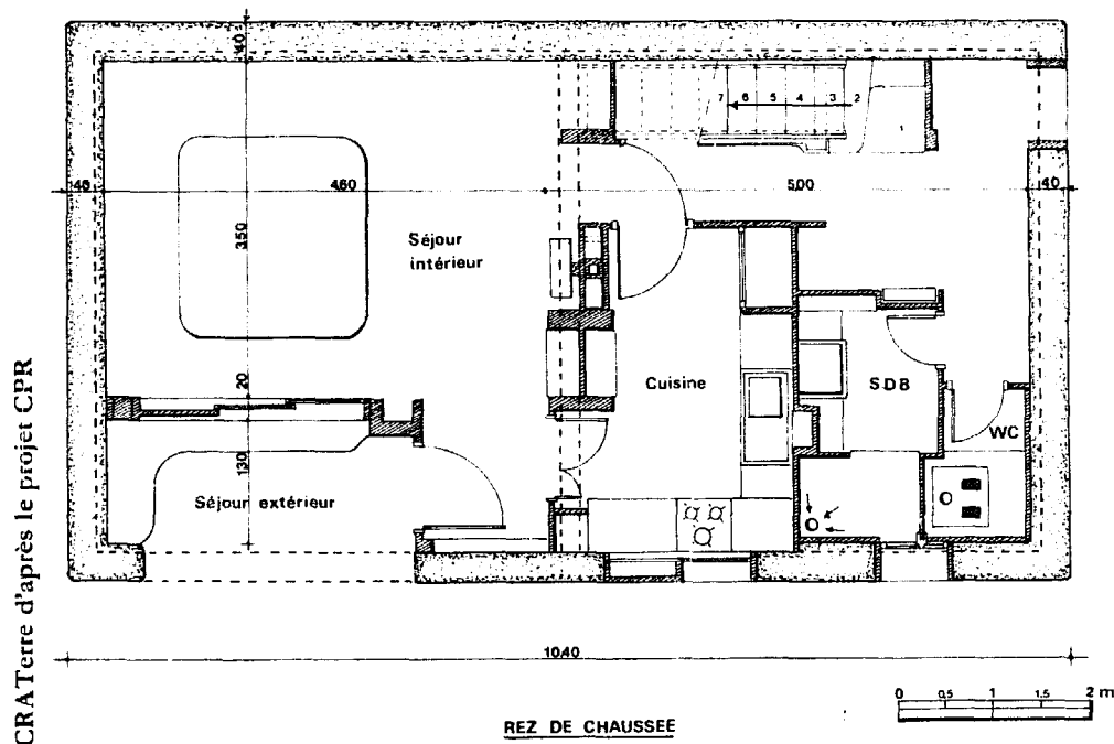
FIGURE 110 : REZ-DE-CHAUSSEE
