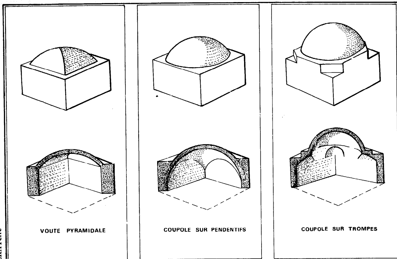
FIGURE 315 : TROIS METHODES POUR POSER UNE COUPOLE SUR UNE PIECE CARREE
