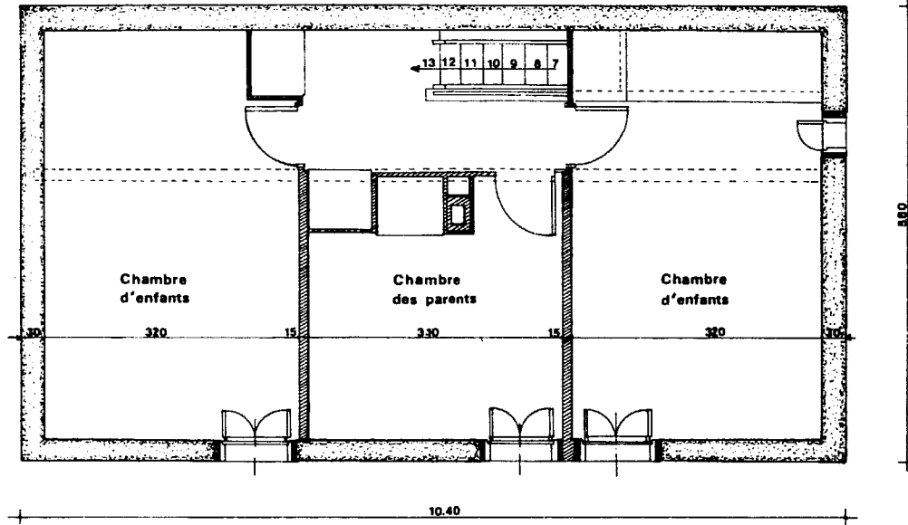
FIGURE 111 : ETAGE
