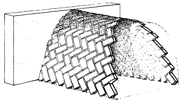
FIGURE 307 : APPAREILLAGE EN EPIS (OU EN CHEVIRON)
